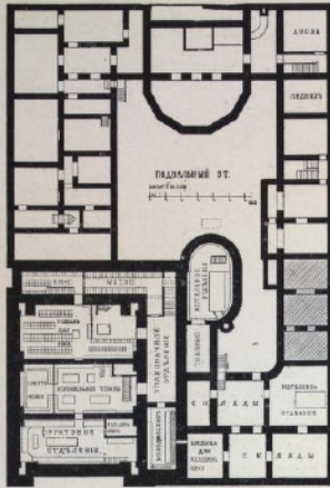
План подвального этажа. Plan du soubassement.
