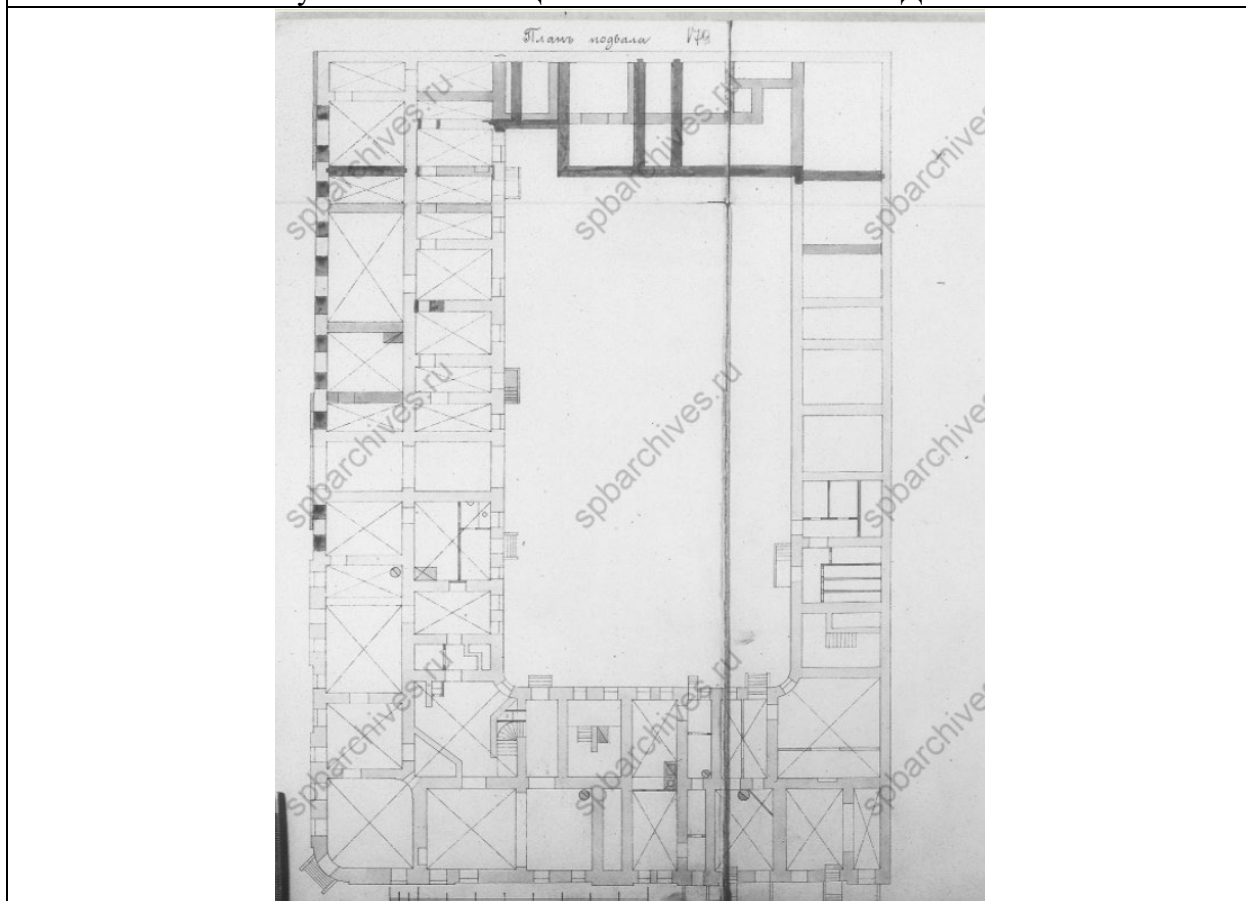
15. План подвала. 1900 г. ЦГИА СПб. Ф.513. Оп.102. Д.9815.Л.178-179.
