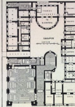
План 1-го этажа. Plan du rez-de-chaussée.
