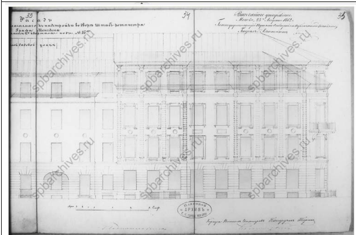
9. Фасад здания по Малой Садовой улице. 1862 г. ЦГИА СПб. Ф.513. Оп.102. Д.9815. Л.34-35.
