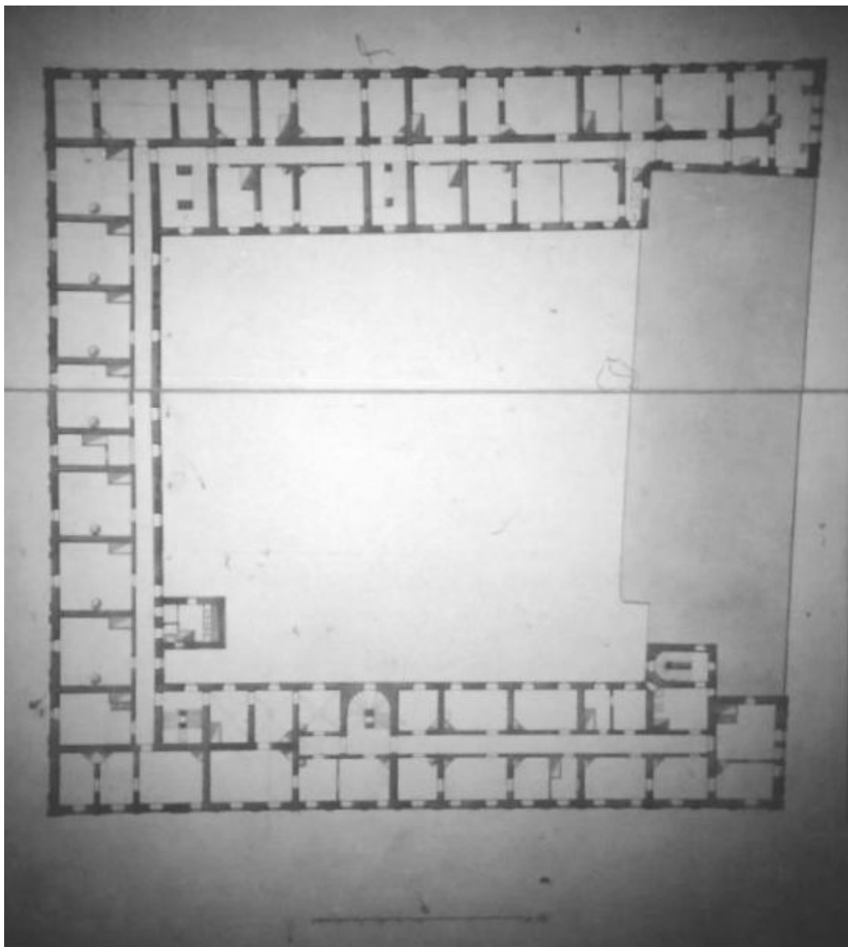
Илл. 11. План верхнего этажа Служебного дома при Мраморном дворце. 1844 г. Архитектор А.П. Брюллов. РГИА. Ф. 485. Оп. 2. Д. 65. Л. 6.
