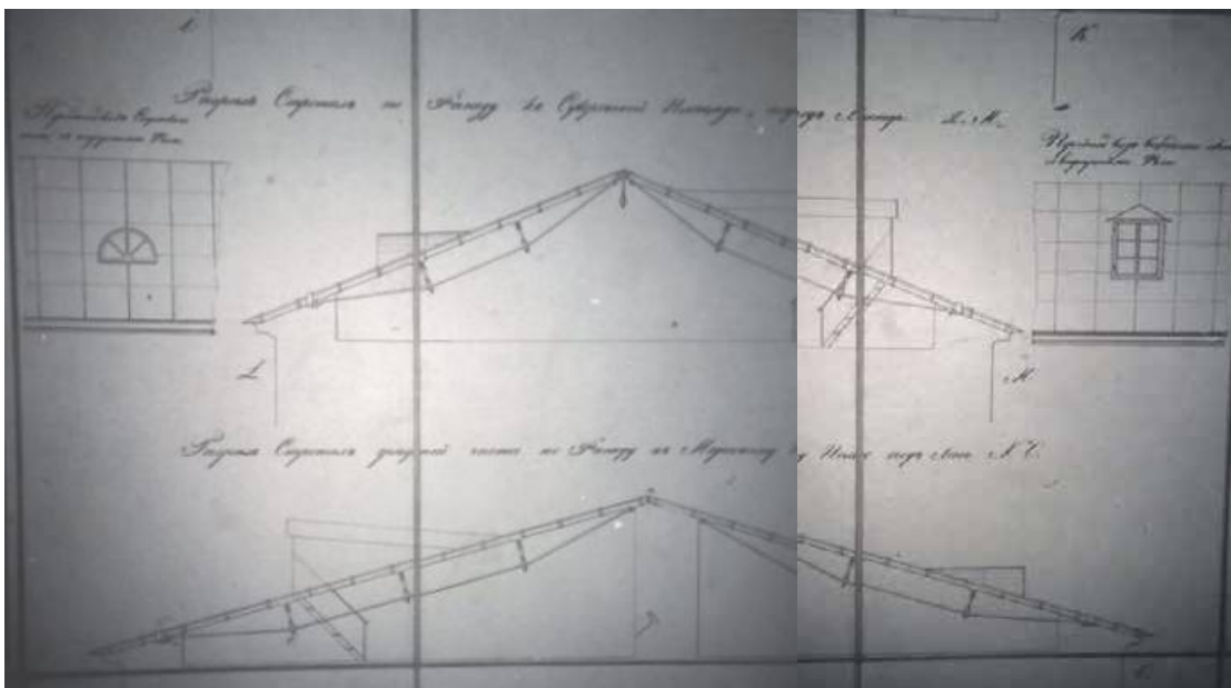
Илл. 12. Разрез стропил по фасаду к Суворовской площади и к Марсову полю. 1844 г.
