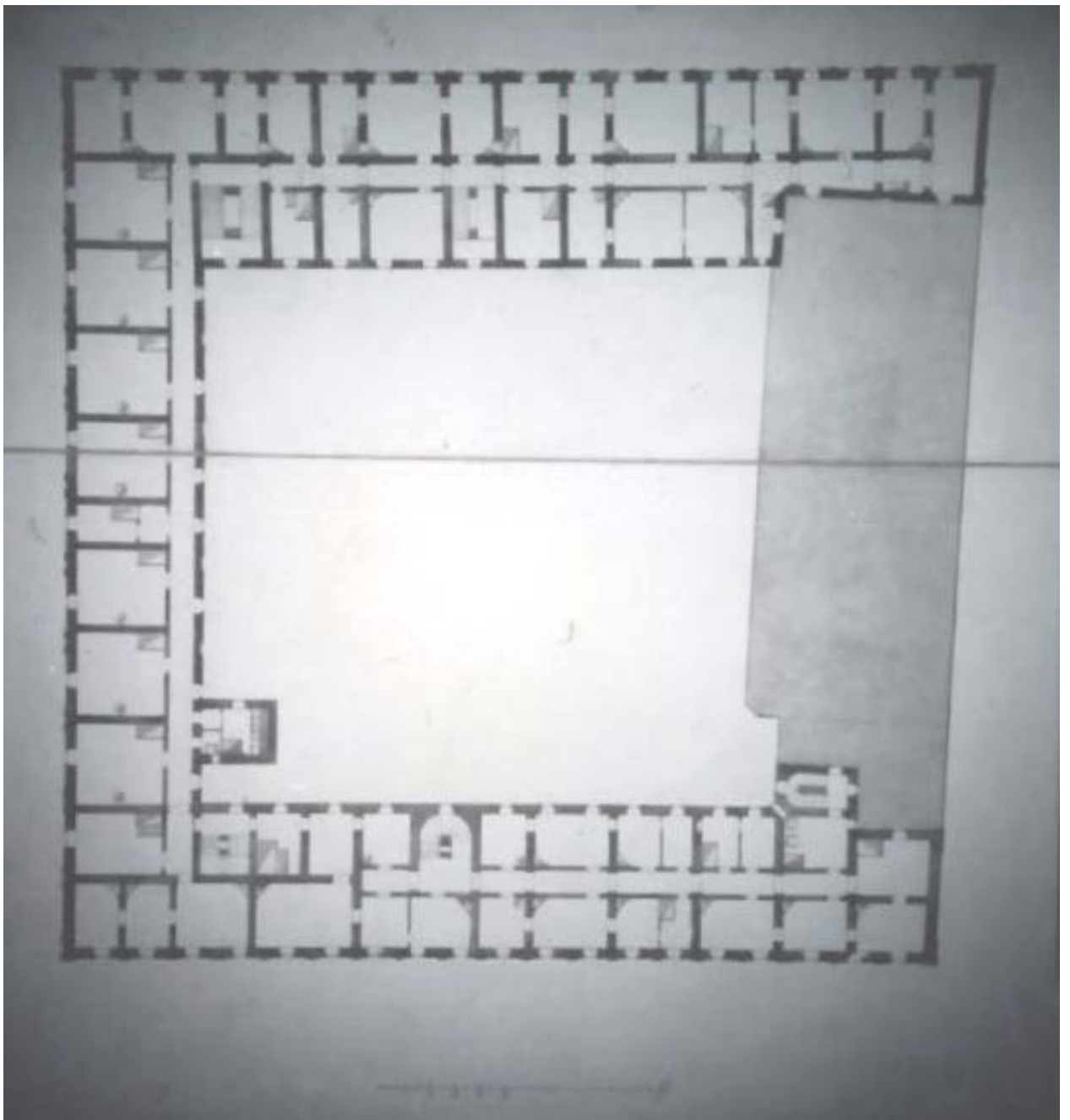
Илл. 10. План среднего этажа Служебного дома при Мраморном дворце. 1844 г. Архитектор А.П. Брюллов. РГИА. Ф. 485. Оп. 2. Д. 65. Л. 5.
