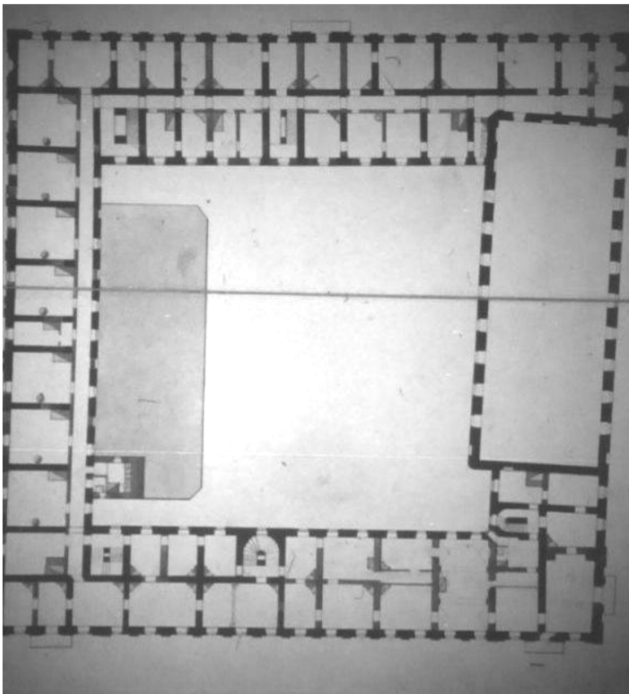
Илл. 9. План второго этажа Служебного дома при Мраморном дворце. 1844 г.
