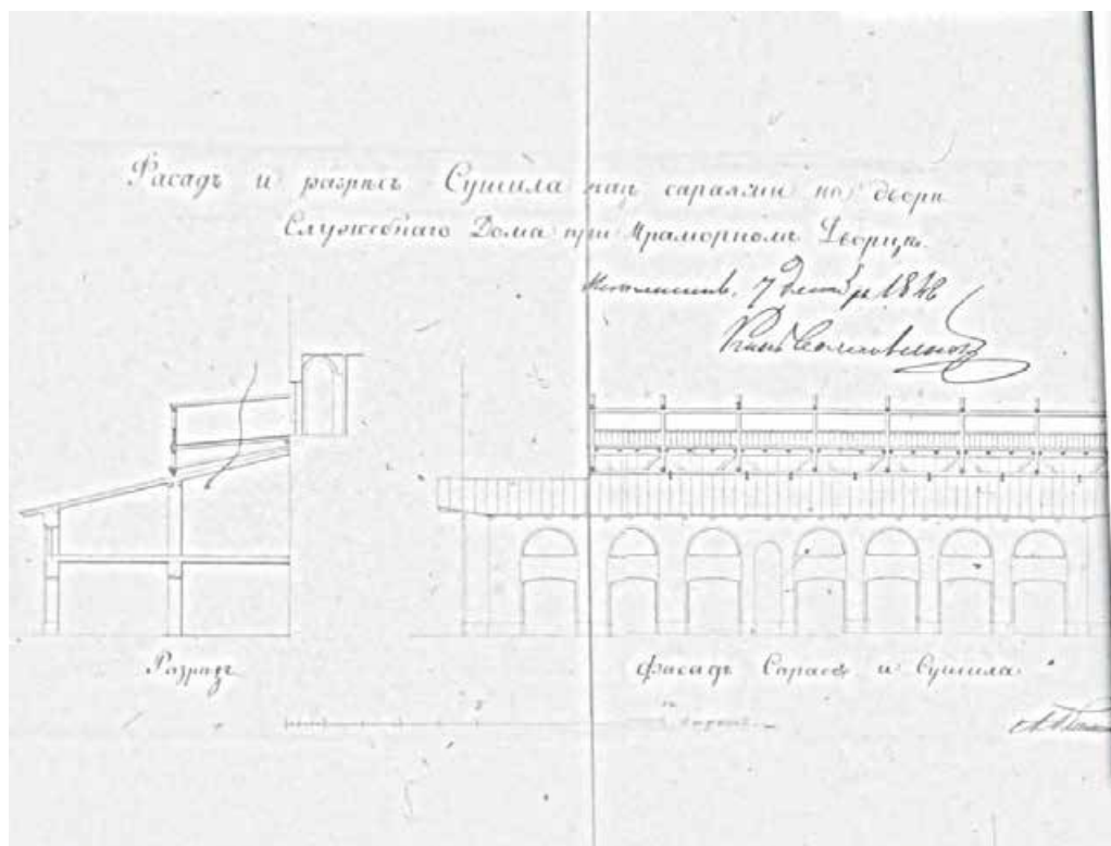
Илл. 16. Фасад и разрез сушила над сараями на дворе Служебного дома при Мраморном дворце. 1846 г. Архитектор А.П. Брюллов. РГИА. Ф. 485. Оп. 2. Д. 65. Л. 8.
