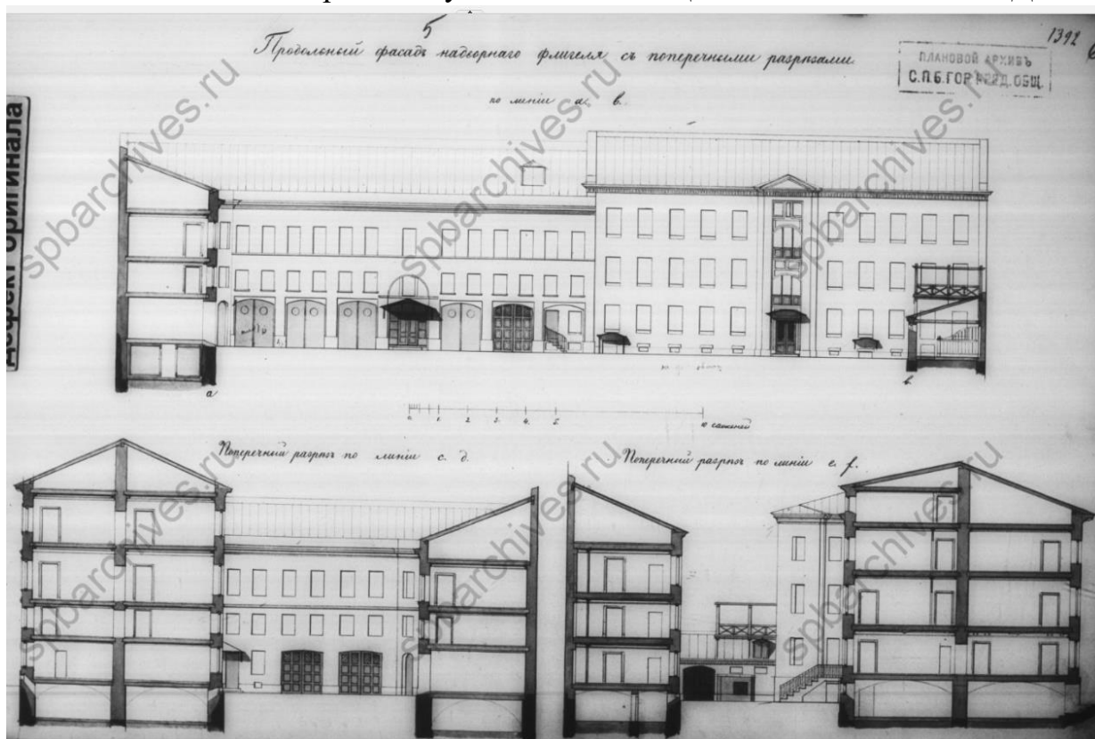
Илл. 14. Продольный фасад надворного флигеля с поперечными разрезами. Поперечные разрез по лицовому и дворовому флигелям. 1891 г. // ЦГИА СПб Ф. 515 Оп. 4 Д. 614
