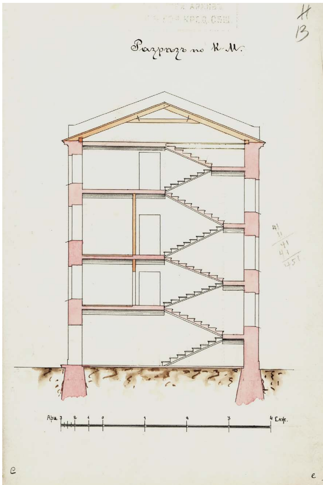
17. Моховая улица, участок № 48/15. Проект архитектора А. Веретенникова 1901 г. ЦГИА СПб Фонд 515, Описание 4, Дело 3580, Листы 13. Разрез по К.М.
