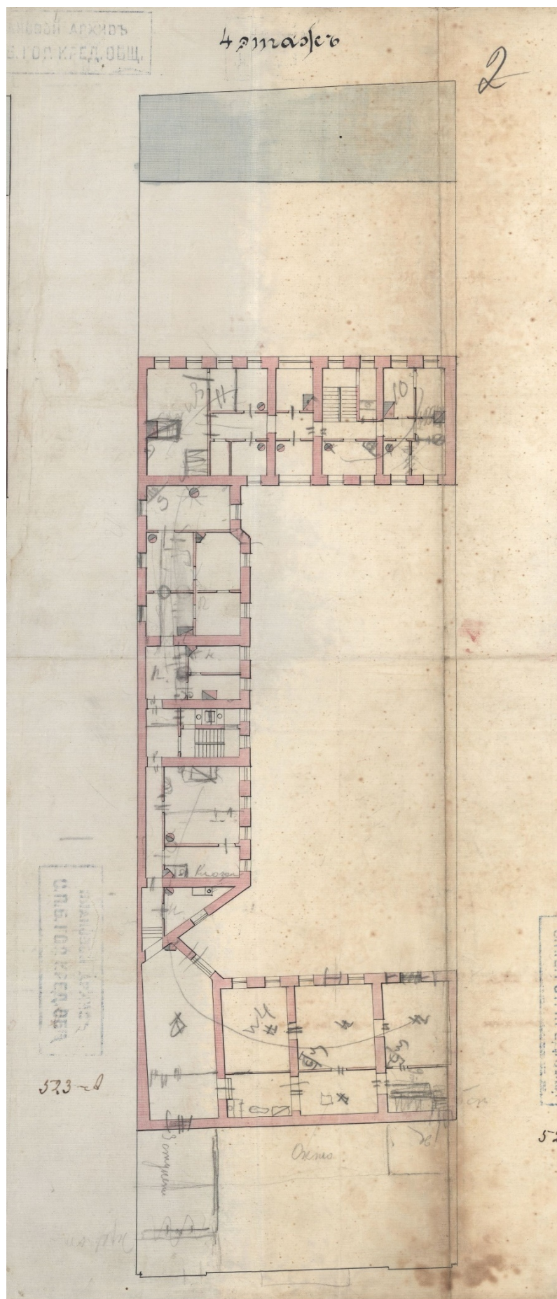
11. Моховая улица, участок № 48/15. Проект архитектора Л. Бонштедта 1851 г. - первый вариант проекта. ЦГИА СПб Фонд 515, Опись 4, Дело 3580, Листы 5 – 8. План 4 этажа.
