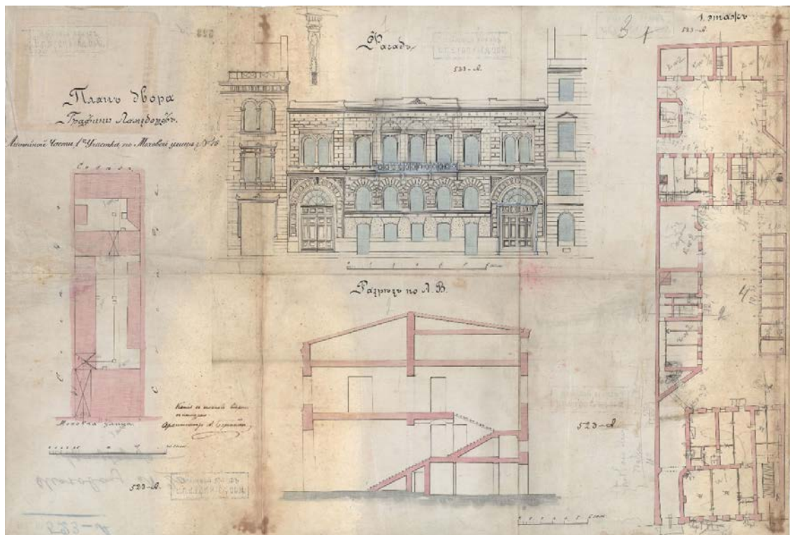
5. Моховая улица, участок № 48/15. Проект архитектора Л. Бонштедта 1851 г. - первый вариант проекта. ЦГИА СПб Фонд 515, Опись 4, Дело 3580, Листы 1 – 4.
