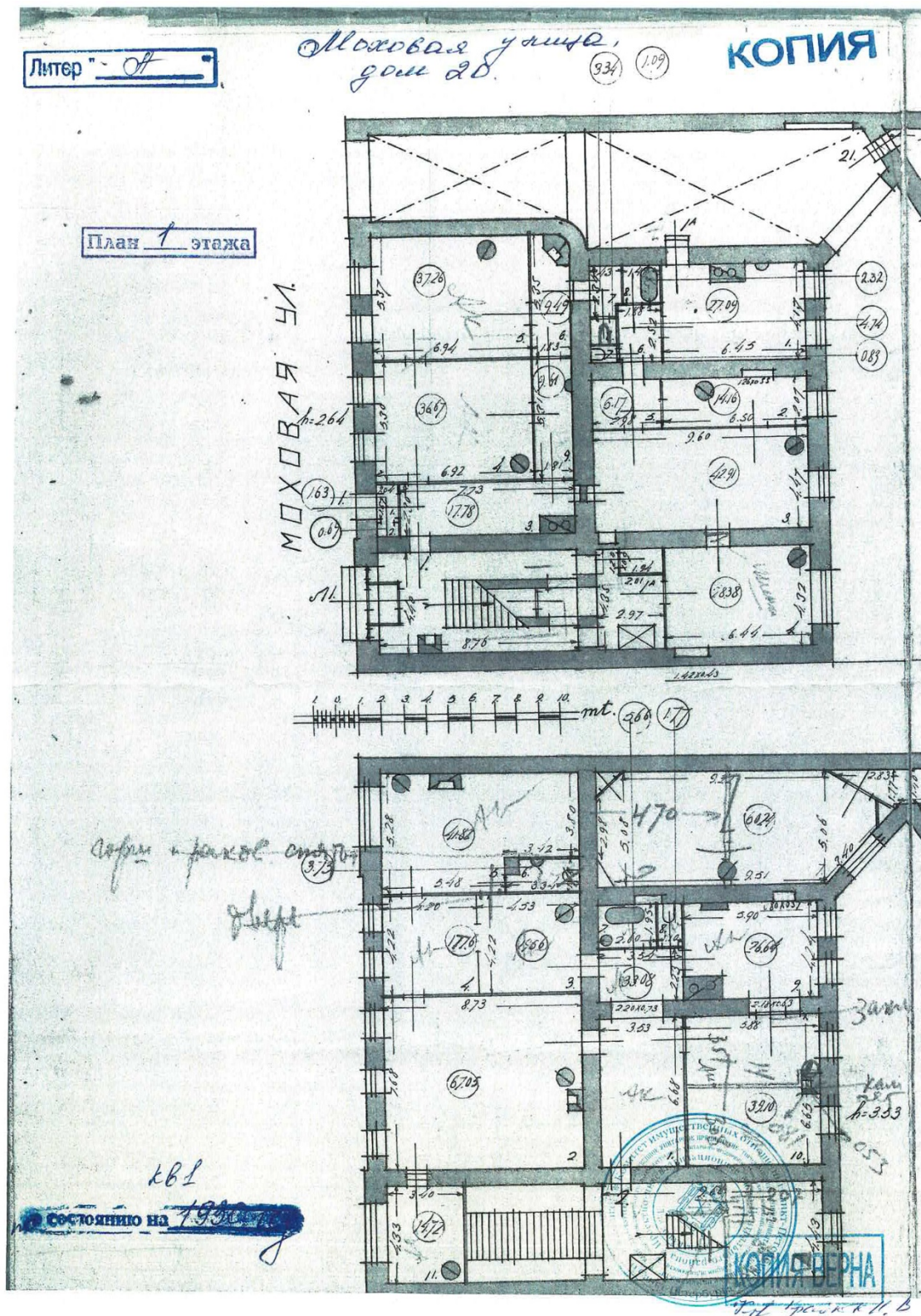
25. Планы ПИБ по состоянию на 1930 г. На плане первого этажа по шестой световой оси показан дверной проем.
