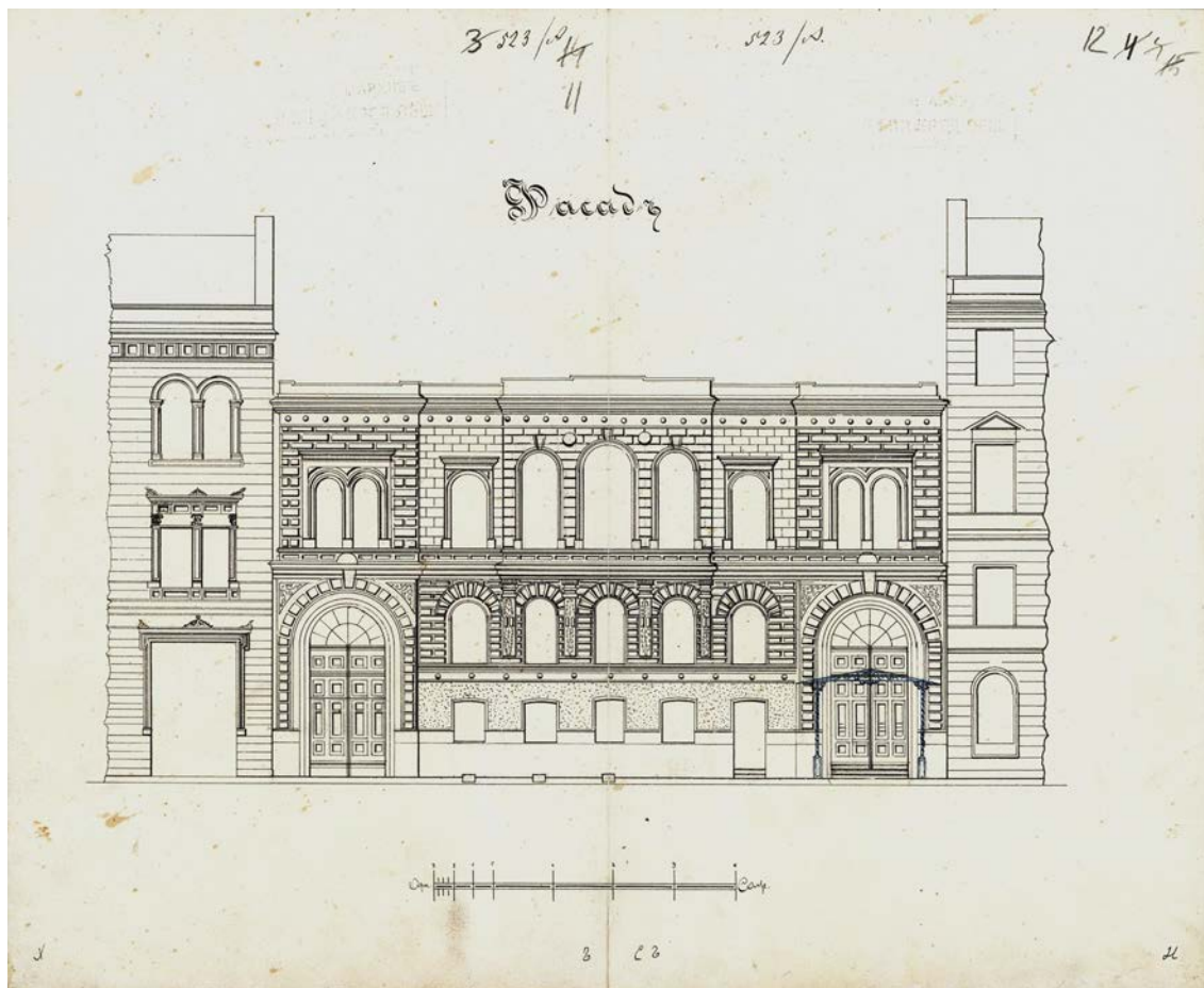
15. Моховая улица, участок № 48/15 Проект архитектора А. Веретенникова 1901 г. ЦГИА СПб Фонд 515, Опись 4, Дело 3580, Листы 11 – 12. Лицевой фасад. Промежуточный вариант лицевого фасада по Моховой улице, существует один (непарадный) вход по 6 оси.
