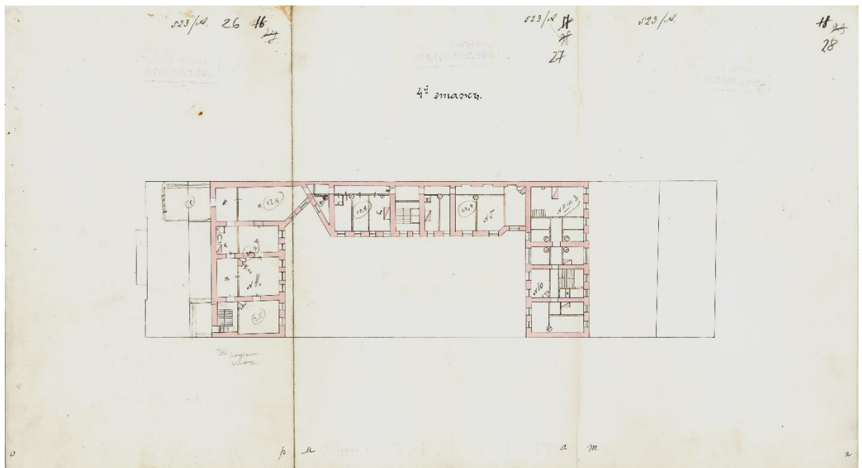
22. Моховая улица, участок № 48/15. Проект архитектора А. Веретенникова 1901 г. ЦГИА СПб Фонд 515, Описание 4, Дело 3580, Листы 26 – 28. Окончательный вариант плана четвертого этажа.
