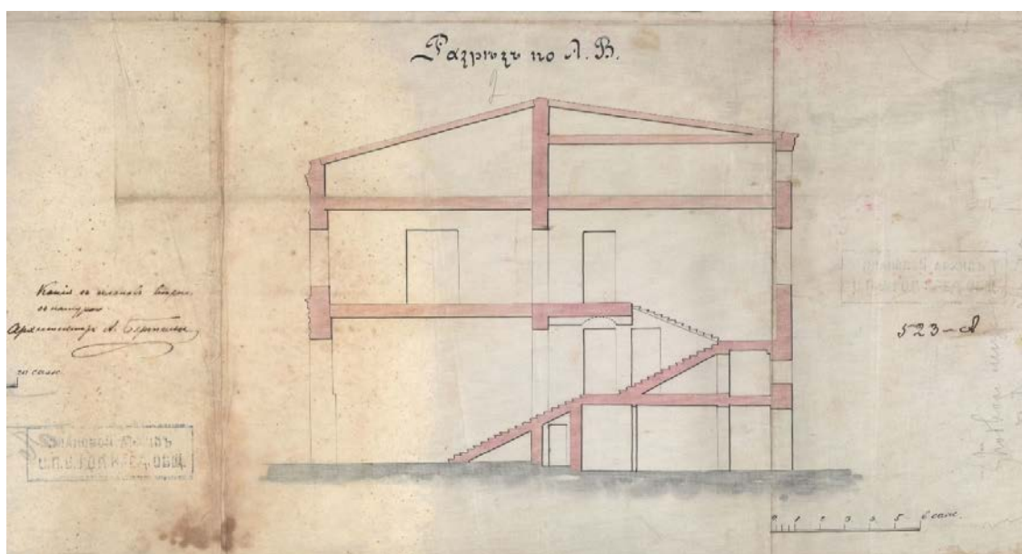
13. Моховая улица, участок № 48/15. Проект архитектора Л. Бонштедта 1851 г. - первый вариант проекта. ЦГИА СПб Фонд 515, Опись 4, Дело 3580, Листы 1 – 4. Фрагмент. Разрез по А.В.
