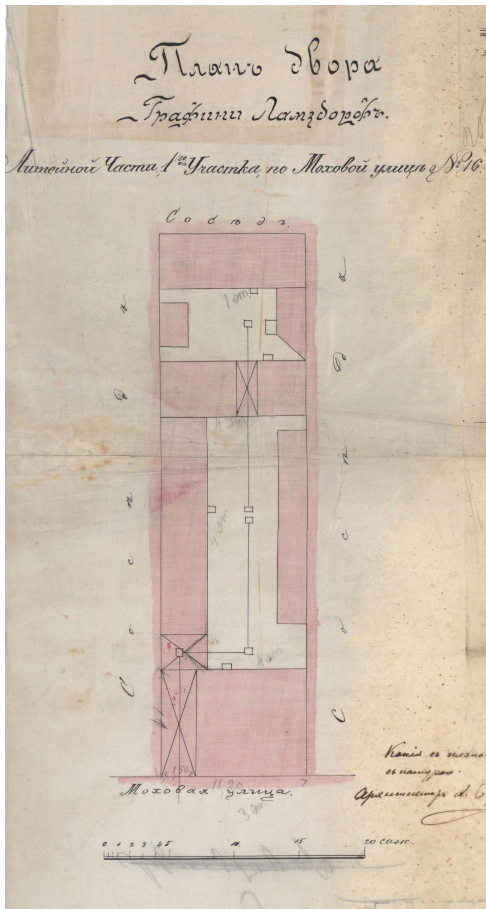
7. Моховая улица, участок № 48/15. Проект архитектора Л. Бонштедта 1851 г. - первый вариант проекта. ЦГИА СПб Фонд 515, Опись 4, Дело 3580, Листы 1 – 4. Фрагмент. План двора Графини Ламздорф. Литейной части 1-го участка, по Моховой улице, № 16.
