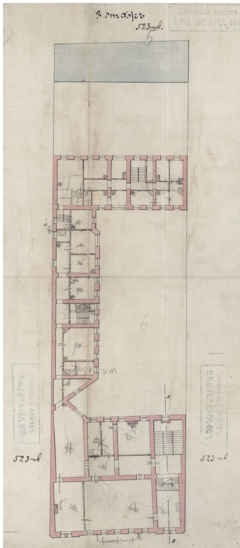
10. Моховая улица, участок № 48/15. Проект архитектора Л. Бонштедта 1851 г. - первый вариант проекта. ЦГИА СПб Фонд 515, Опись 4, Дело 3580, Листы 5 – 8. План 3 этажа.
