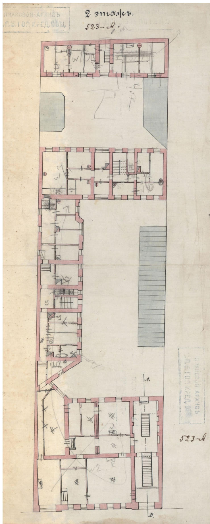
9. Моховая улица, участок № 48/15. Проект архитектора Л. Бонштедта 1851 г. - первый вариант проекта. ЦГИА СПб Фонд 515, Опись 4, Дело 3580, Листы 5 – 8. План 2 этажа.
