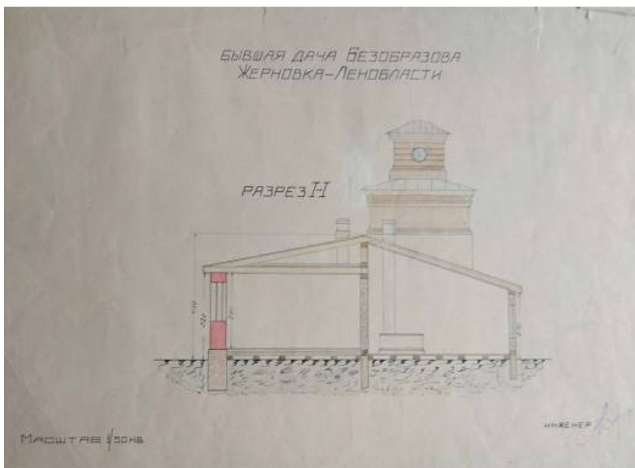
33. Бывшая дача Безобразова. Разрез. 1946 г. Архив КГИОП. 32/Г-24
