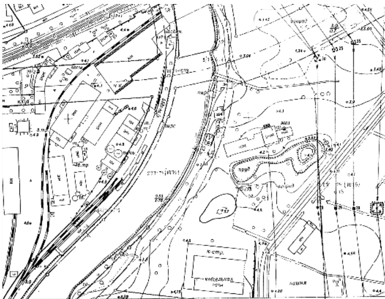
15. Топографическая съемка. 1977 г. Трест ГРИИ.
