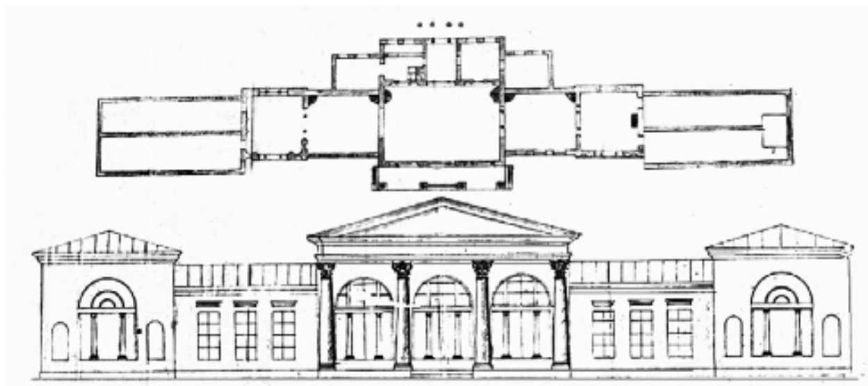
22. Дача Безобразовых. План, фасад. Н. Фомин. 1923–1925 гг. ЦГА СПб. Ф. 2555. Оп. 1. Д. 1181
