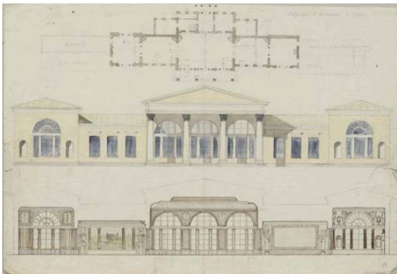
21. Дача Безобразова в имении «Екатериновка», станция «Жерновка». Обмерный чертеж. Арх. А. Соколов. 1924 г. Санкт-Петербургское государственное бюджетное учреждение культуры "Государственный музей истории Санкт-Петербурга". Номер по КП (ГИК): ГМИ СПб 167122. Инвентарный номер: ГМИ СПб Инв.№-I-A-2582 и. Номер в Госкаталоге: 58213846
