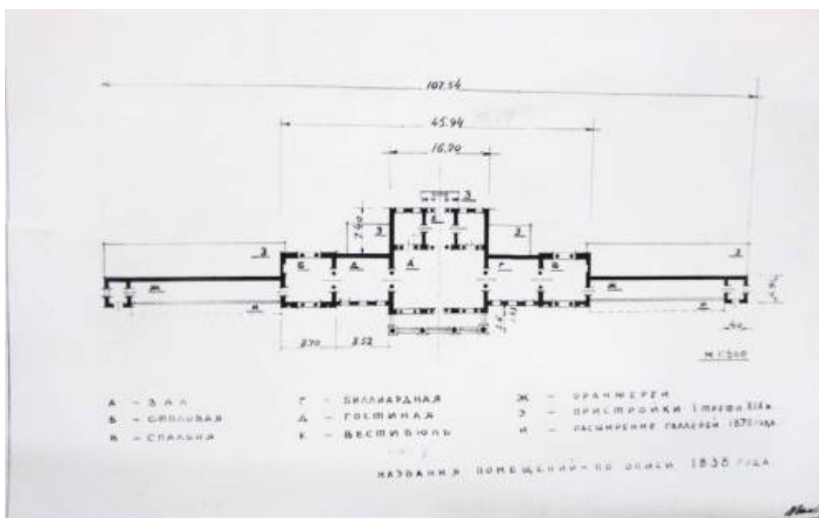
24. Анализ планировочных изменений главного дома усадьбы Безобразовых. Архив КГИОП. П 32. Н-157. Архитектурный паспорт здания общежития Охтинского лесозавода (бывшая дача Безобразовых). Сост.: Вальберг В.П., Липман А.И. 1939. С. 35
