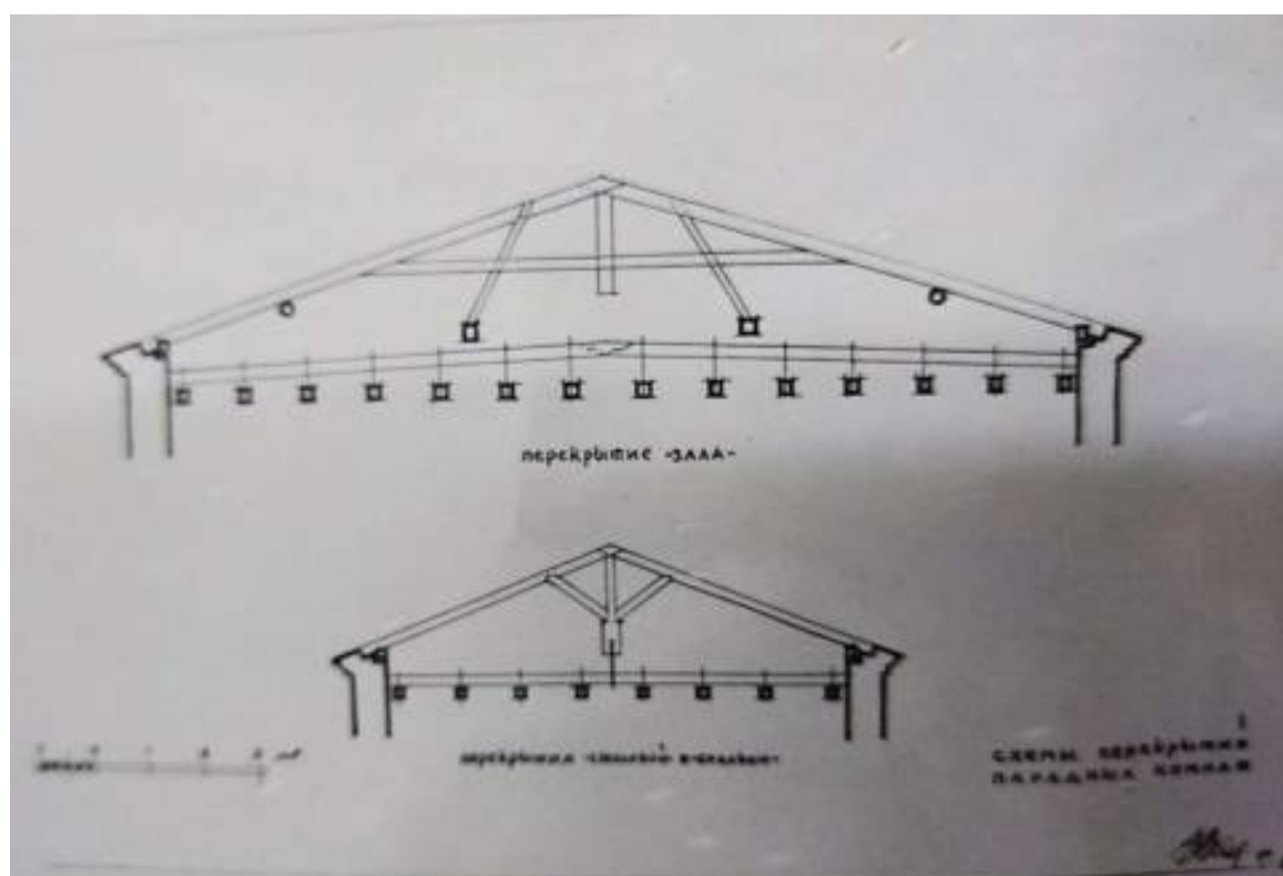
25. Чертеж перекрытия зала, столовой и спальни. Архив КГИОП. П 32. № Н-157. Архитектурный паспорт здания общежития Охтинского лесозавода (бывшая дача Безобразовых). Сост.: Вальберг В.П., Липман А.И. 1939. С. 40
