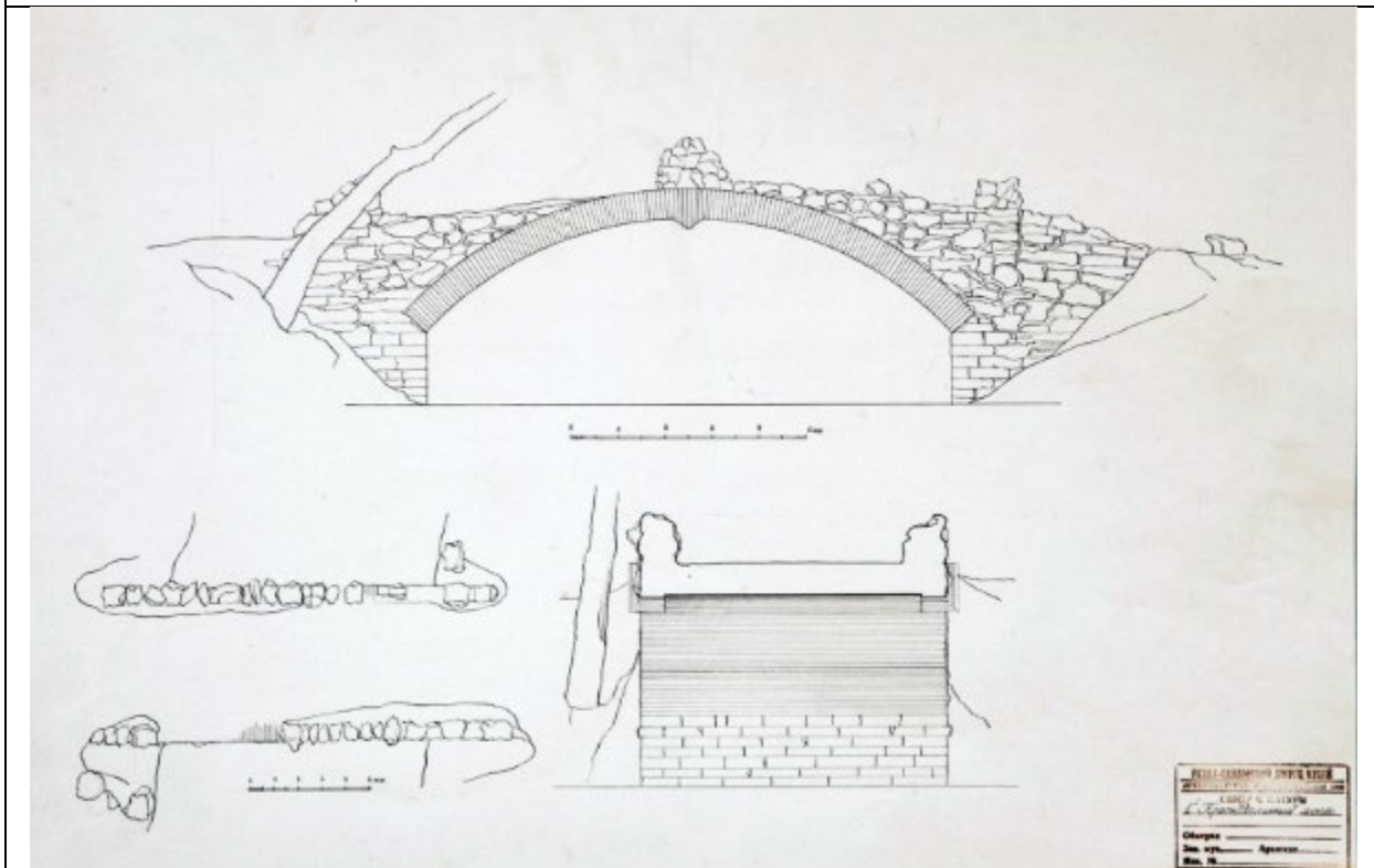
2. Обмер с этюдами для Ново-Сильвийского моста. 1939 г.
