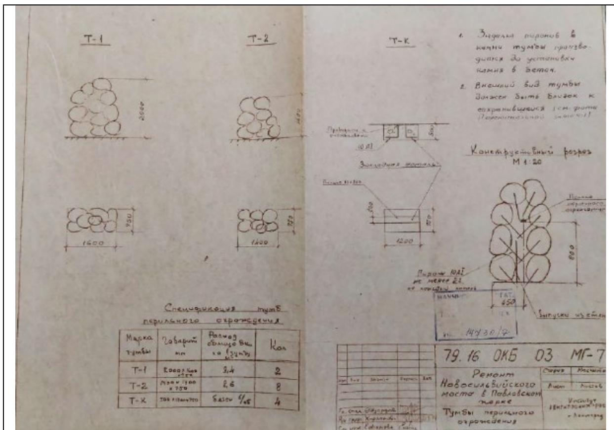
5. Тумбы перильного ограждения. Проект ремонта Ново-Сильвийского моста в Павловском парке, 1979 г.
