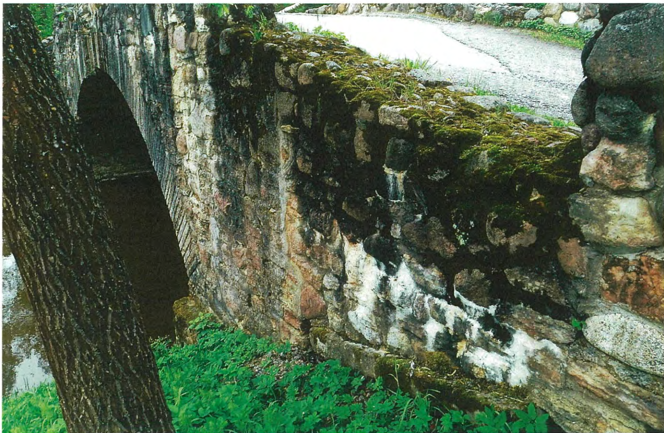
3. Фрагмент устоев моста с северного фасада.
