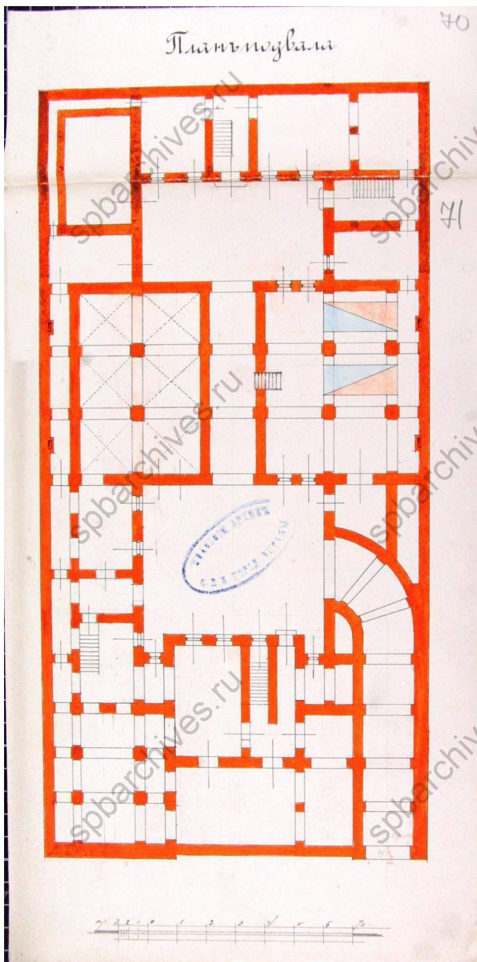
10. План подвала. 1896 г. // ЦГИА СПб. Фонд 513. Опись 102. Дело 9818.
