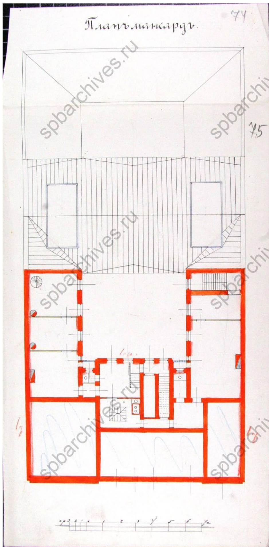
12. План мансарды. 1896 г. // ЦГИА СПб. Фонд 513. Опись 102. Дело 9818.
