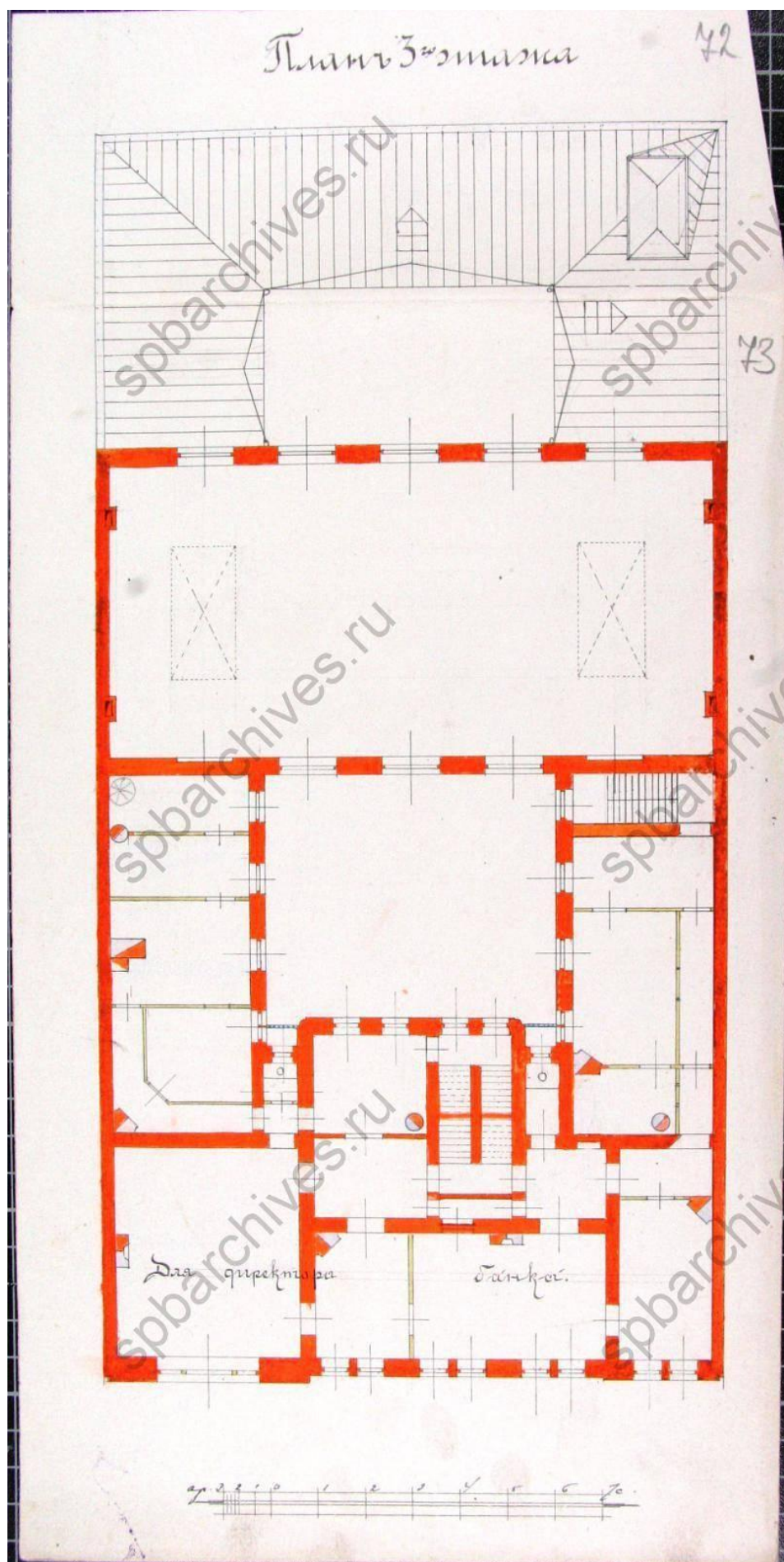
11. План 3-го этажа. 1896 г. // ЦГИА СПб. Фонд 513. Опись 102. Дело 9818.
