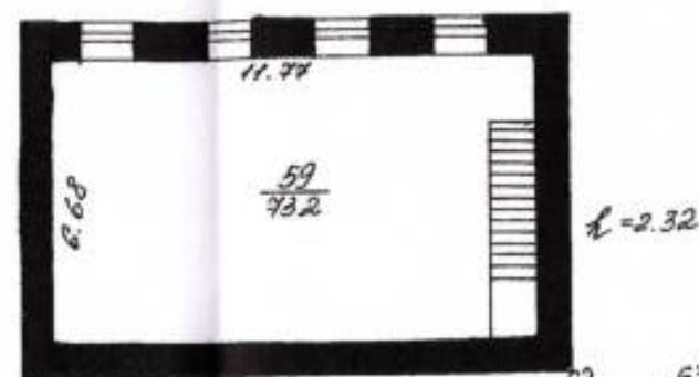
План антресоли
