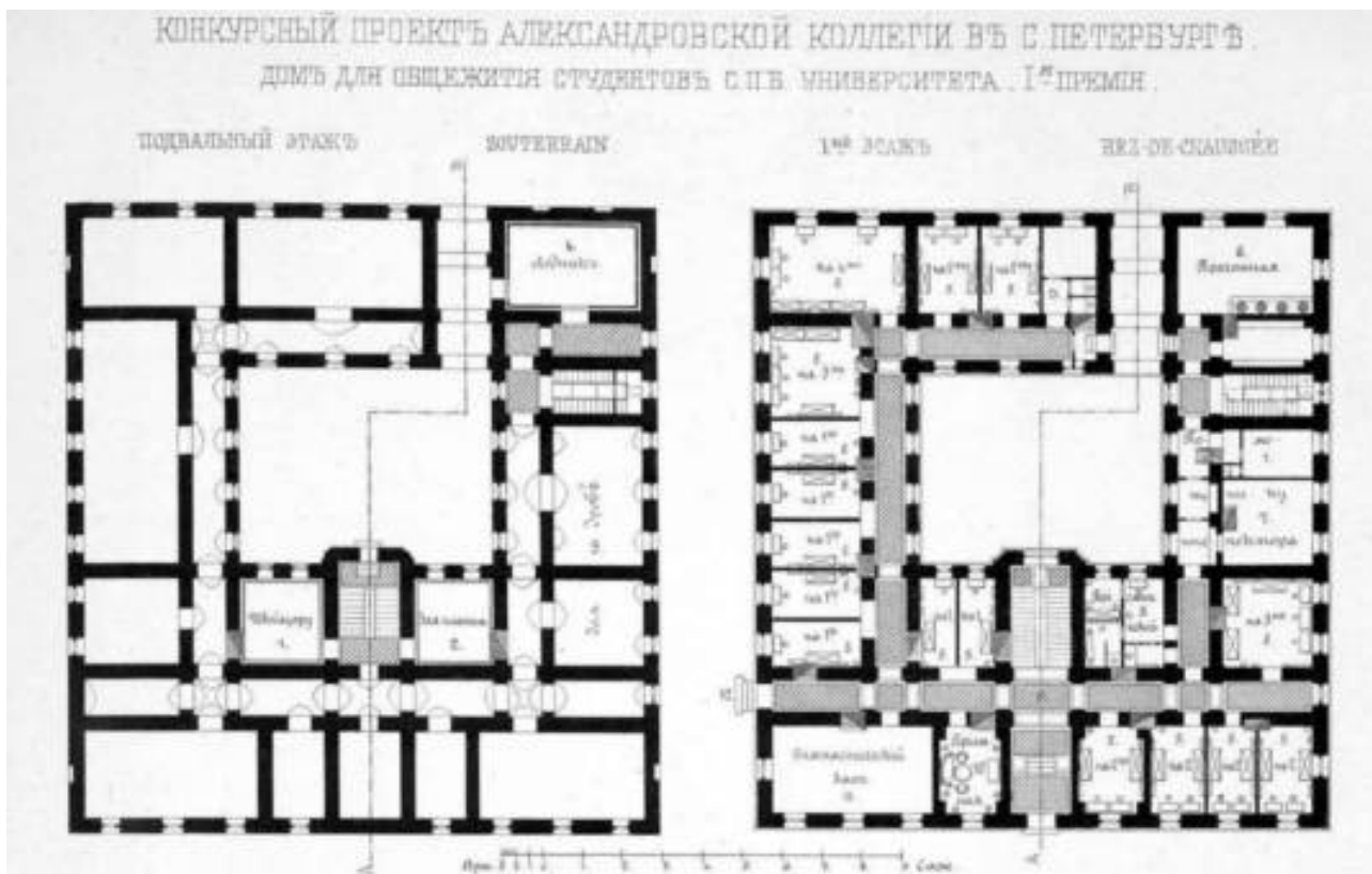
29. Конкурсный проект Александровской коллегии в С. Петербурге. Дом для общежития студентов. 1-я премия. Подвальный и 1-й этажи. 1881 г. Из: «Зодчий». 1881. № 12. Л. 15.
