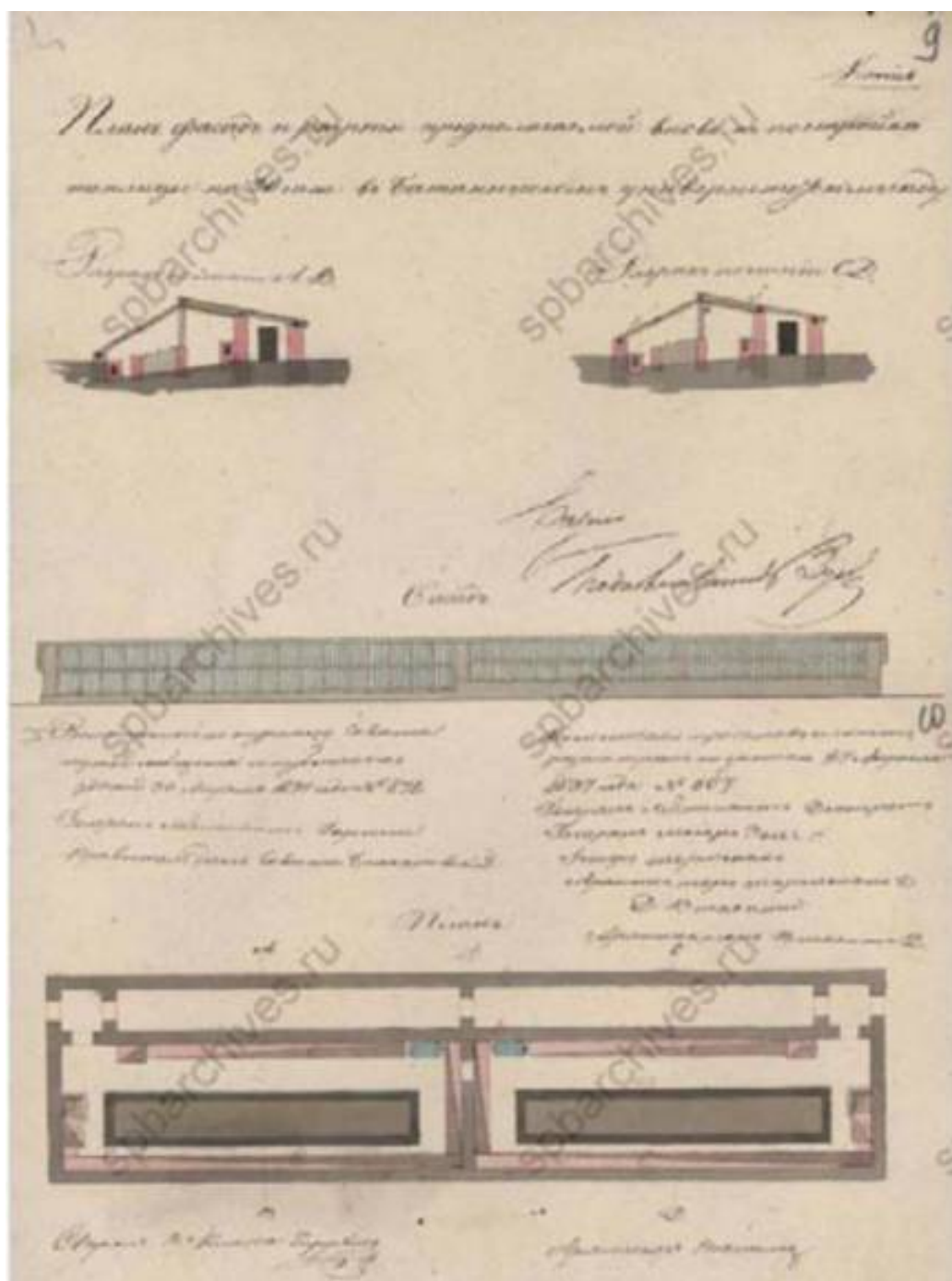
48. План, фасад и разрез вновь предполагаемой к постройке теплицы. ЦГИА СПб.
