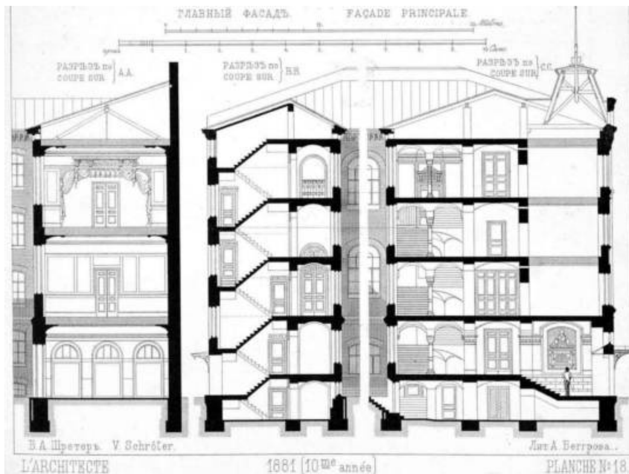
32. Конкурсный проект Александровской коллегии в С. Петербурге. 2-я премия. Разрезы. 1881 г. Из: «Зодчий». 1881. № 12. Л. 18.
