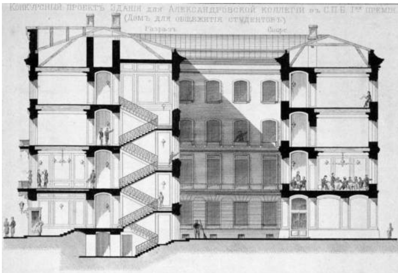
28. Конкурсный проект Александровской коллегии в С. Петербурге. Дом для общежития студентов. 1-я премия. Разрез. 1881 г. Из: «Зодчий». 1881. № 12. Л. 16.
