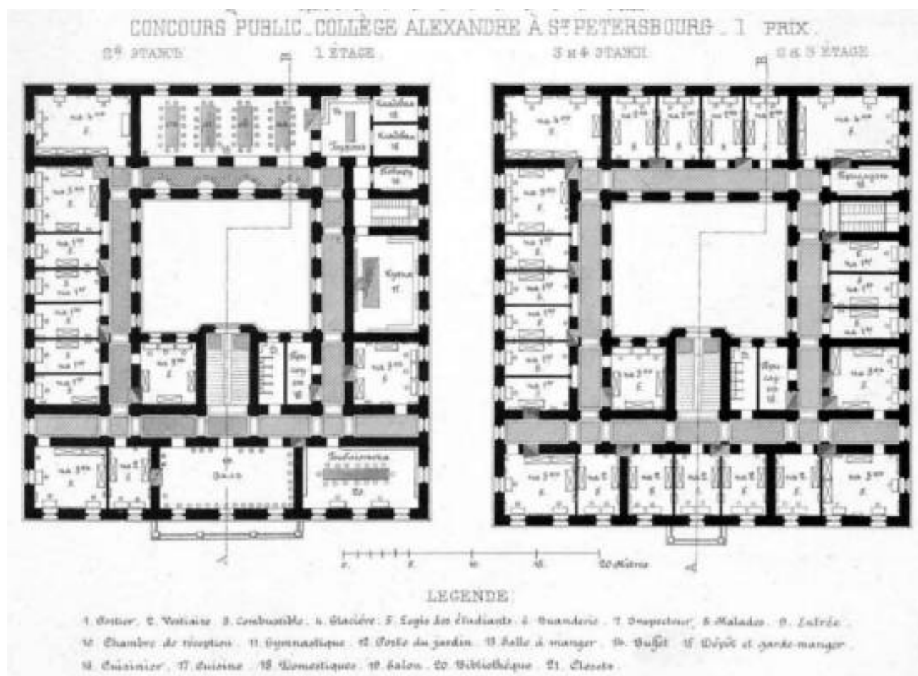
30. Конкурсный проект Александровской коллегии в С. Петербурге. Дом для общежития студентов. 1-я премия. 2–4-й этажи. 1881 г. Из: «Зодчий». 1881. № 12. Л. 15.
