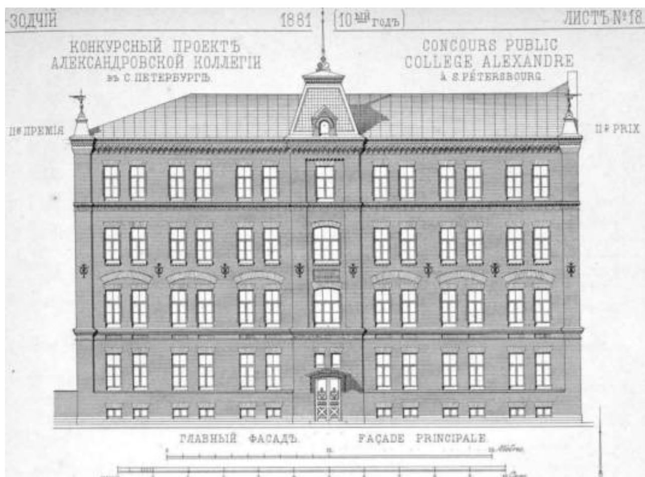
31. Конкурсный проект Александровской коллегии в С. Петербурге. 2-я премия. Главный фасад. 1881 г. Из: «Зодчий». 1881. № 12. Л. 18.
