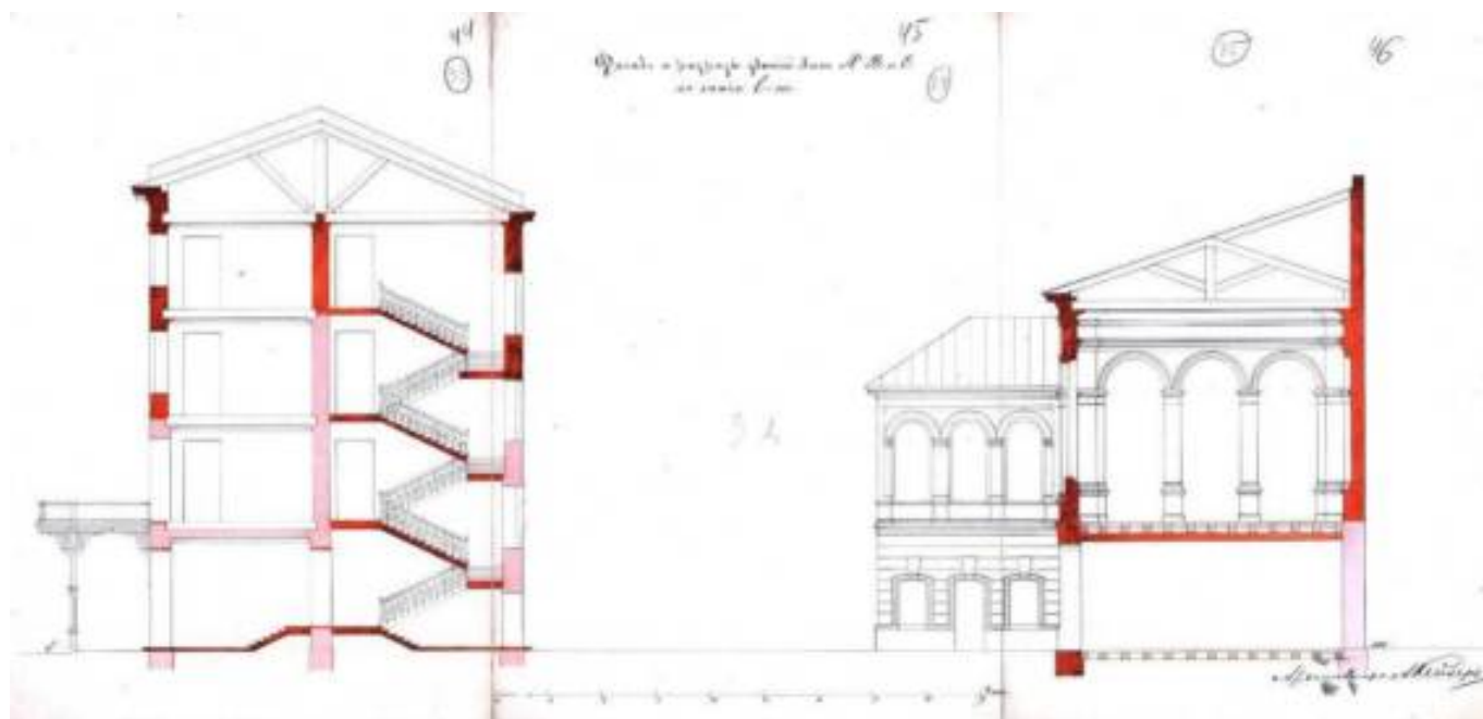
Илл.18. Фасад и разрез зданий лит. А', В и С по линии I-m. 1873 г. ЦГИА СПб. Фонд 513. Опись 102. Дело 4682. Л.44-46.
