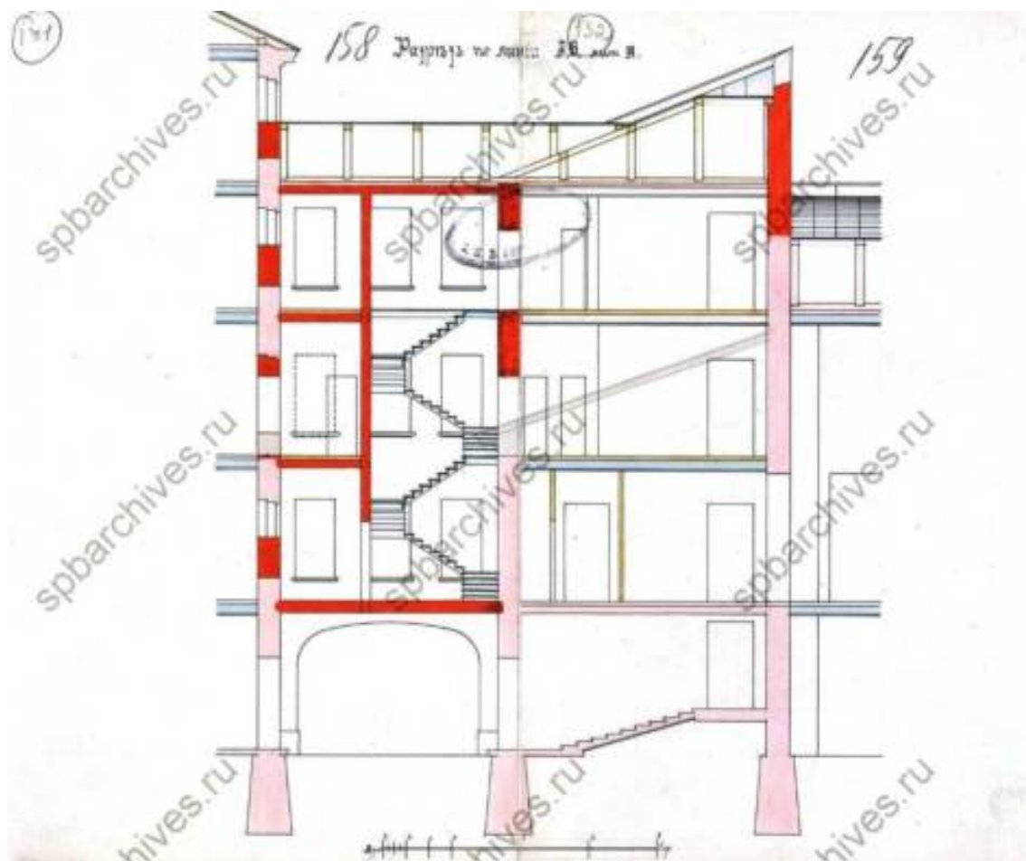
Илл.48. Разрез по линии А-В. 1904 г. ЦГИА СПб. Фонд 513. Опись 102. Дело 4682. Л.158-159.
