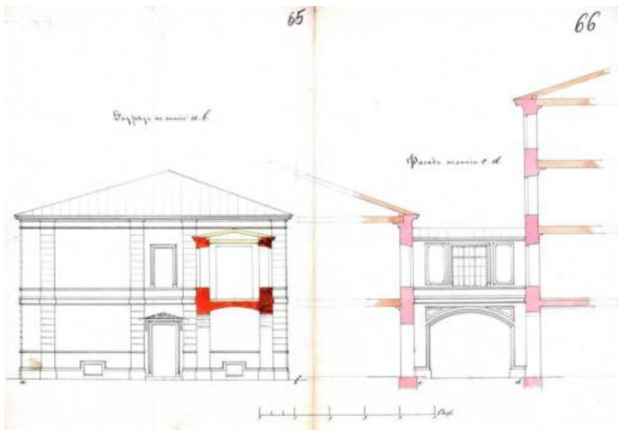
Илл.23. Разрез по линии а-в, фасад по линии с-д. 1882 г. ЦГИА СПб. Фонд 513. Описание 102. Дело 4682. Л.65-66.
