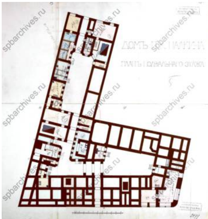
Илл.57. План подвала. 1910 г. ЦГИА СПб. Фонд 515. Опись 4. Дело 3709. Л.13-18.
