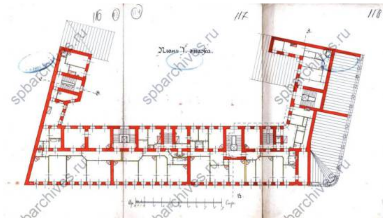
Илл.38. План 5-го этажа. 1904 г. ЦГИА СПб. Фонд 513. Опись 102. Дело 4682. Л.116-118.
