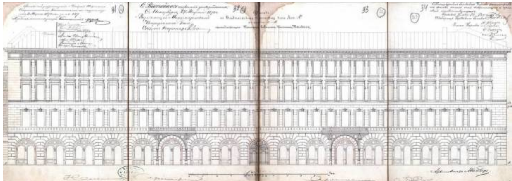
Илл.15. Фасад по Владимирскому проспекту дома лит. А' по линии с-d, принадлежащего коммерции советнику К.П. Палкину. 1873 г. ЦГИА СПб. Фонд 513. Опись 102. Дело 4682. Л.31-34.
