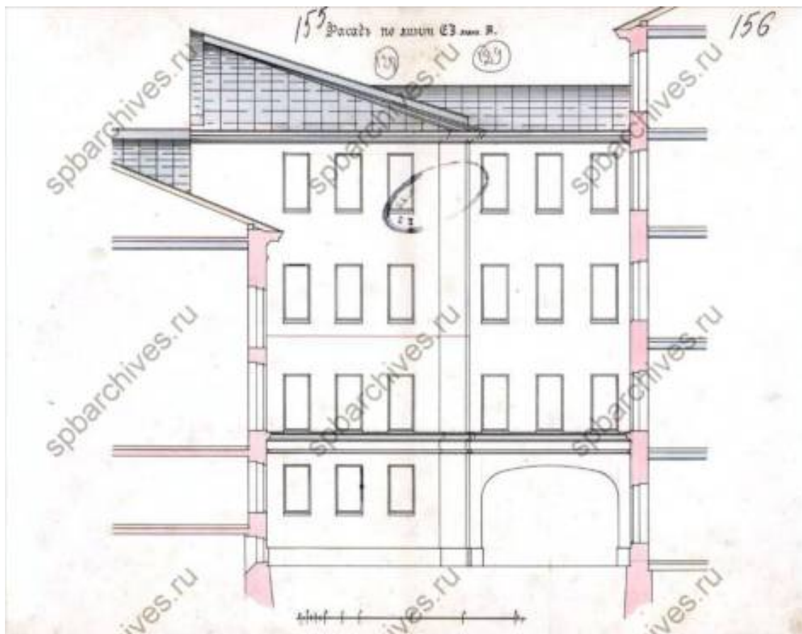
Илл.47. Фасад по линии С-Д. 1904 г. ЦГИА СПб. Фонд 513. Опись 102. Дело 4682. Л.155-156.
