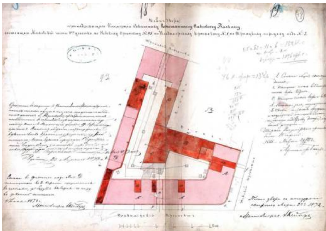
Илл.11. План двора принадлежащего коммерции советнику К.П. Палкину, состоящего Московской части 1-го участка по Невскому пр. №45, Владимирскому пр. №1 и Троицкому пер. под №2. 1873 г. ЦГИА СПб. Фонд 513. Опись 102. Дело 4682. Л.18-19.
