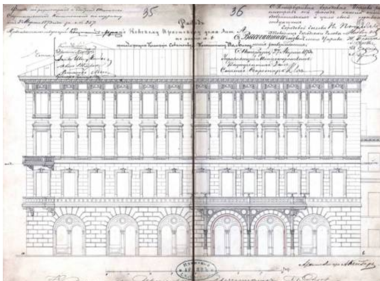
Илл.17. Фасад по Невскому пр. дома лит. А по линии a-b, , принадлежащего коммерции советнику К.П. Палкину. 1873 г. ЦГИА СПб. Фонд 513. Опись 102. Дело 4682. Л.35-36.
