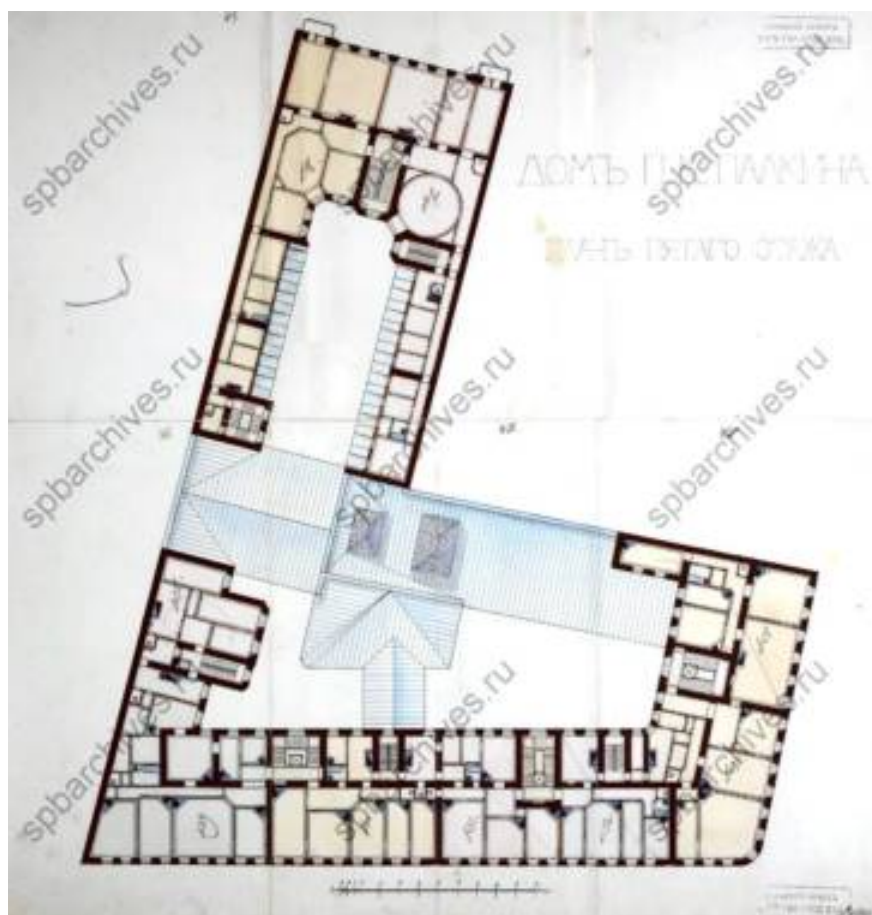
Илл.62. План 5-го этажа. 1910 г. ЦГИА СПб. Фонд 515. Описание 4. Дело 3709. Л.43-48.
