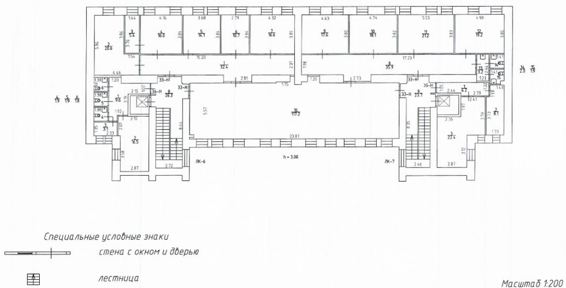
План 6 этажа
