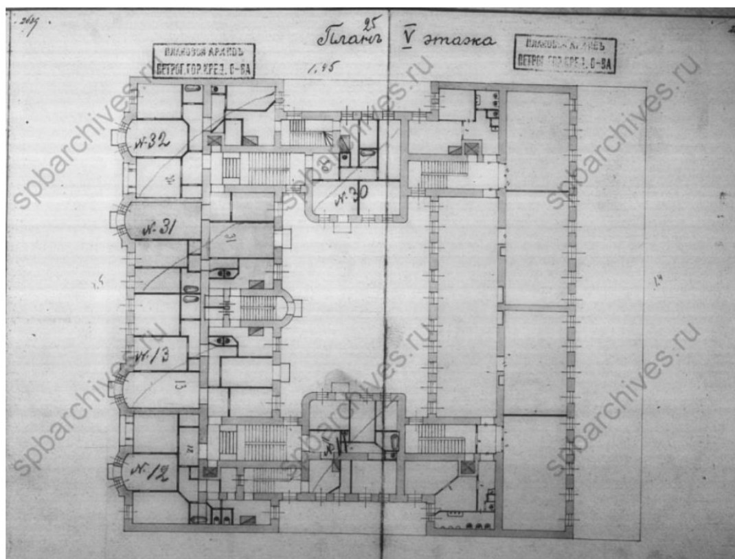
20. План пятого этажа. 1915 г. ЦГИА СПб. Ф. 515. Оп. 4. Д. 823. ЛЛ. 25-26.
