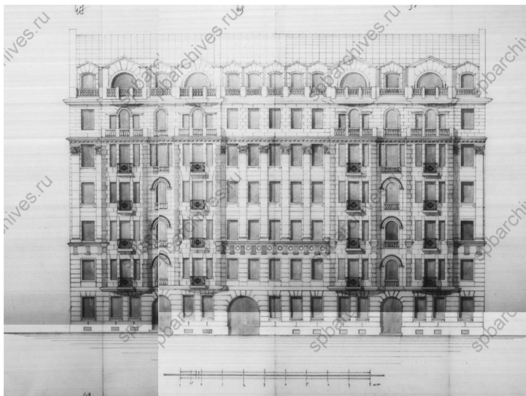
14. Фасад по Большой Гребенцкой (Пионерской) улице. 1915 г. ЦГИА СПб. Ф. 515. Оп. 4. Д. 823. Л. 14.
