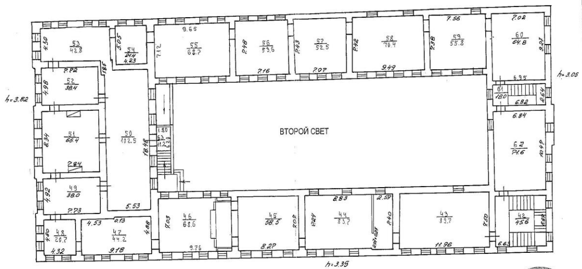
ПЛАН 2 ЭТАЖА
