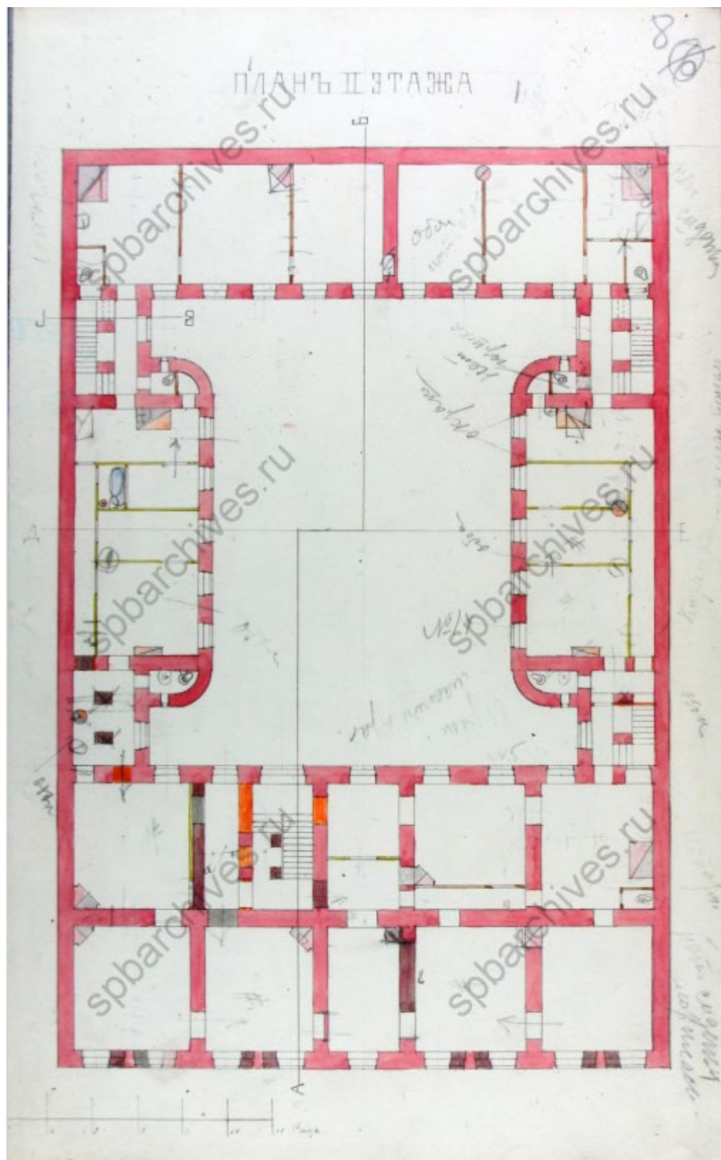
11. ЦГИА СПб. Фонд 513. Опись 102. Дело 81. Чертежи дома на участке, принадлежавшем Орлову-Давыдову по Гороховой ул., 5.
