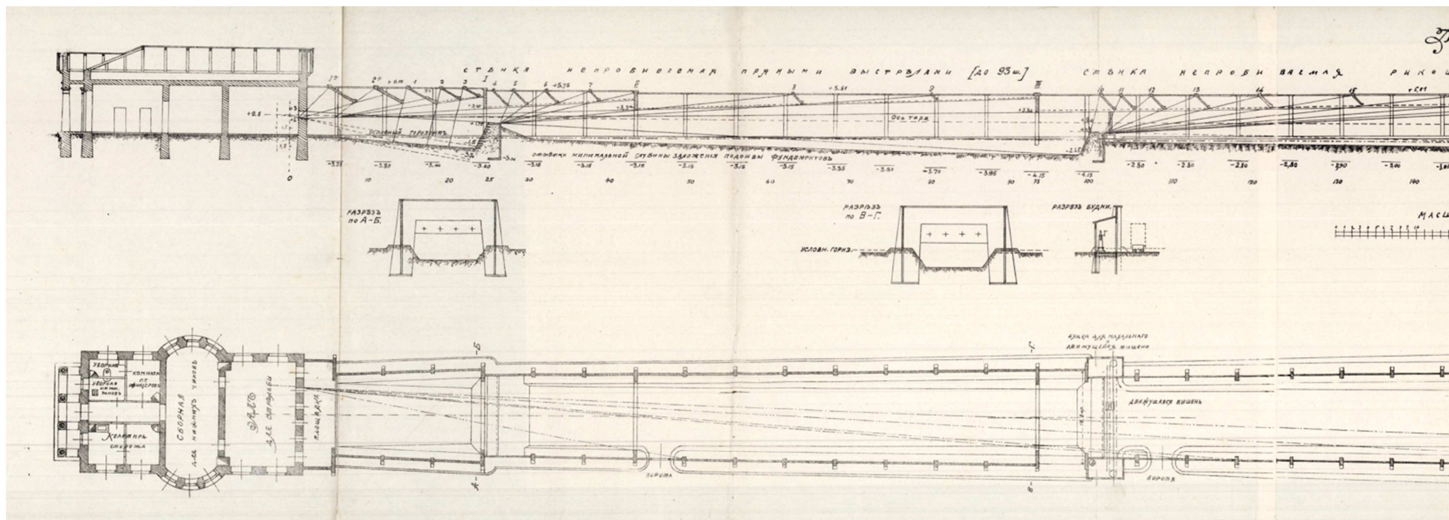
5. Проект тира лейб-гвардии Гусарского и Кирасирского Его Величества полков. (Б/д, б/п). [до 1917 г.] РГАВМФ.
