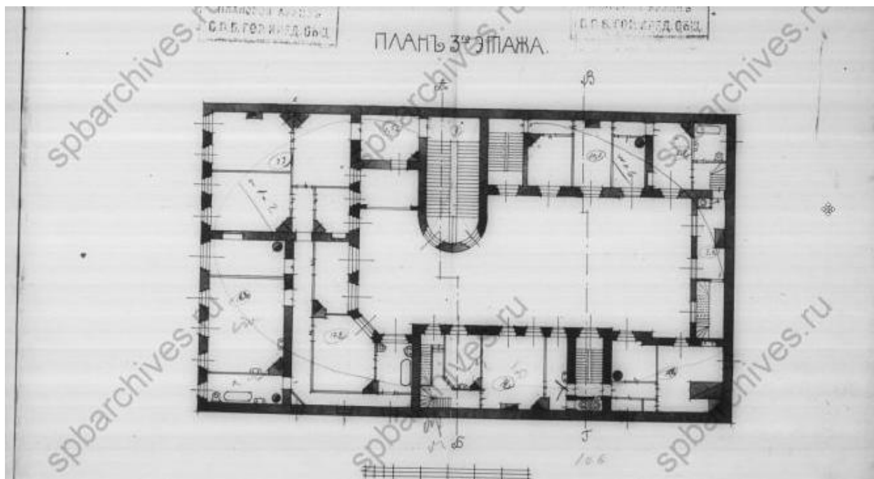
Илл. 3. Чертежи дома О.Б. и П.А. Столыпиных по Гагаринской ул.,5. Источник: ЦГИА СПб. Фонд 515. Описание 4. Дело 612.
