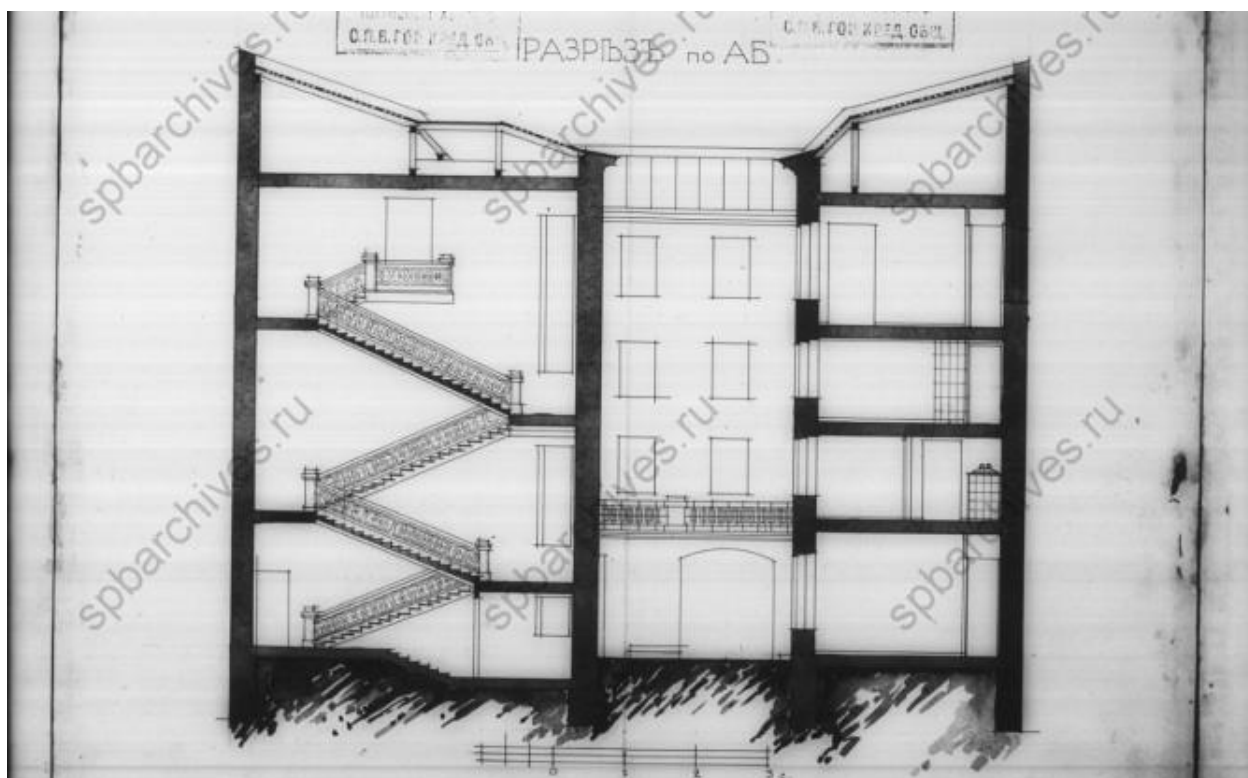
Илл. 2. Чертежи дома О.Б. и П.А. Столыпиных по Гагаринской ул.,5. Источник: ЦГИА СПб. Фонд 515. Опись 4. Дело 612.
