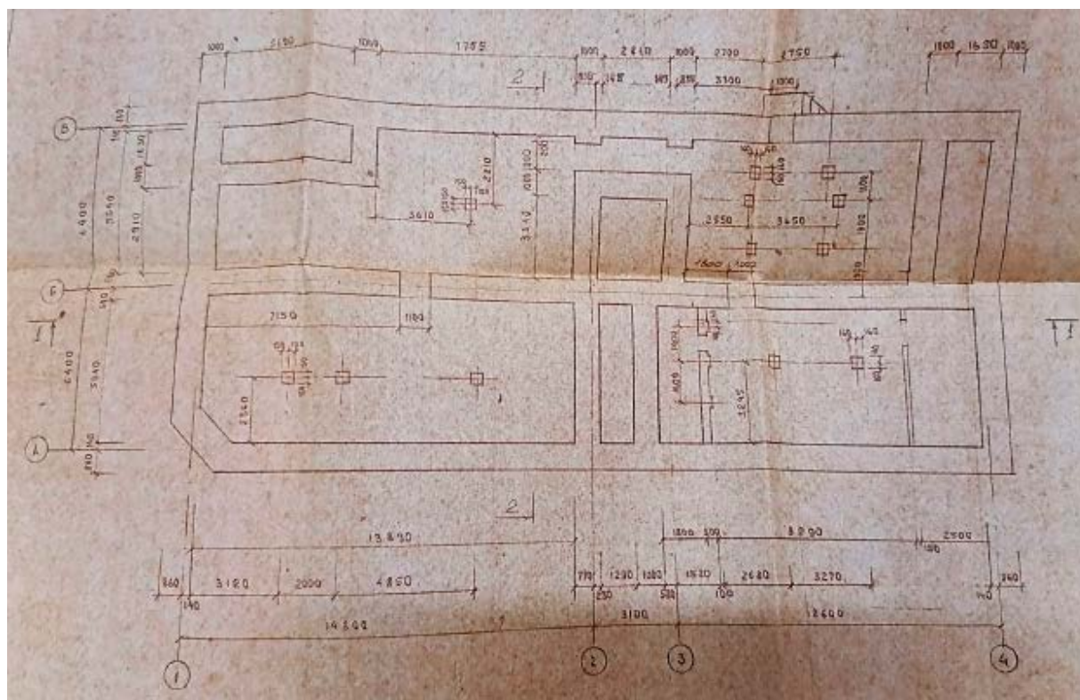
36. СПб., г. Ломоносов, Дворцовый пр., д.14/9 (пр. Юного Ленинца). План подвала. Технический отчет. Инженерное обследование здания. Кн.2. Обмерные чертежи, Сбс «Стройбытсервис», 1993г. Архив КГИОП, п-616-Г-6, пр.-136.
