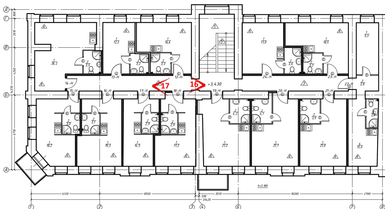
План 2-го этажа
