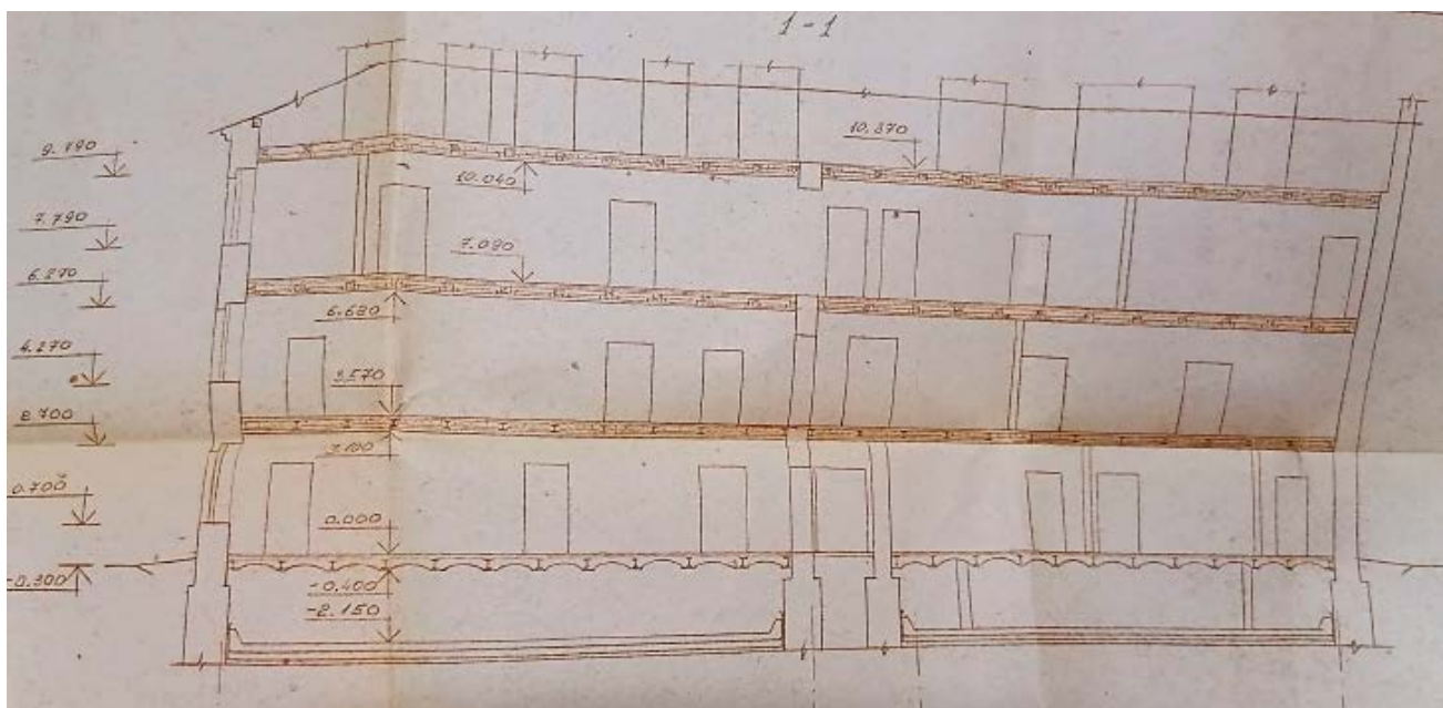
37. СПб., г. Ломоносов, Дворцовый пр., д.14/9 (пр. Юного Ленинца). Продольный разрез. Технический отчет. Инженерное обследование здания. Кн.2. Обмерные чертежи, Сбс «Стройбытсервис», 1993г. Архив КГИОП, п-616-Г-6, пр.-136.
