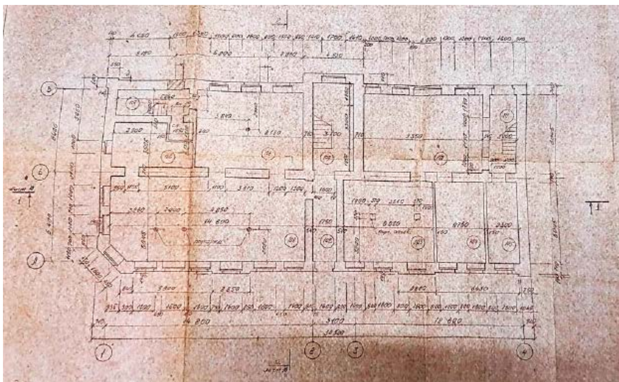
33. СПб., г. Ломоносов, Дворцовый пр., д.14/9 (пр. Юного Ленинца). План 1-го этажа. Технический отчет. Инженерное обследование здания. Кн.2. Обмерные чертежи, Сбс «Стройбытсервис», 1993г. Архив КГИОП, п-616-Г-6, пр.-136
