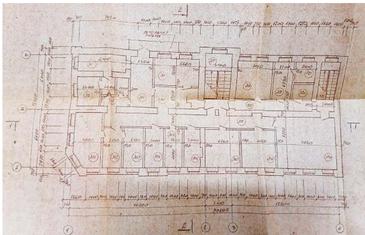
35. СПб., г. Ломоносов, Дворцовый пр., д.14/9 (пр. Юного Ленинца). План 3-го этажа. Технический отчет. Инженерное обследование здания. Кн.2. Обмерные чертежи, Сбс «Стройбытсервис», 1993г. Архив КГИОП, п-616-Г-6, пр.-136.
