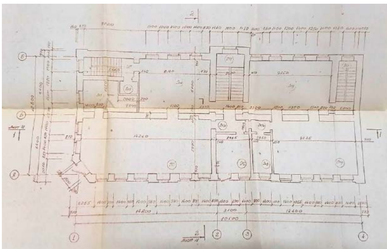
34. СПб., г. Ломоносов, Дворцовый пр., д.14/9 (пр. Юного Ленинца). План 2-го этажа. Технический отчет. Инженерное обследование здания. Кн.2. Обмерные чертежи, Сбс «Стройбытсервис», 1993г. Архив КГИОП, п-616-Г-6, пр.-136.
