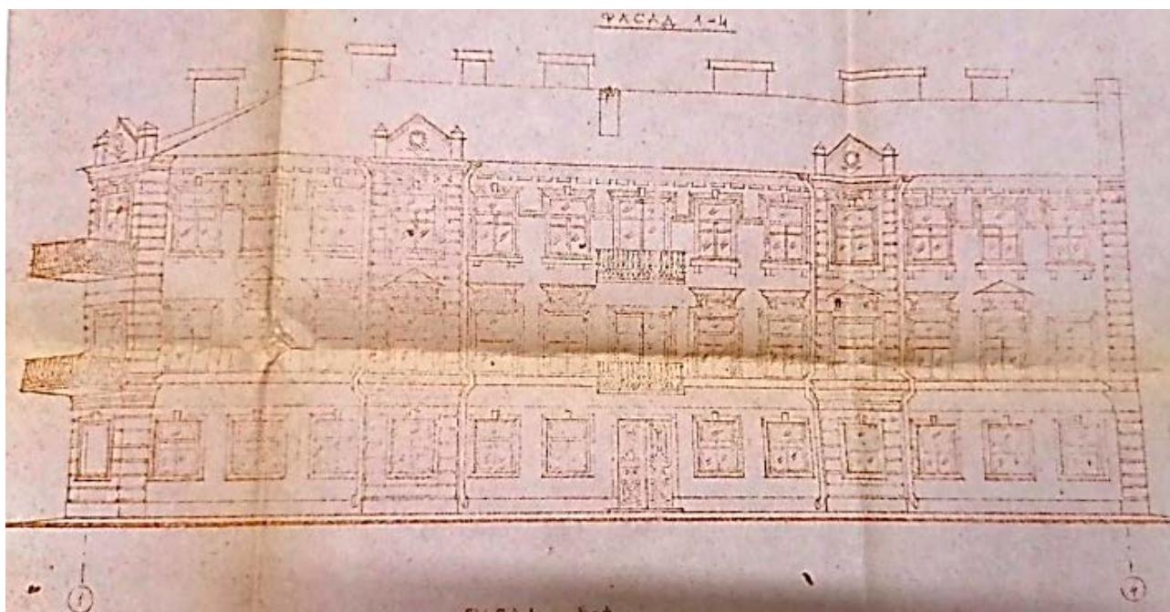
39. СПб., г. Ломоносов, Дворцовый пр., д.14/9 (пр. Юного Ленинца). Лицевой фасад по Дворцовому пр. Технический отчет. Инженерное обследование здания. Кн.2. Обмерные чертежи, Сбс «Стройбытсервис», 1993г. // Архив КГИОП, п-616-Г-6, пр.-136.
