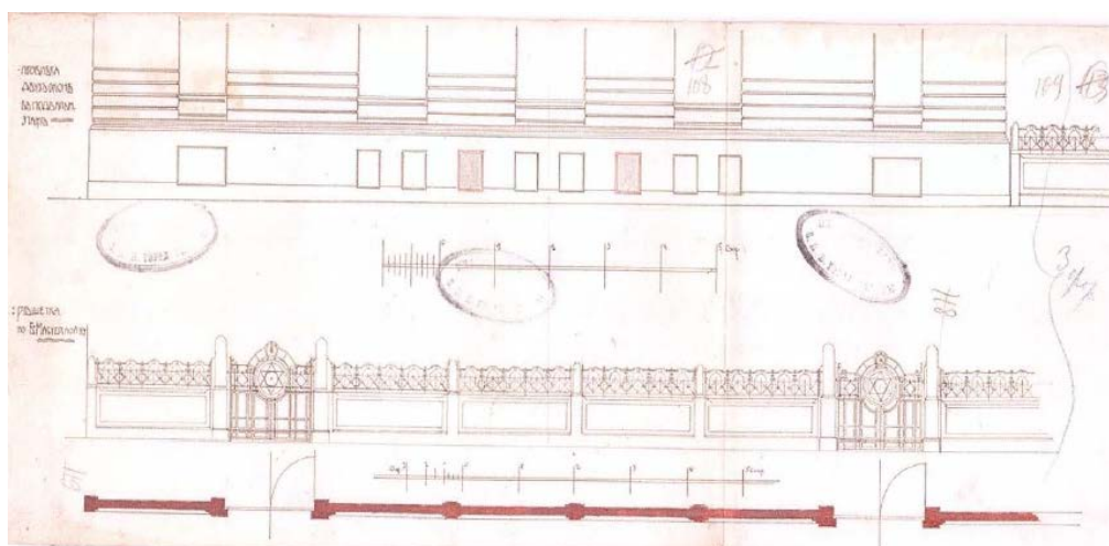
21. Проект. Здание Еврейского ремесленного училища. Пробивка окон в подвальном этаже. Архитектор Б.И. Гиршович. 1905г. Источники: ЦГИА СПб., Ф. 513, Оп. 102, Д.3645, Л.108-109
