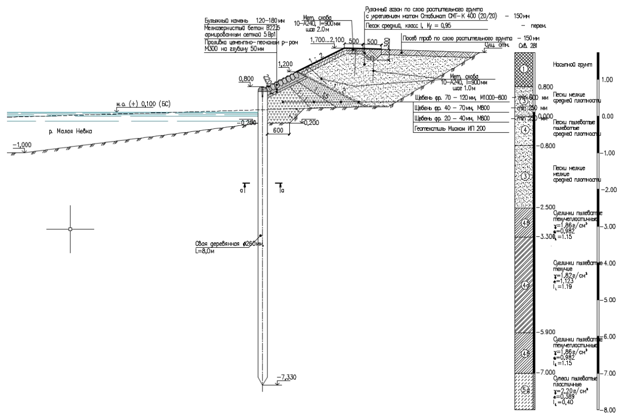
Илл.18. Поперечный разрез деревянного берегоукрепления вблизи пристани, по данным архива СПбГУ «Мостотрест», 2023 г.
