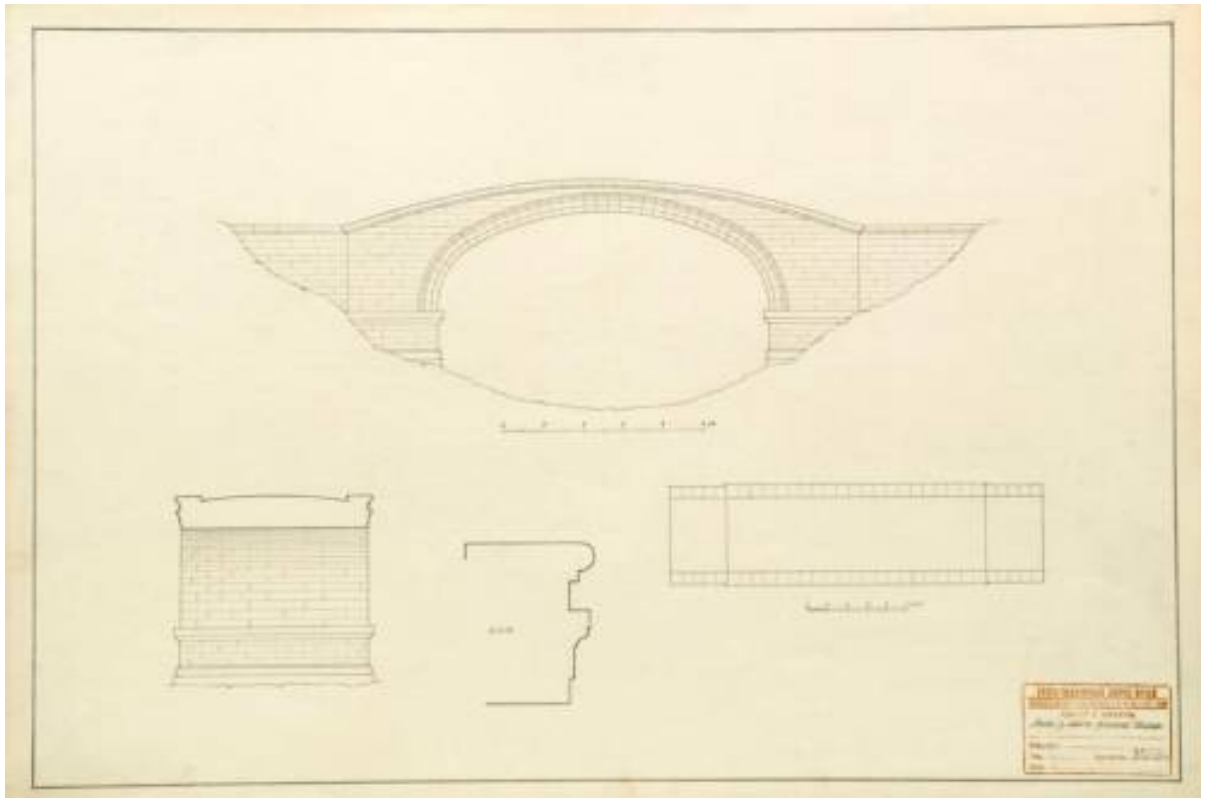
Ил. 19. 1940 г. Архитектор Соколов. Чертеж обмерный (ватман_тушь). Мост у левого флигеля. НВК-695_1. ГМЗ Павловск.
