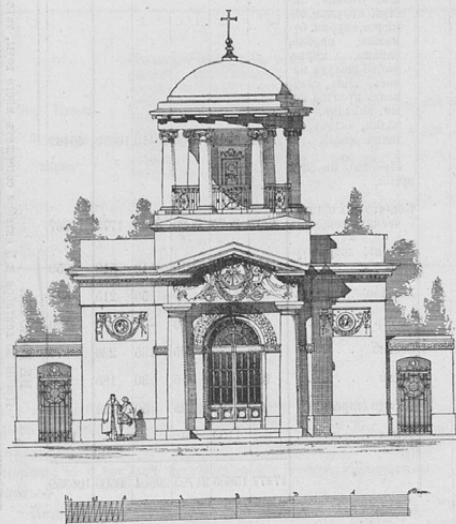
4. Фасады Николаевского дома призрения престарелых и увечных граждан. Журнал Зодчий, выпуск № 22, 1910 г.
