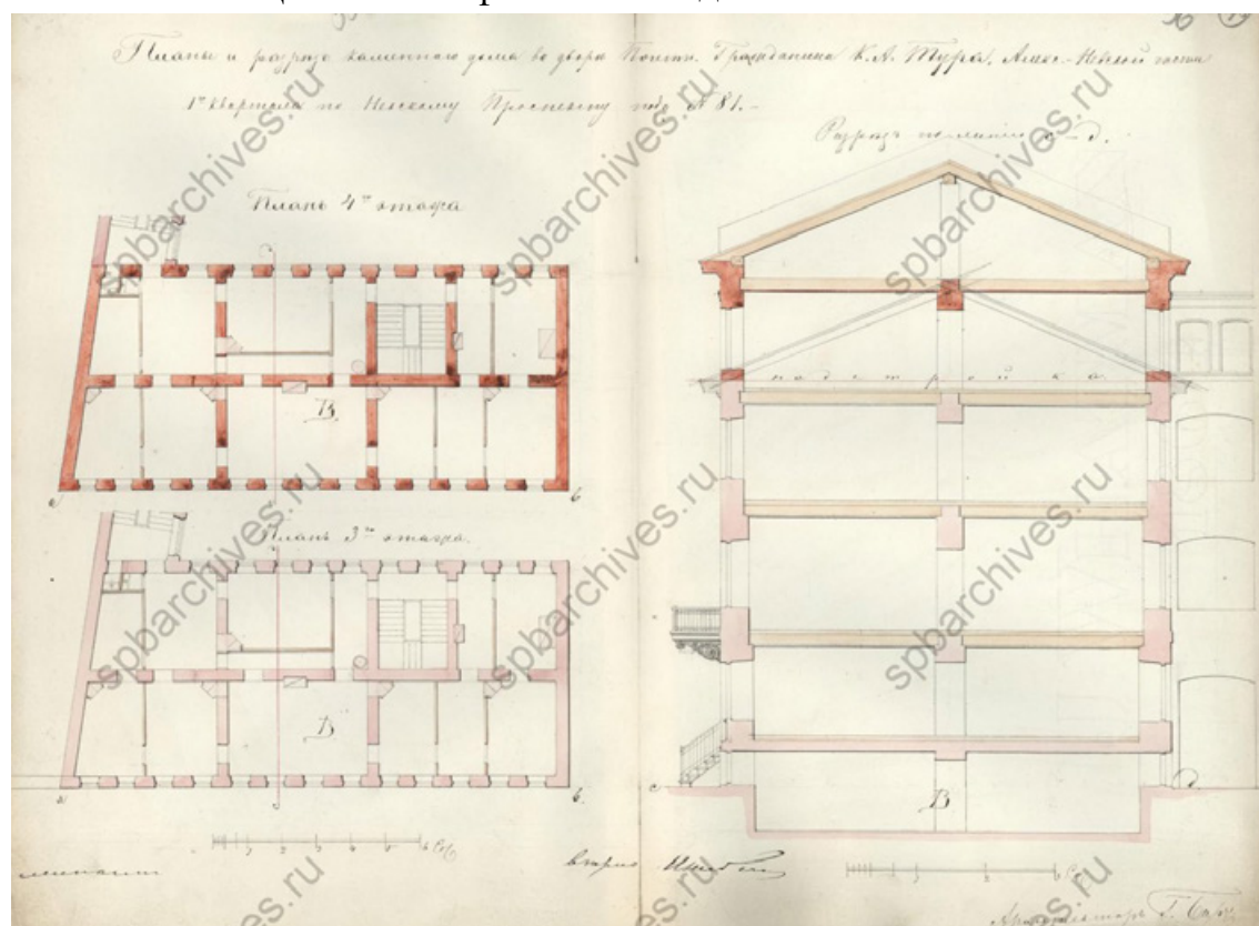
Илл. 40. План и разрез дома во дворе почетного гражданина К.А. Тура. 1867 г. ЦГИА СПб. ф.513 оп.102 д.712. ЛЛ. 55-56.
