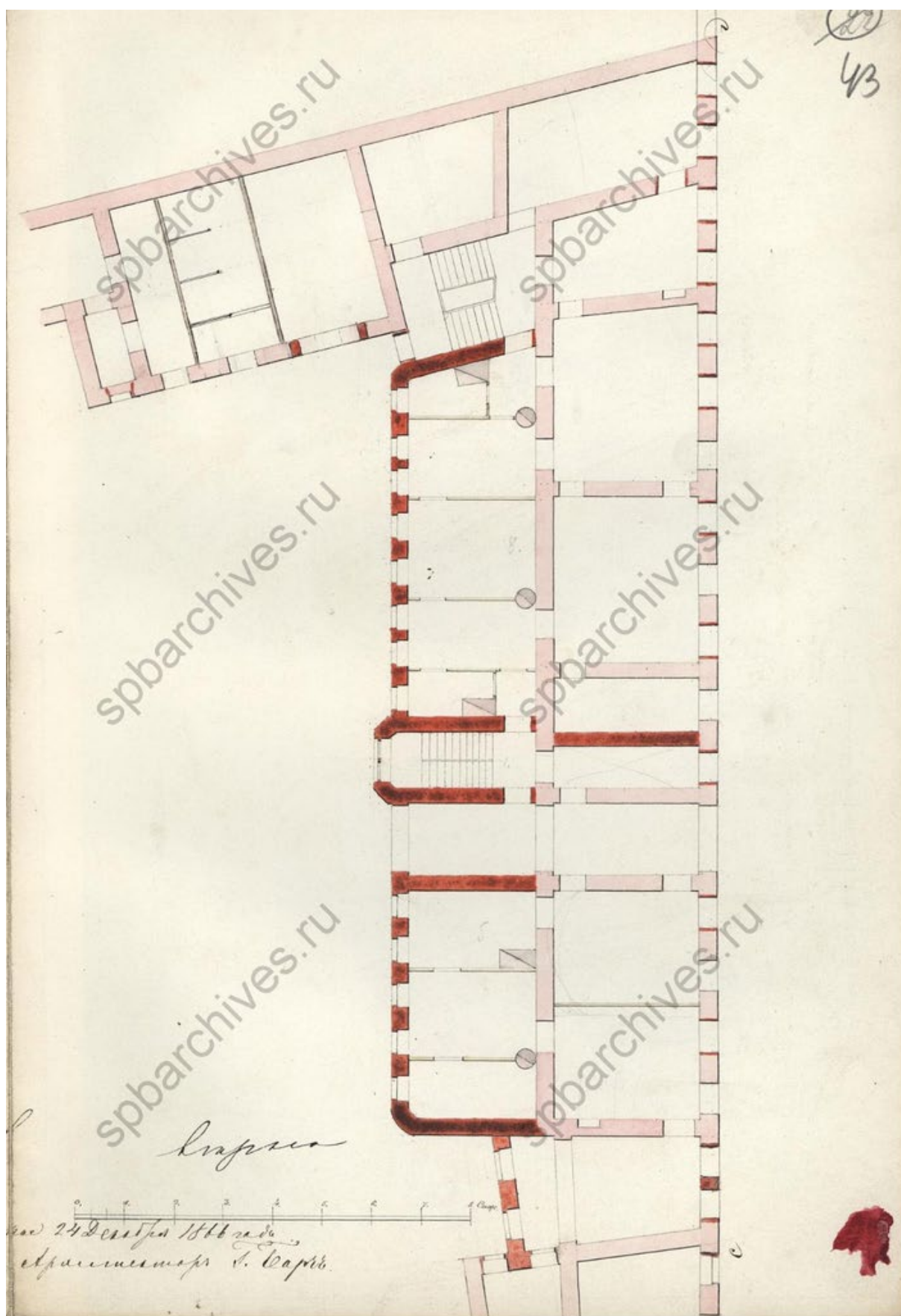
Илл. 33. План. 1867 г. ЦГИА СПб. ф.513 оп.102 д.712. Л. 43.
