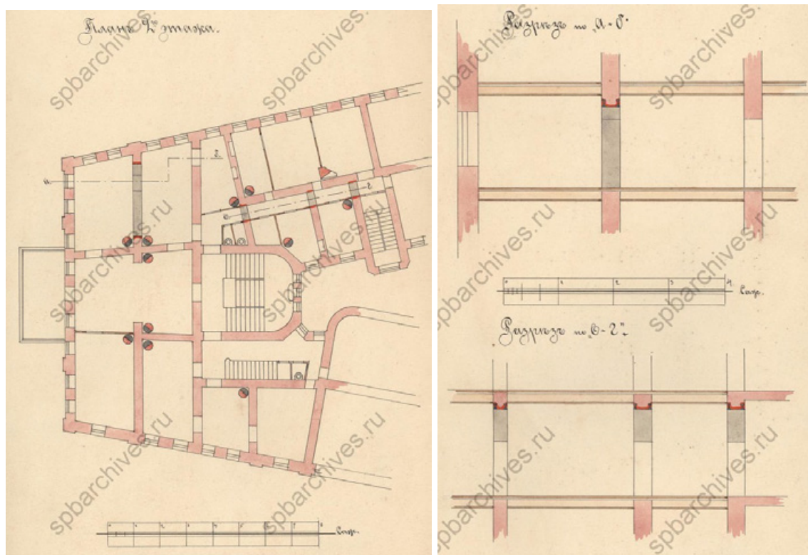
Илл. 59. План 20го эт. Разрез. 1903 г. ЦГИА СПб. ф.513 оп.102 д.712. ЛЛ. 85-86
