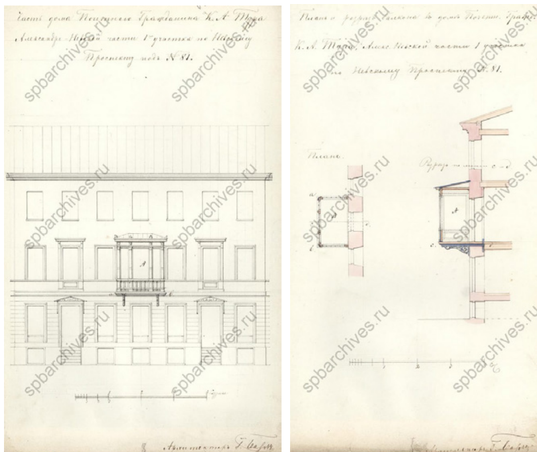
Илл. 53. Часть дома почетного гражданина К.А.Тура. 1867 г. ЦГИА СПб. ф.513 оп.102 д.712. ЛЛ. 76-77.
