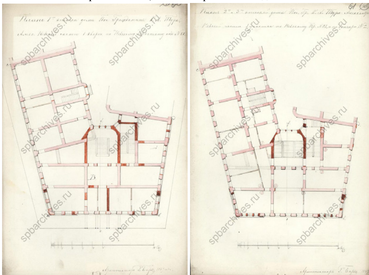
Илл. 43. Планы 1-го, 2-го, 3-го этажей. 1867 г. ЦГИА СПб. ф.513 оп.102 д.712. ЛЛ. 60-61.
