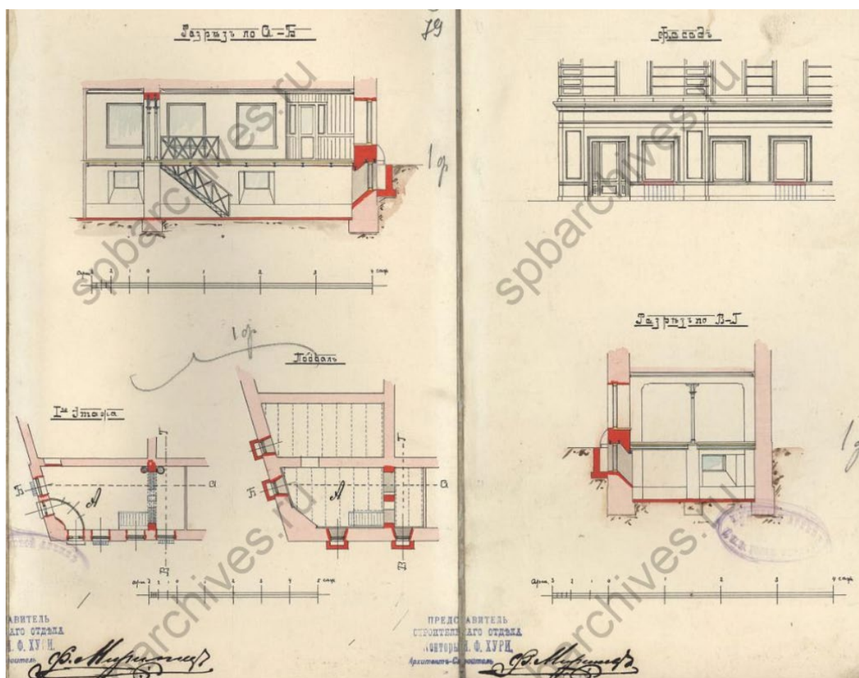
Илл. 55. Разрез, планы, фасады. 1899 г. ЦГИА СПб. ф.513 оп.102 д.712. ЛЛ. 79-80.
