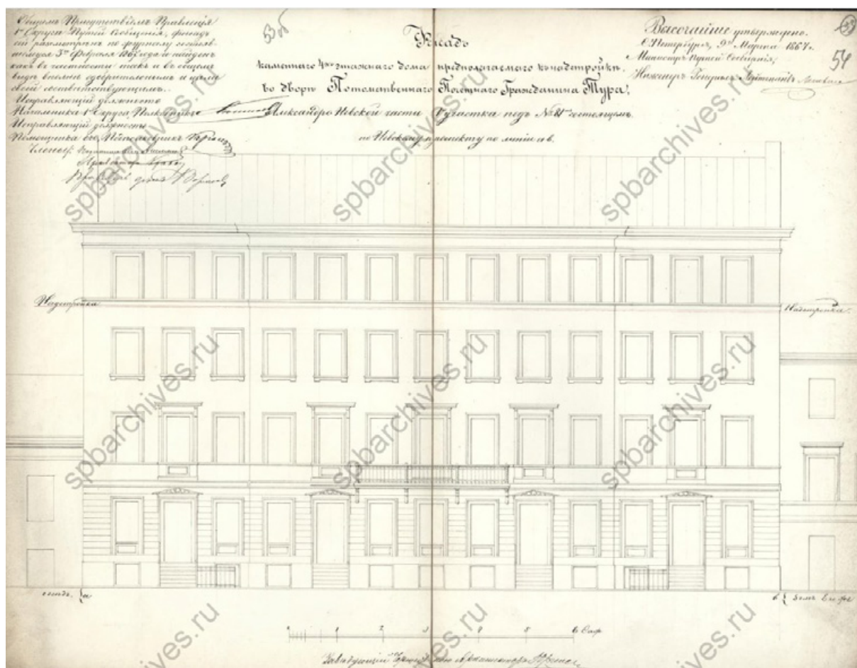
Илл. 39. Фасад дома по Невскому пр. почетного гражданина К.А. Тура 1867 г. ЦГИА СПб. ф.513 оп.102 д.712. ЛЛ. 53об-54.
