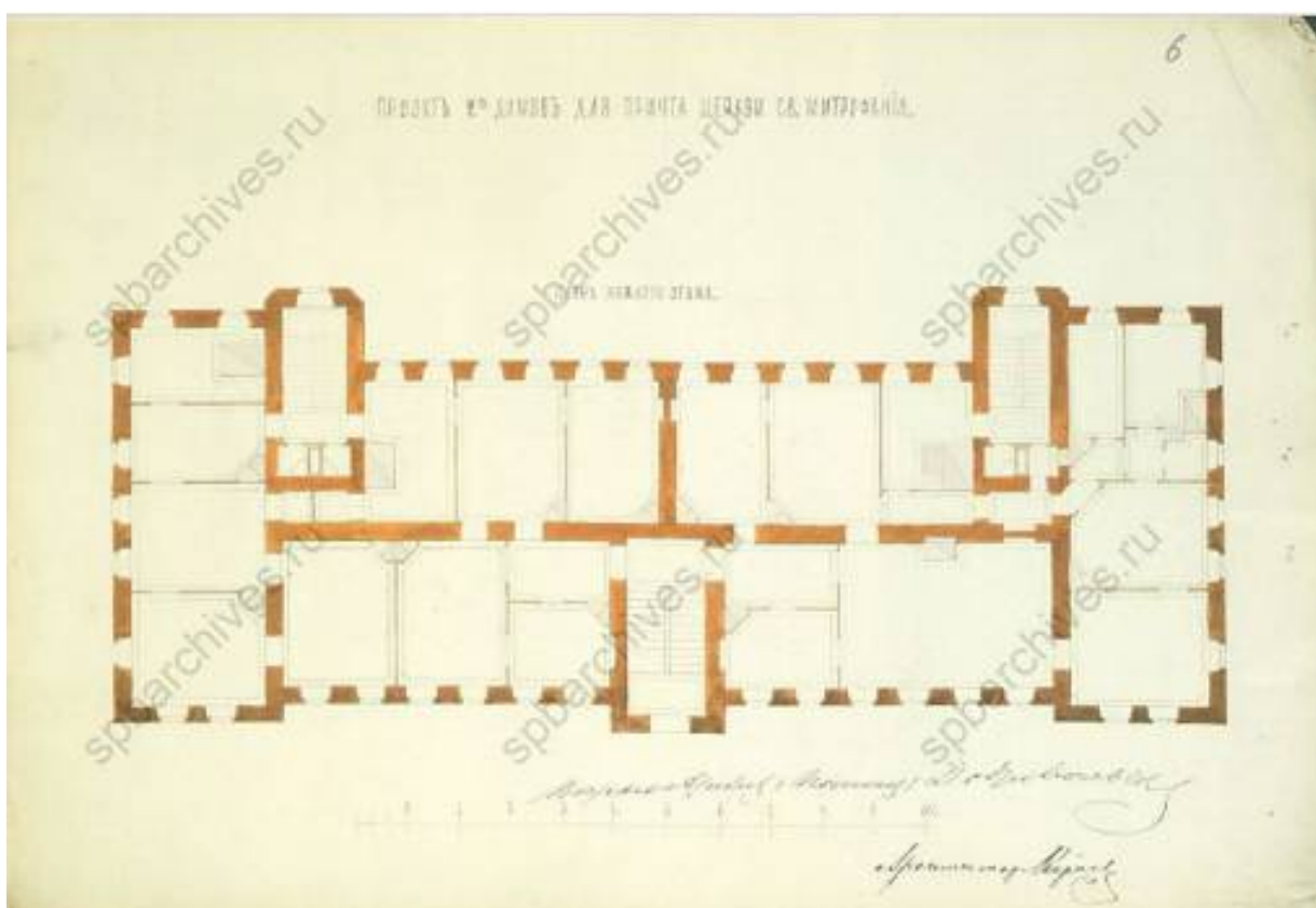
29. Проект двух домов для причта церкви Св. Митрофания. План нижнего этажа. Арх. Г.И. Карпов. 1864 г. ЦГИА СПб. Ф. 513. Оп. 102. Д. 5564. Л. 6.
