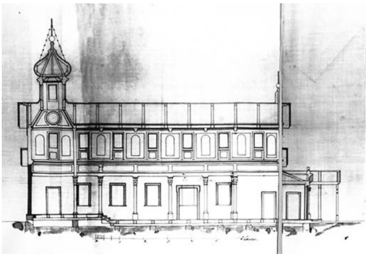
23. Церковь Спаса Всемилоственного (Спасская церковь) на Митрофаниевском православном кладбище. Разрез. 1883 г. ЦГИА СПб. Ф. 513. Оп. 102. Д. 5568. Л. 55-57.
