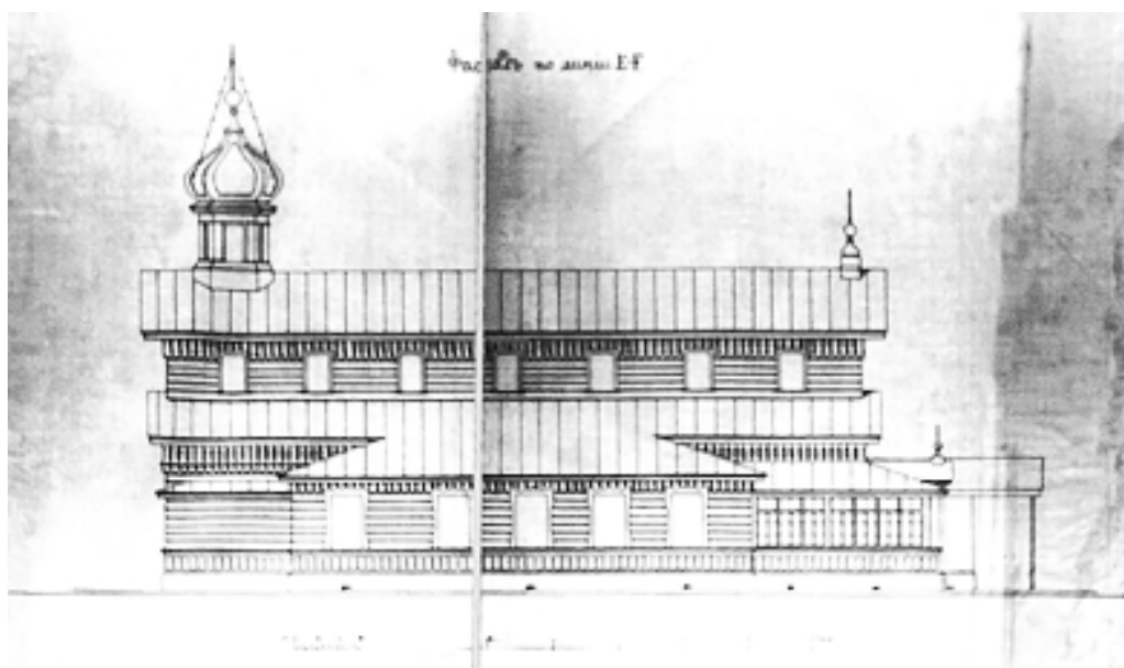
25. Церковь Спаса Всемилоостивого (Спасская церковь) на Митрофаниевском православном кладбище. Фасад по линии Е-Ф. 1883 г. ЦГИА СПб. Ф. 513. Оп. 102. Д. 5568. Л. 52-53.
