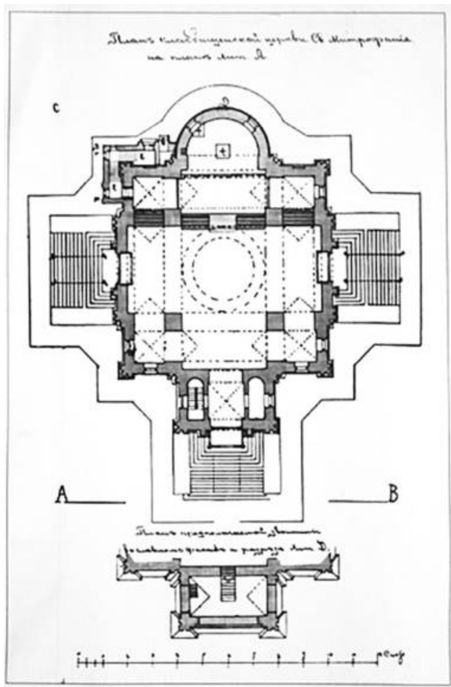
17. Церковь свт. Митрофана Воронежского. План 1883 г. ЦГИА СПб. Ф. 513. Оп. 102. Д. 5568. Л. 45.
