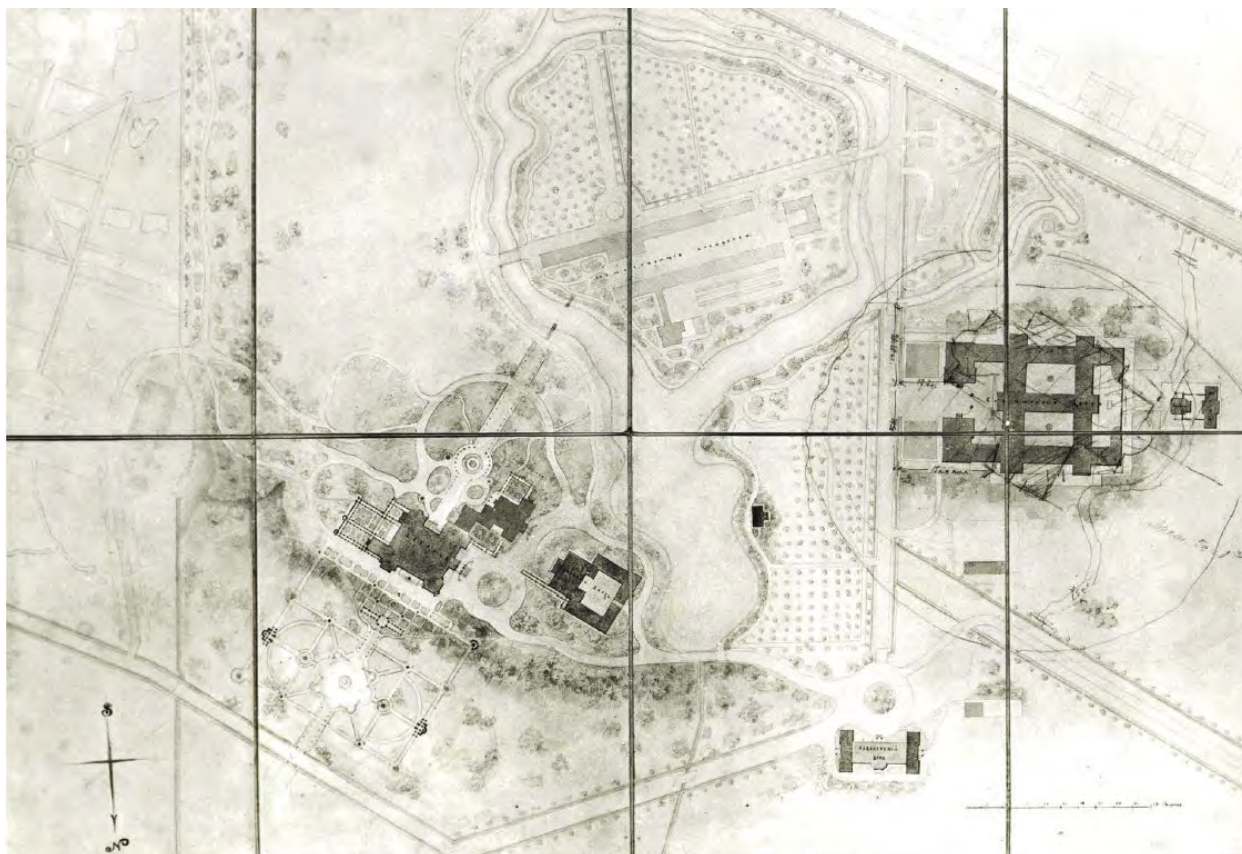
Илл. 27. И.И. Шарлемань. Проект дворца и служб на Михайловской даче. Генеральный план. 1857 г. Источник: НИМ РАХ, А-2947.
