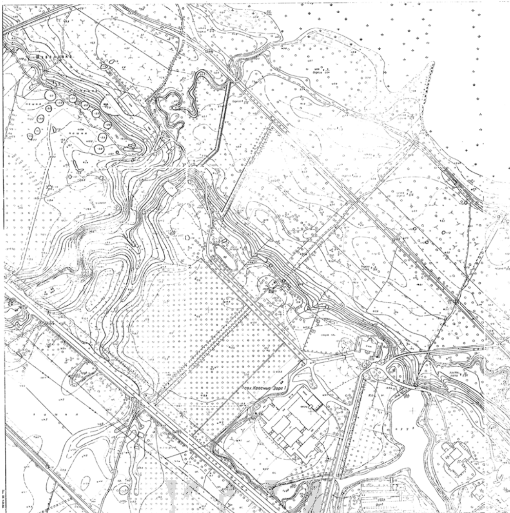
Илл. 33. Михайловская дача. Топоъемка 1965 г. Архив треста ГРИИ.
