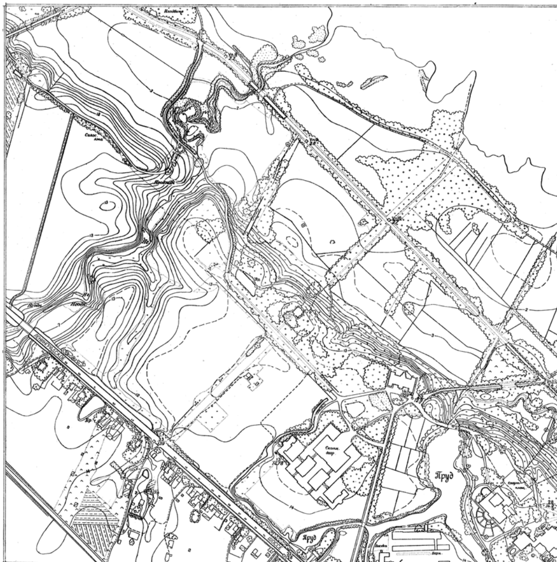
Илл. 31. Михайловская дача. Топоъемка 1935 г. Архив треста ГРИИ.
