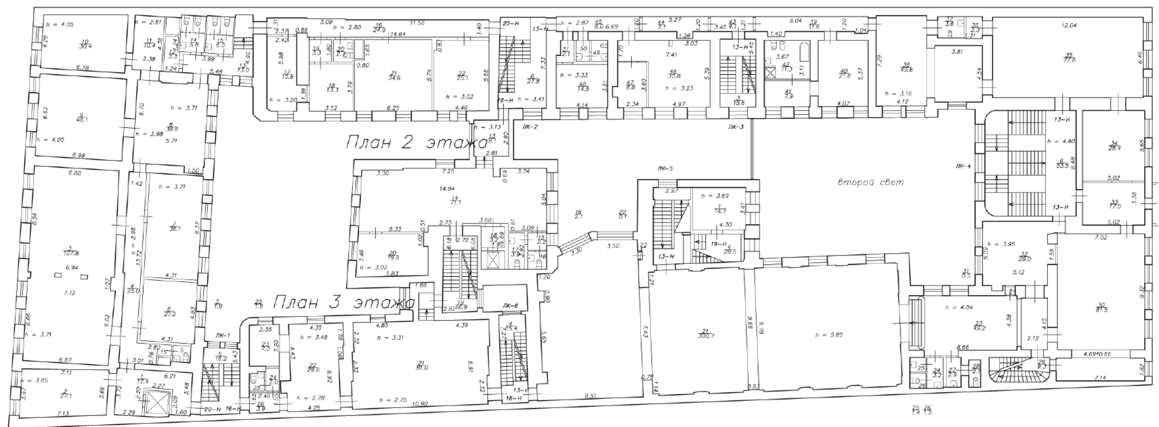
План 2 этажа
