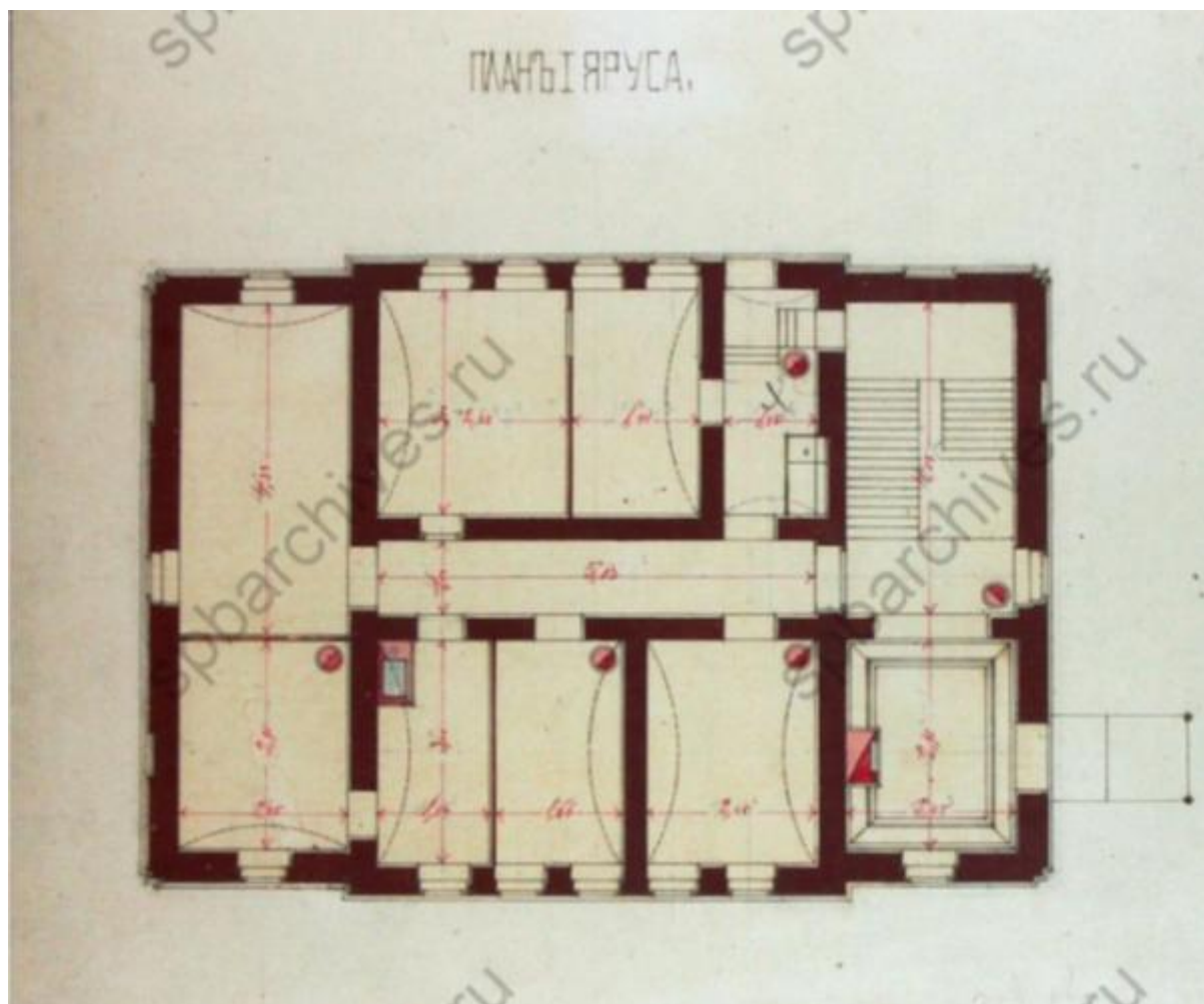
Илл. 15. Проект Общества Правления спасения на водах. Архитектор П. С. Купинский. 1893 г. ЦГИА СПб Ф. 513 Оп. 102 Д.9889. Л. 11-12.
