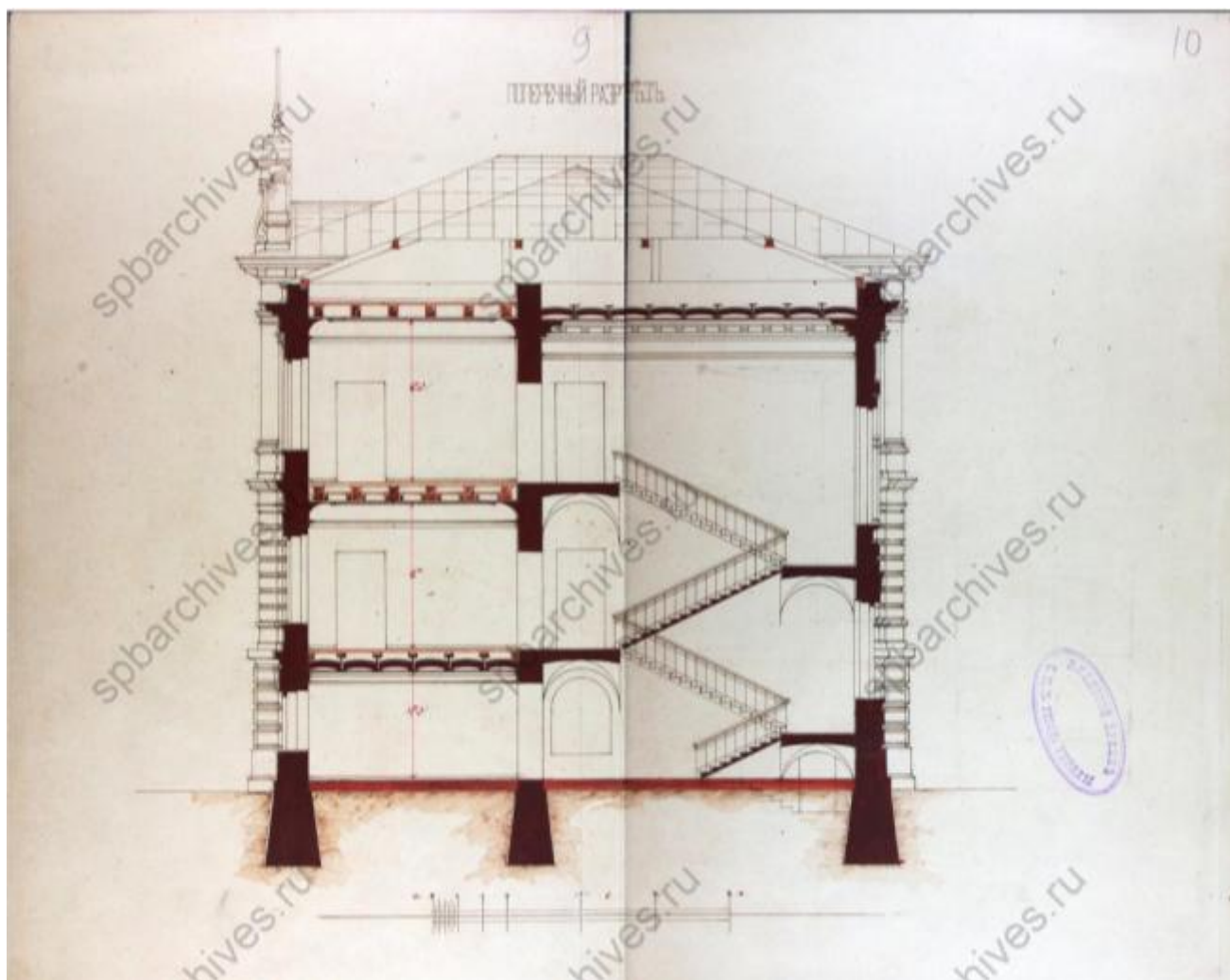
Илл. 14. Проект Общества Правления спасения на водах. Архитектор П. С. Купинский. 1893 г. ЦГИА СПб Ф. 513 Оп. 102 Д.9889. Л. 9-10.
