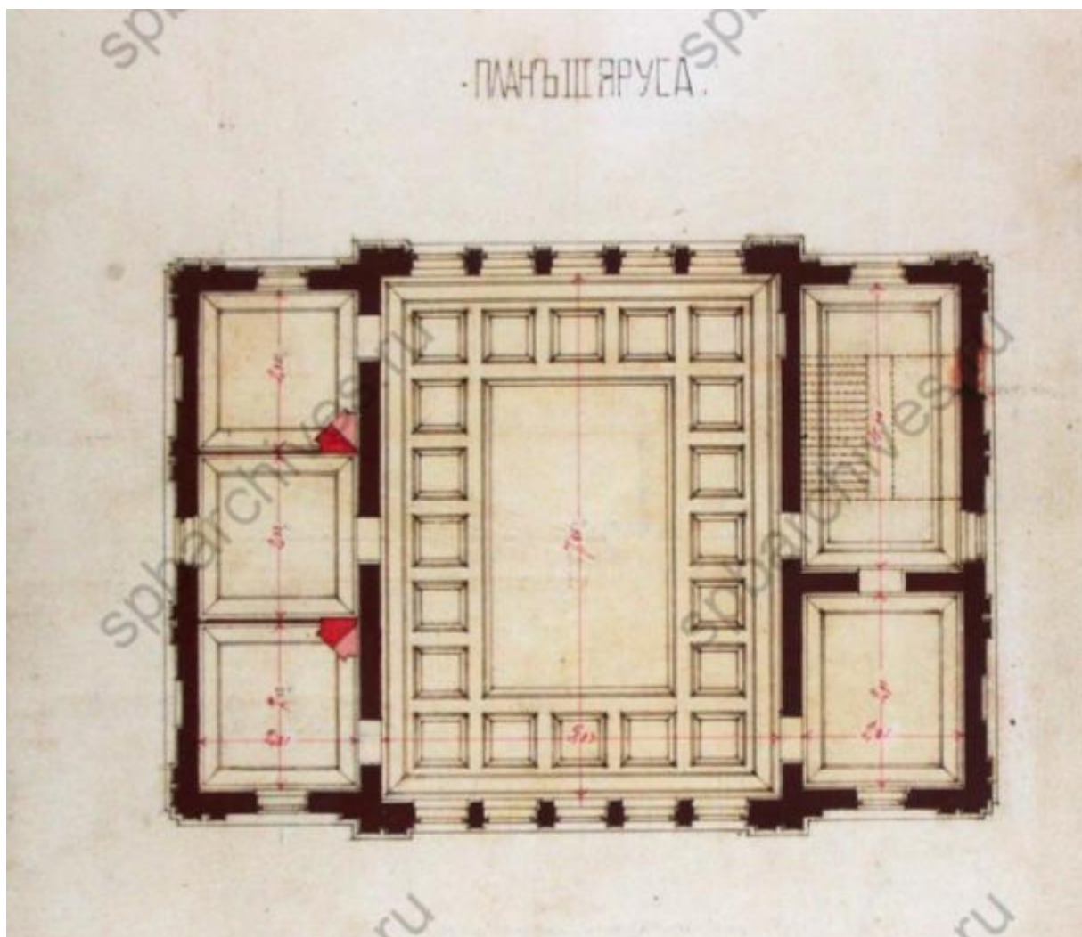
Илл. 17. Проект Общества Правления спасения на водах. Архитектор П. С. Купинский. 1893 г. ЦГИА СПб Ф. 513 Оп. 102 Д.9889. Л. 15-16.
