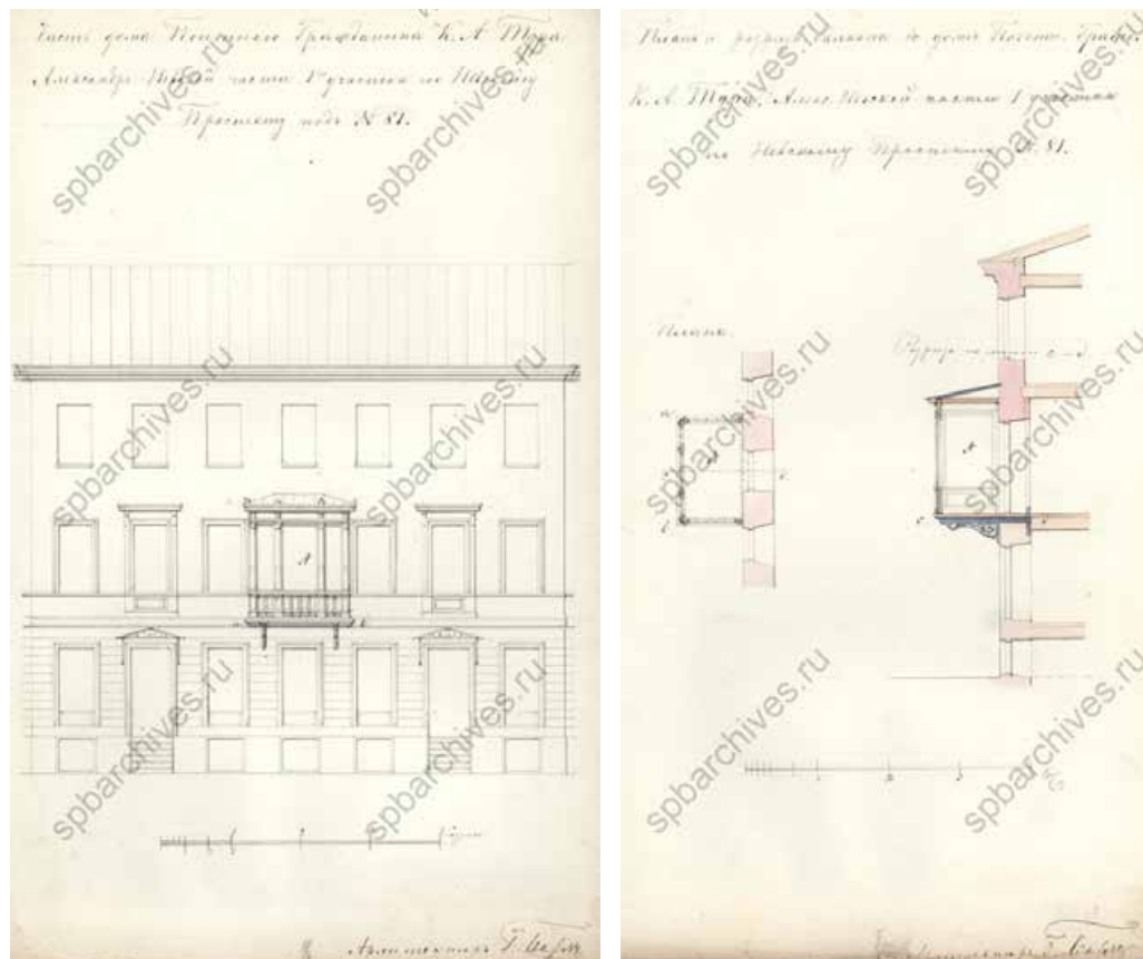
Илл. 53. Часть дома почетного гражданина К.А.Тура. 1867 г. ЦГИА СПб. ф.513 оп.102 д.712. ЛЛ. 76-77.
