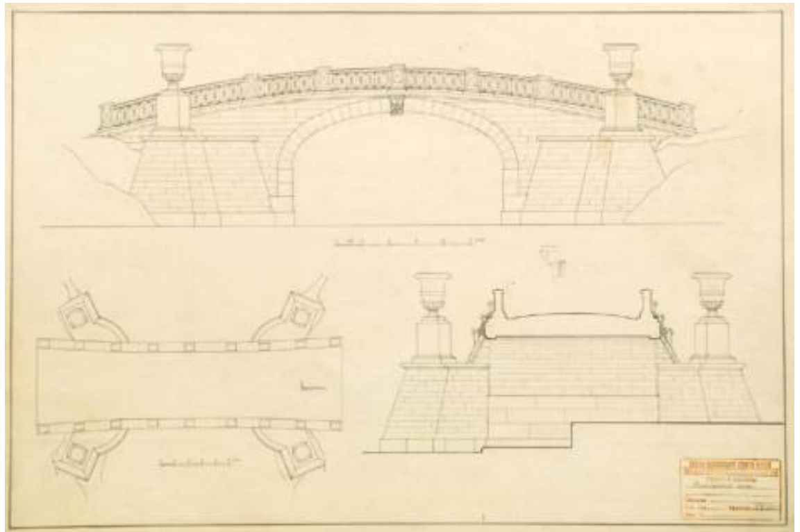
Ил. 35. 1940 г. Архитектор Соколов. Чертеж обмерный (ватман_тушь). Висконтиев мост. О. НВК-691 1.
