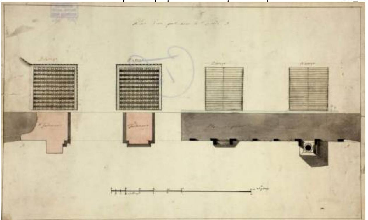
Ил. 19. 1801-1802 гг. Ч-290. Шретер (Shcröter) П.Д.( ). Павловск. Висконтиев мост. План. ПМ КП-42876_1.
