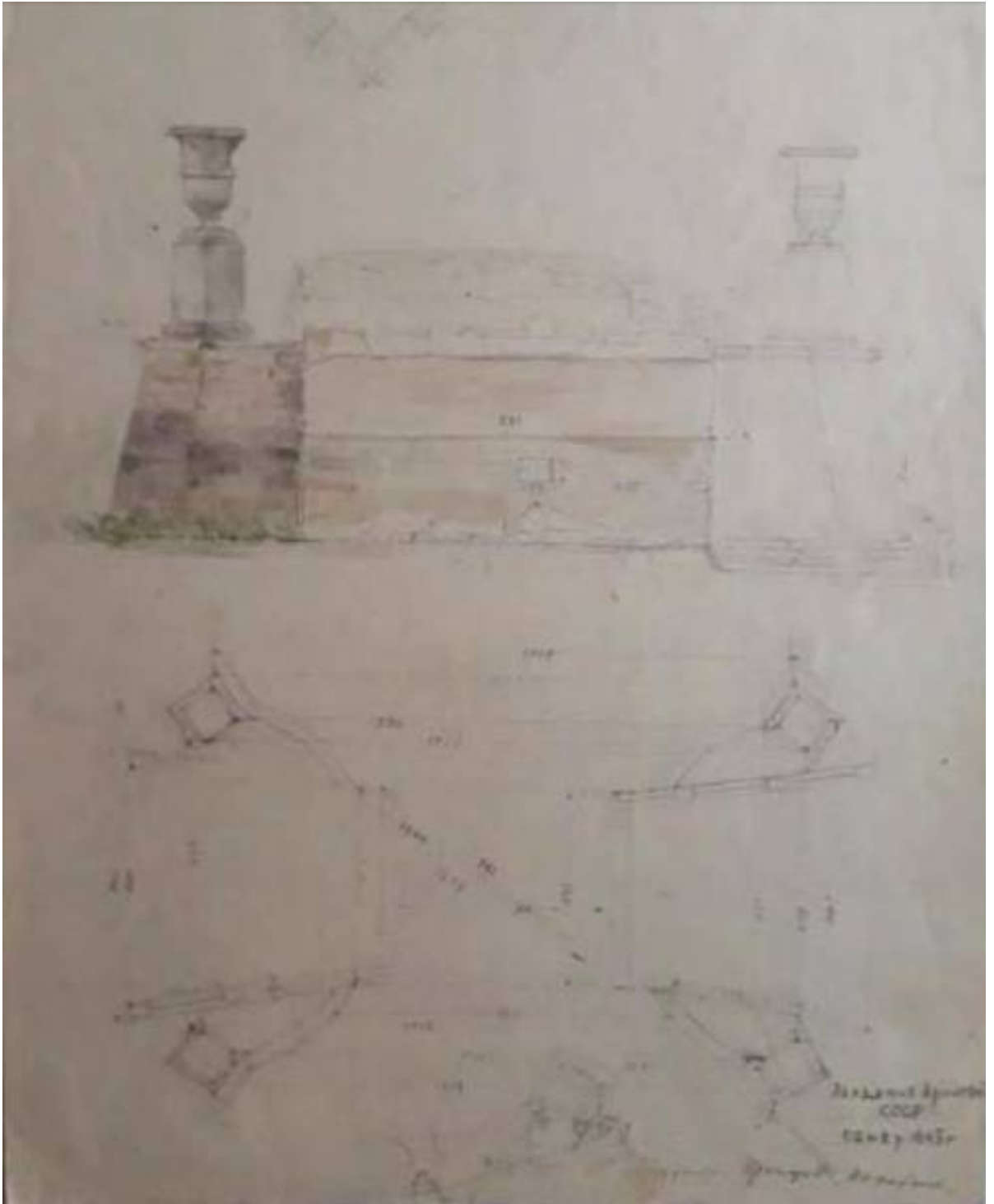
Ил. 37. 1945 г. Обмерный чертёж. Прохоров, Нахабина. Висконтиев мост. Павловский парк 1808 г. Ленинградская обл., г. Павловск. План и фасад. Архитектор: Воронихин А.Н. бумага, карандаш, акварель, 41,5х29,5 см, № ГК 30189520, № КП (ГИК): ГНИМА ОФ-1173/899, Инв. Арх.-391/2, ФГБУК "ГНИ музей архитектуры имени А.В. Щусева".
