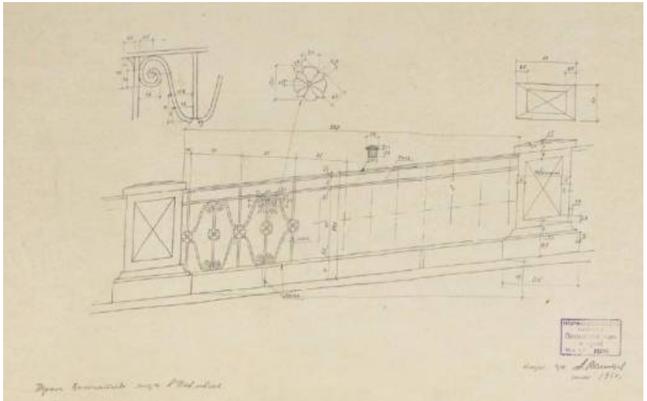
Ил. 38. 1950_Васильев А. Обмерные кроки. Павловский парк. Перила Висконтиева моста. НВК-12174 1.
