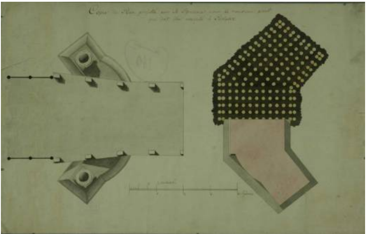
Ил 17. 1801-1802 г. Ч-130. Шретер (Shcröter) П.Д. Павловск. Висконтиев мост. План. ПМ КП-42696_1. Висконтиев мост. План. Копия с чертежа В. Бренны.
