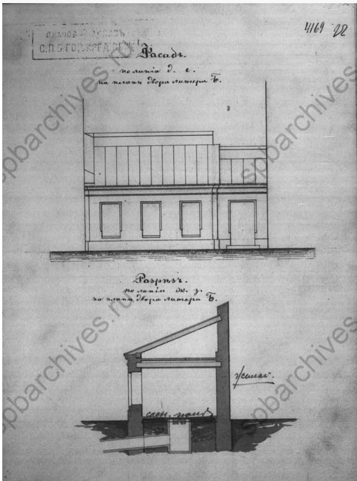
Илл.20. Фасад и разрез исследуемого здания. Фиксационный чертеж. [1878 – 1894гг.]. ЦГИА СПб. Ф. 515. Оп. 4. Д. 2705. Л. 22.
