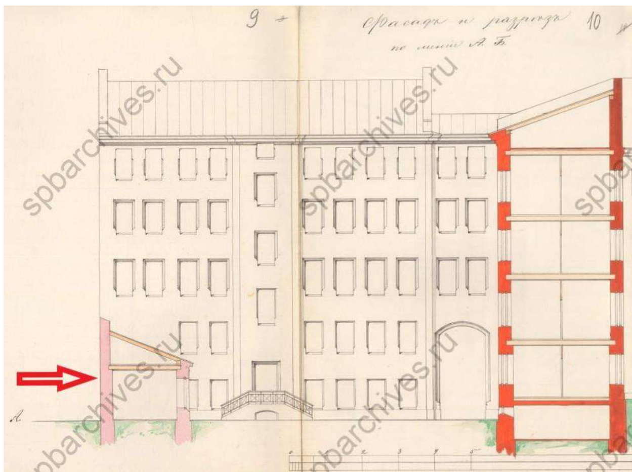
Илл.11. Разрез исследуемого здания (обозначено красной стрелкой) на проектном чертеже 1877 г. ЦГИА СПб. Ф. 513. Оп. 102. Д. 1549. Л. 9 — 10.
