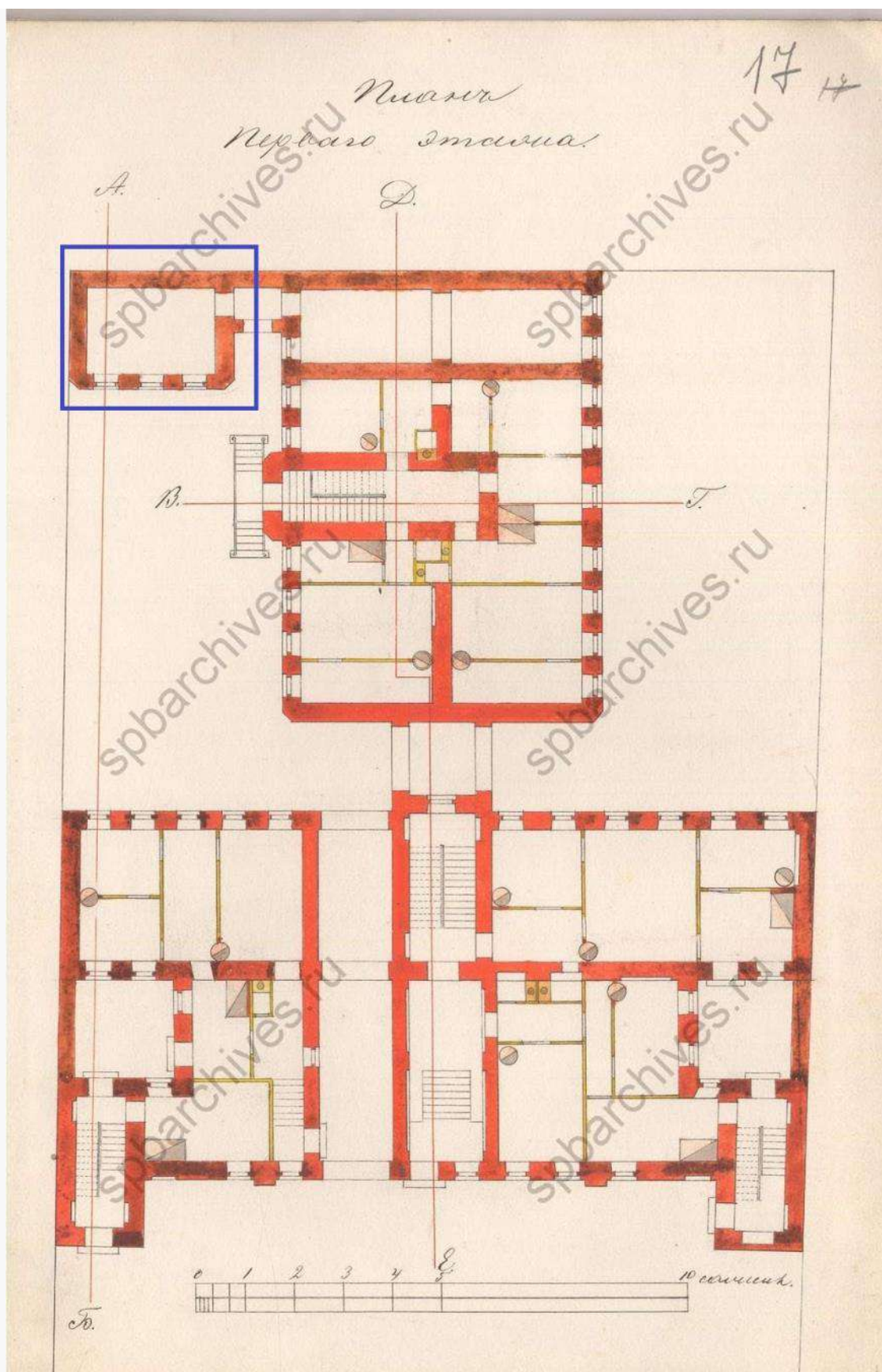
Илл.13. План первого этажа исследуемого здания (выделено рамкой) на проектом чертеже 1877 г. ЦГИА СПб. Ф. 513. Оп. 102. Д. 1549. Л. 17.
