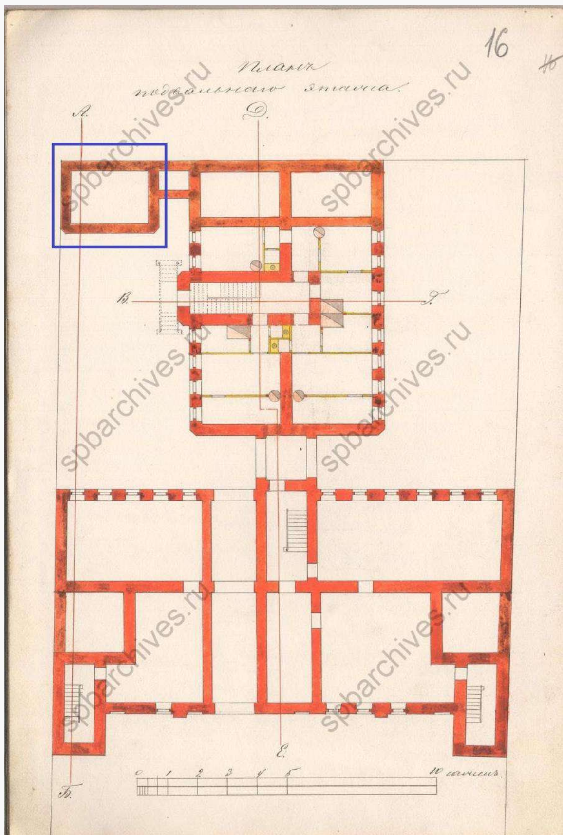
Илл.12. План подвального этажа исследуемого здания (выделено синей рамкой) на проектном чертеже 1877 г. ЦГИА СПб. Ф. 513. Оп. 102. Д. 1549. Л. 16.
