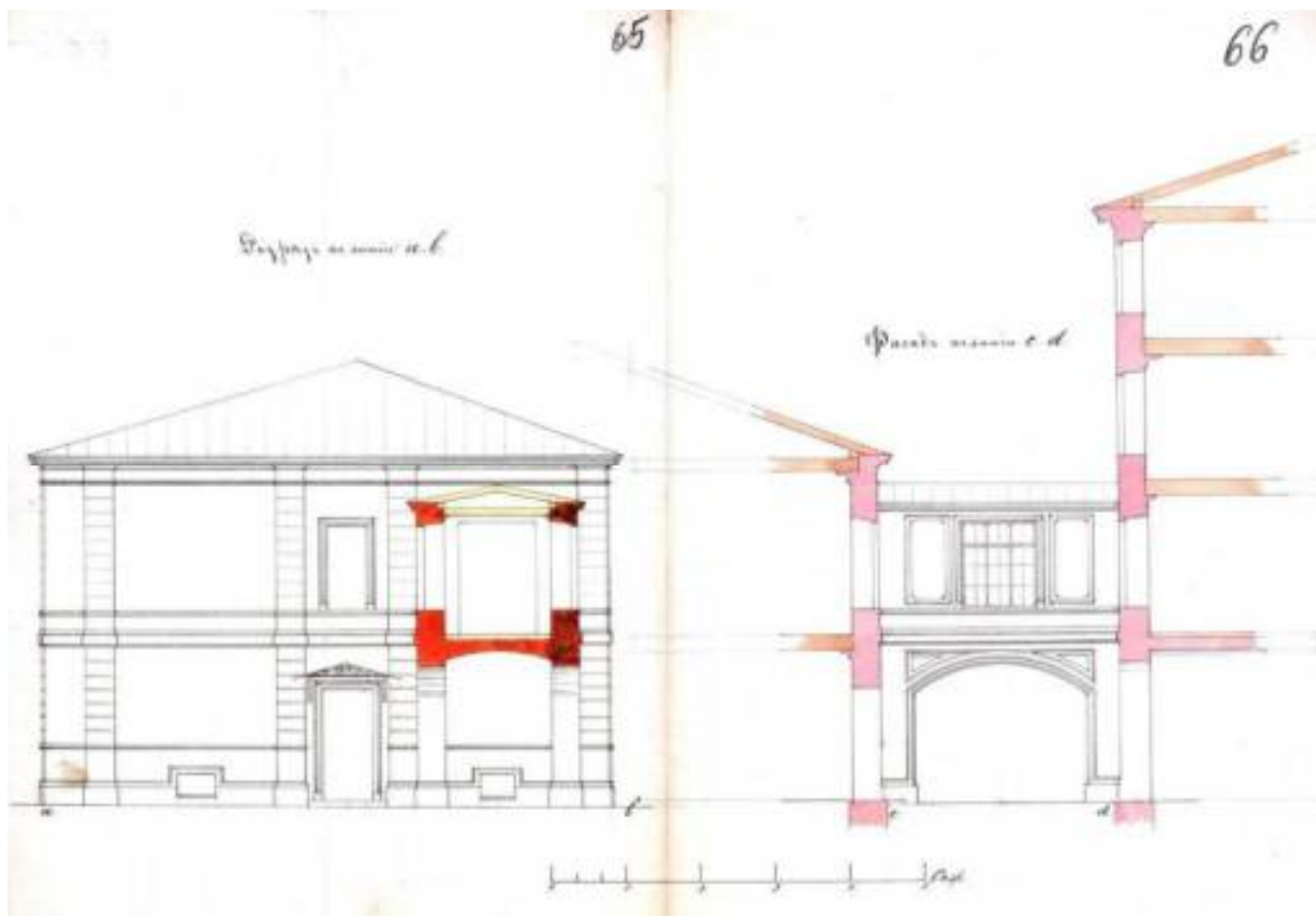
Илл.23. Разрез по линии а-в, фасад по линии с-д. 1882 г. ЦГИА СПб. Фонд 513. Опись 102. Дело 4682. Л.65-66.
