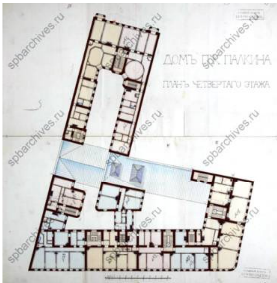
Илл.61. План 4-го этажа. 1910 г. ЦГИА СПб. Фонд 515. Описание 4. Дело 3709. Л.37-42.
