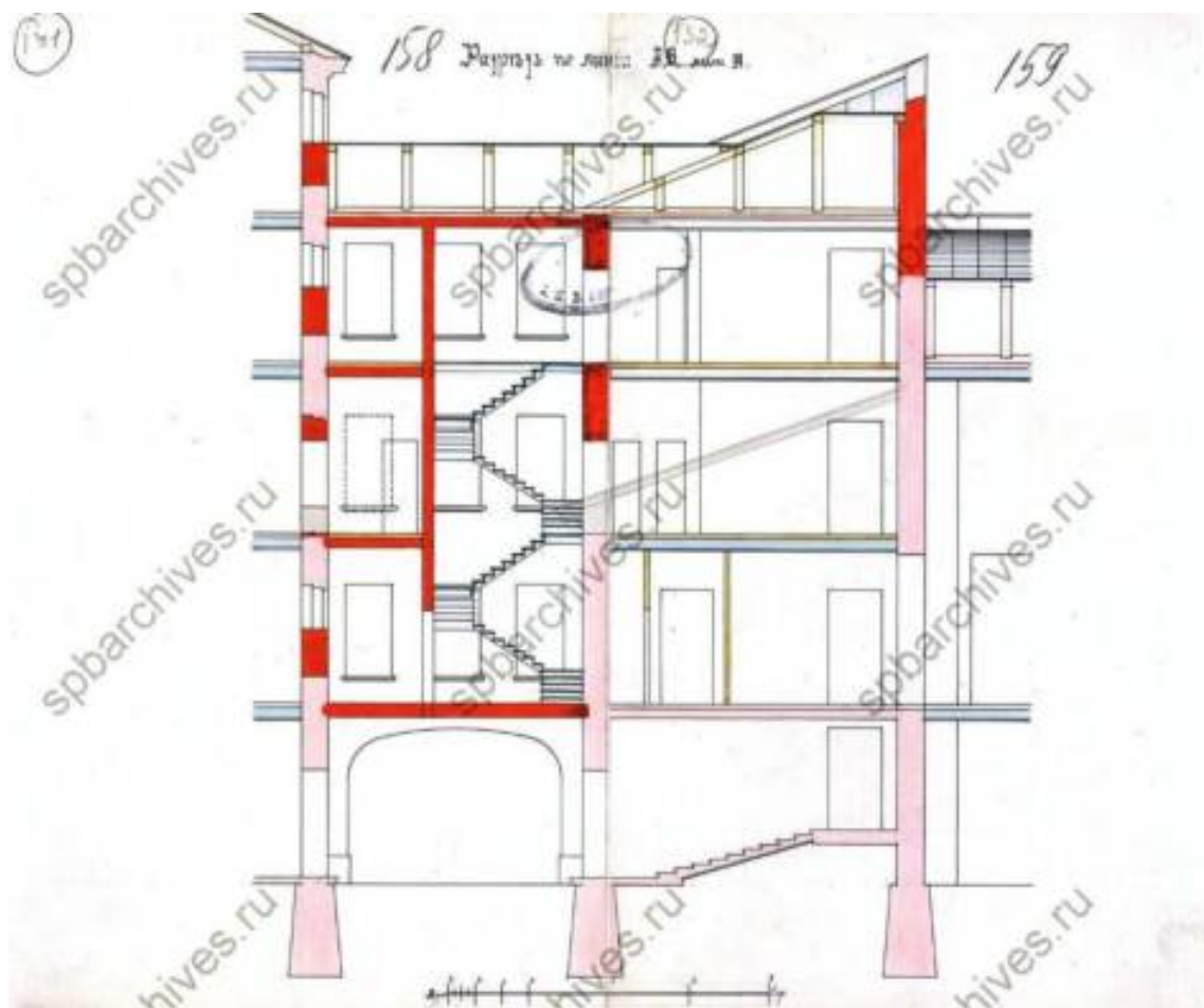
Илл.48. Разрез по линии А-В. 1904 г. ЦГИА СПб. Фонд 513. Опись 102. Дело 4682. Л.158-159.
