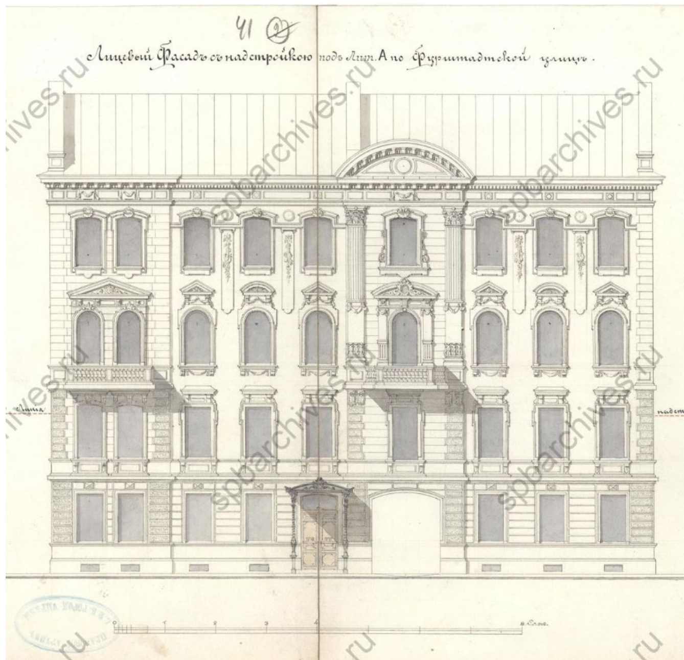
22. 1892. Лицевой фасад с надстройкою под лит А по Фурштадтской улице. ЦГИА СПб Ф. 513. Оп. 102. Д. 4526. Л. 41-42. Красным пунктиром показана линия надстройки, проходящая в верхней четверти окон второго этажа.
