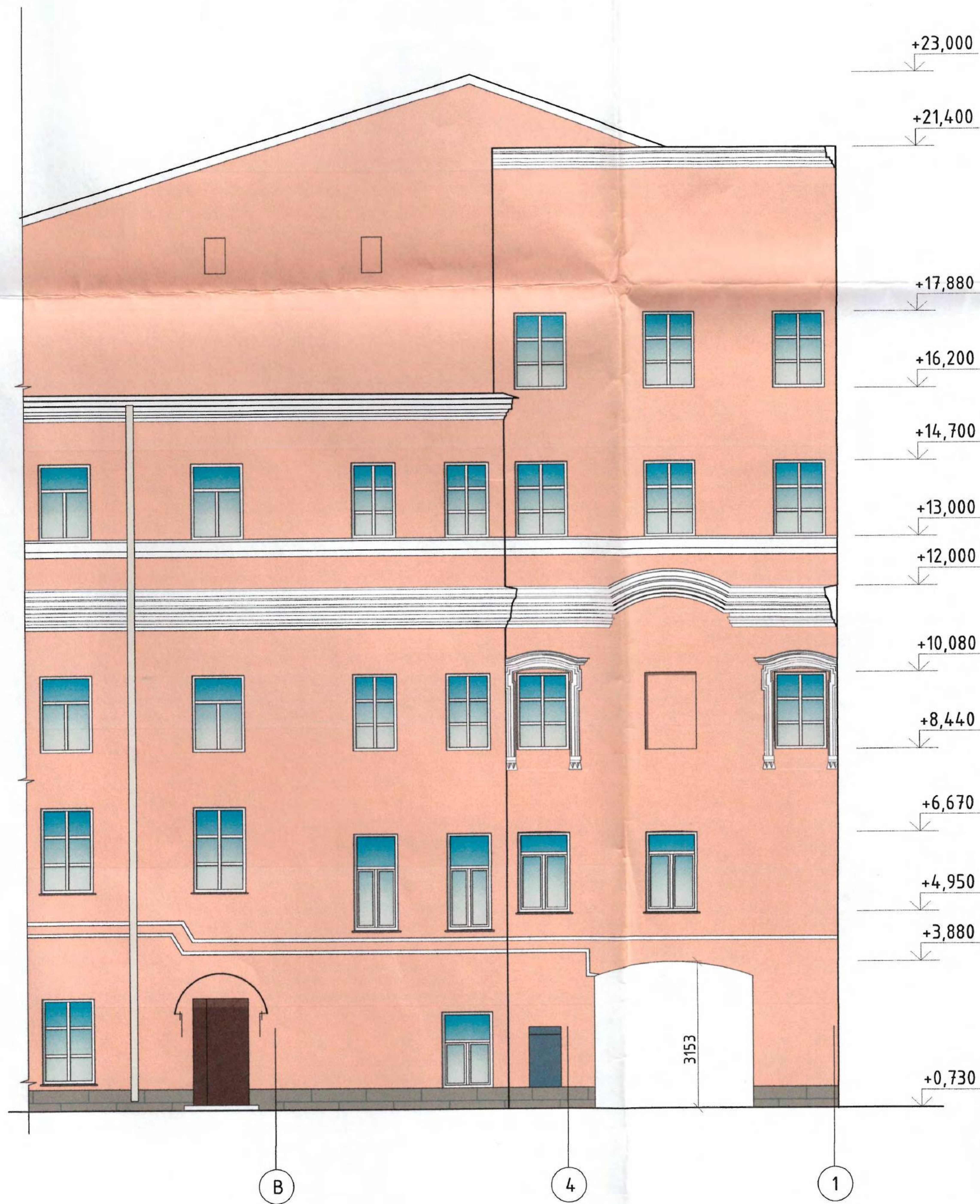
Фасад В-1 до благоустройства М 1:100
