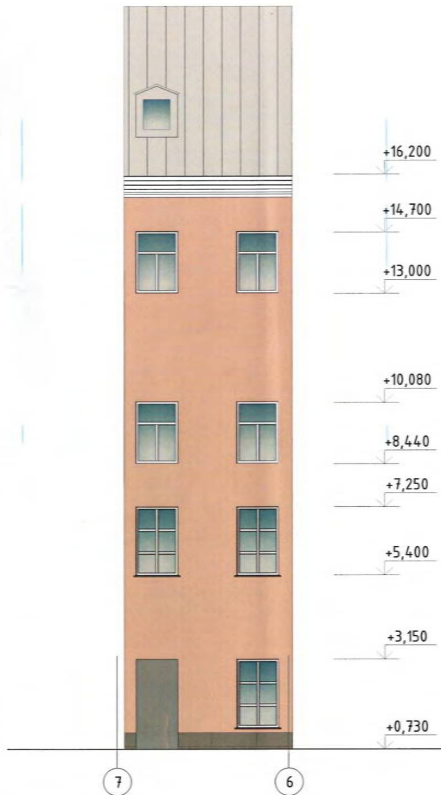
Фасад 7-8 до благоустройства М 1:100
