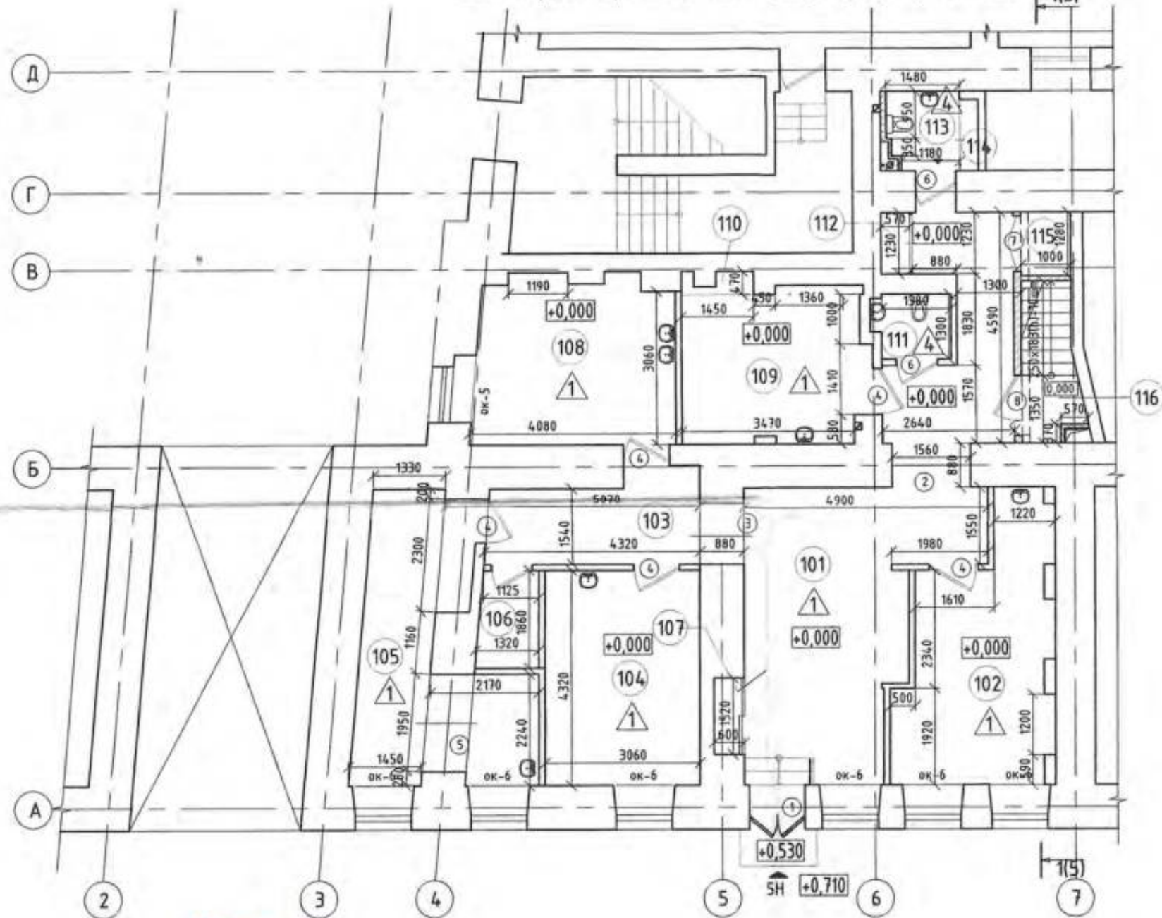
План перепланировки на отм. +2,960, +3,080, +3,680 М 1:100 1(5)
