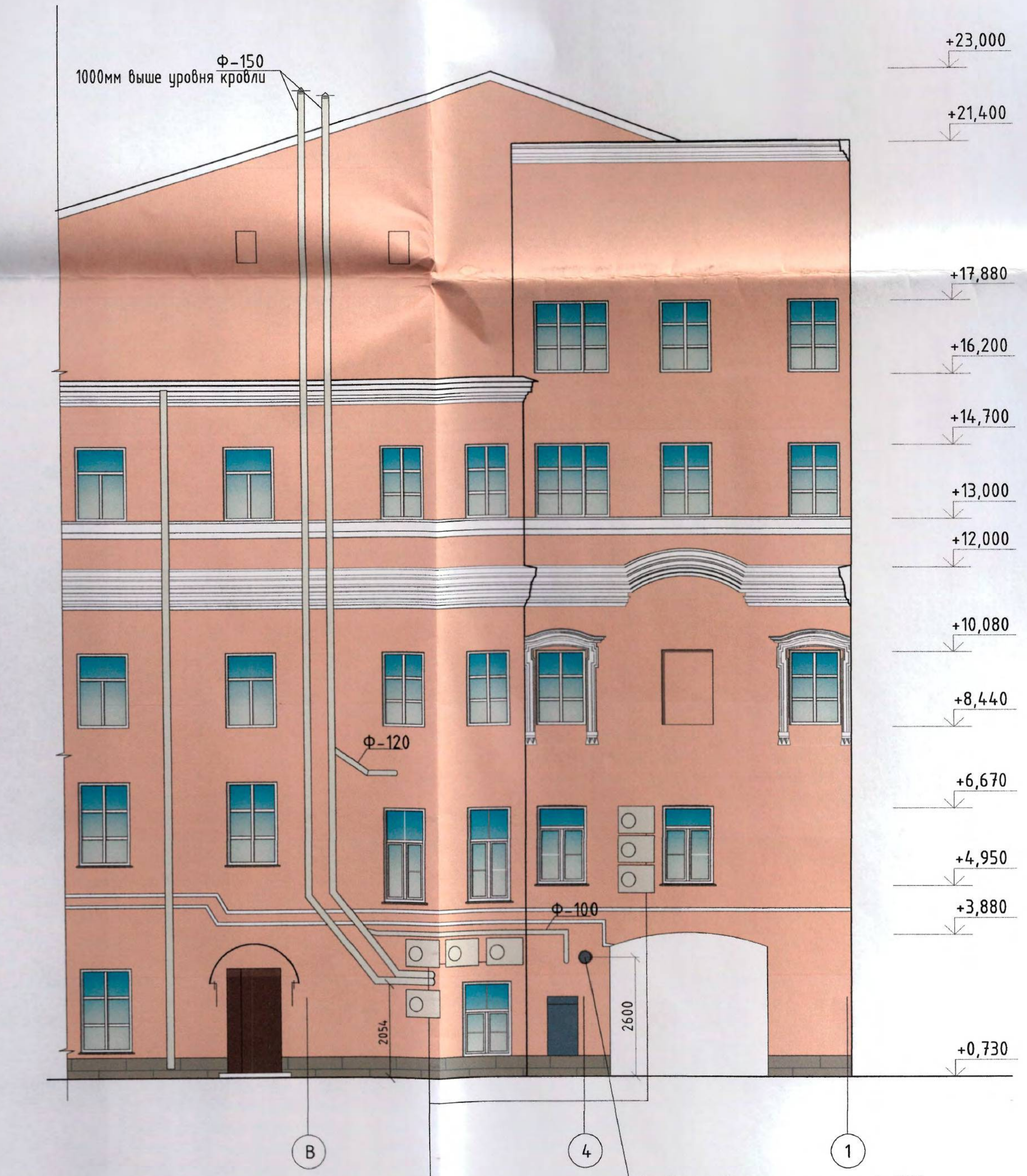
Фасад В-1 после благоустройства М 1:100
