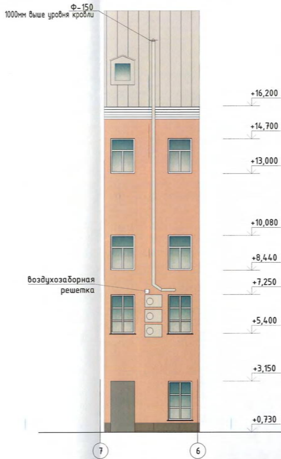
Фасад 7-8 после благоустройства М 1:100
