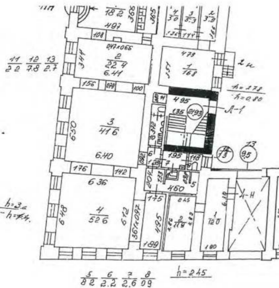
План части цокольного этажа
