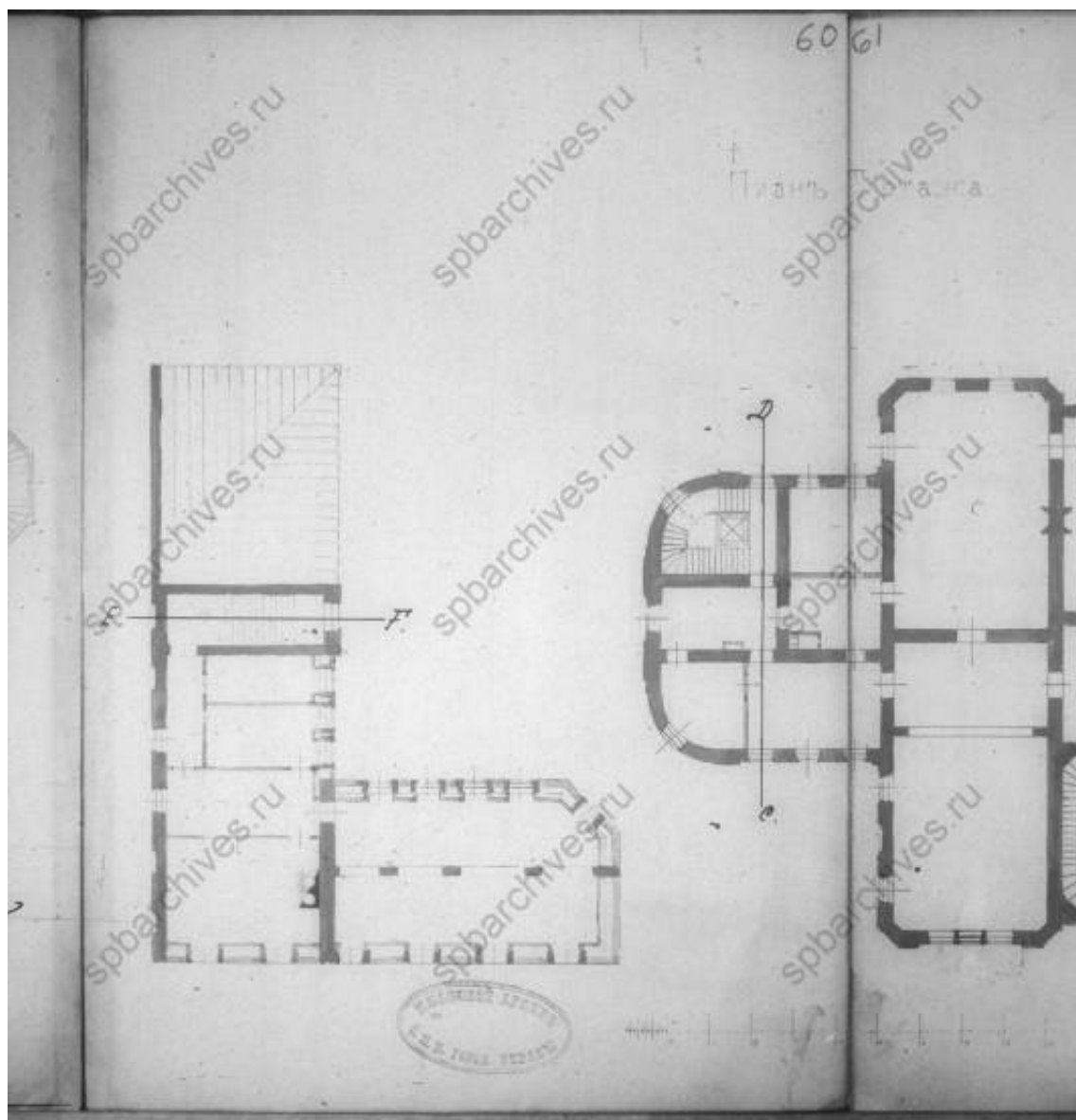
7. Чертежи дома на участке, принадлежавшем Шорохову, А.Н.Колупаевой, Клементьевой, Ф.Ф.Отто, А.К.Отто, В.А.Слепцову, А.С.Слепцовой, кн. К.А.Горчакову по Малой Монетной ул., 10, 12, 14 и Большой Монетной ул., 11. 1832–1908 гг. ЦГИА СПб ф.513 оп.102 д.8141. Л. 60
