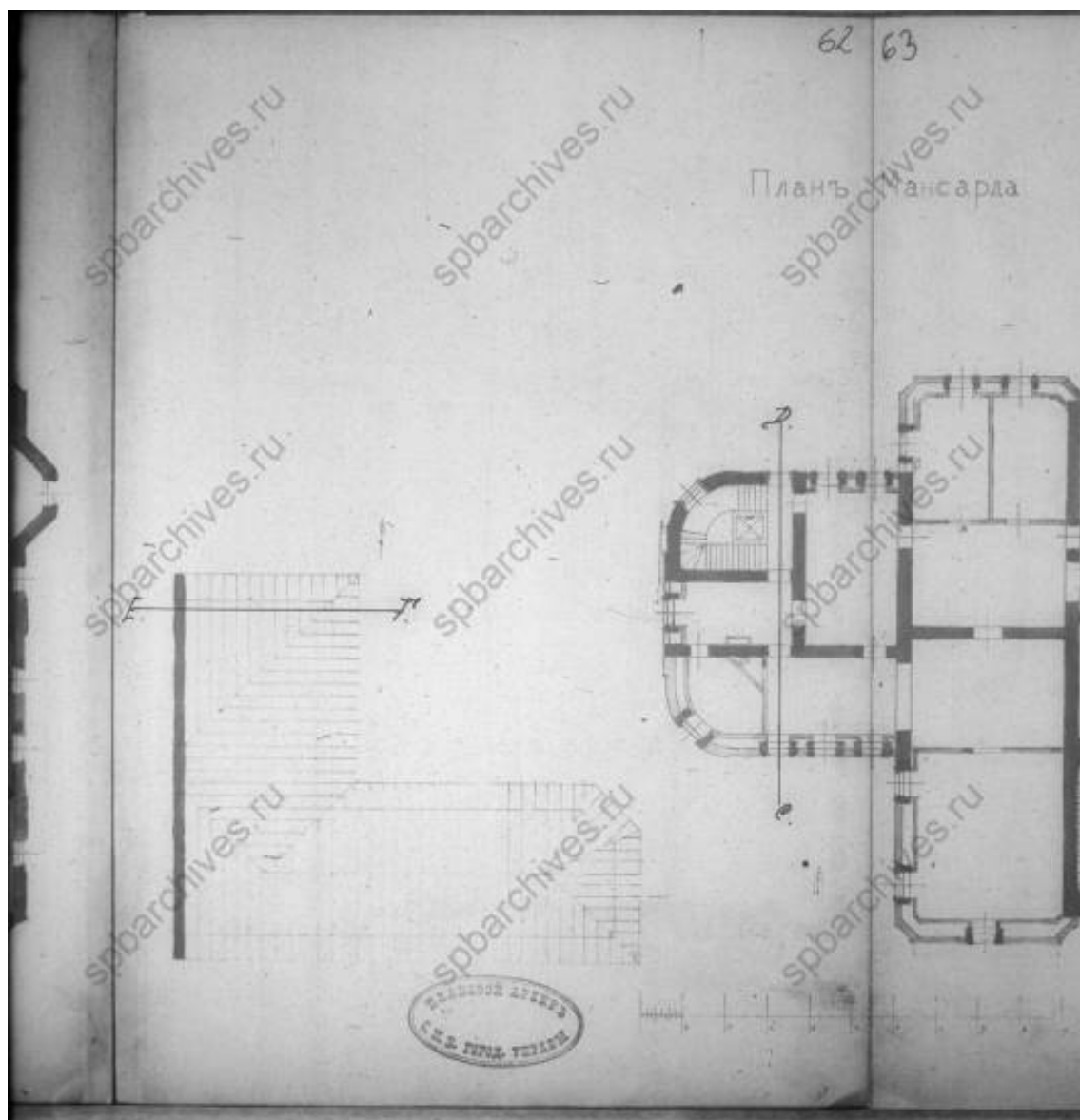
8. Чертежи дома на участке, принадлежавшем Шорохову, А.Н. Колупаевой, Клементьевой, Ф.Ф.Отто, А.К.Отто, В.А.Слепцову, А.С.Слепцовой, кн. К.А.Горчакову по Малой Монетной ул., 10, 12, 14 и Большой Монетной ул., 11. 1832–1908 гг. ЦГИА СПб ф.513 оп.102 д.8141. Л. 62
