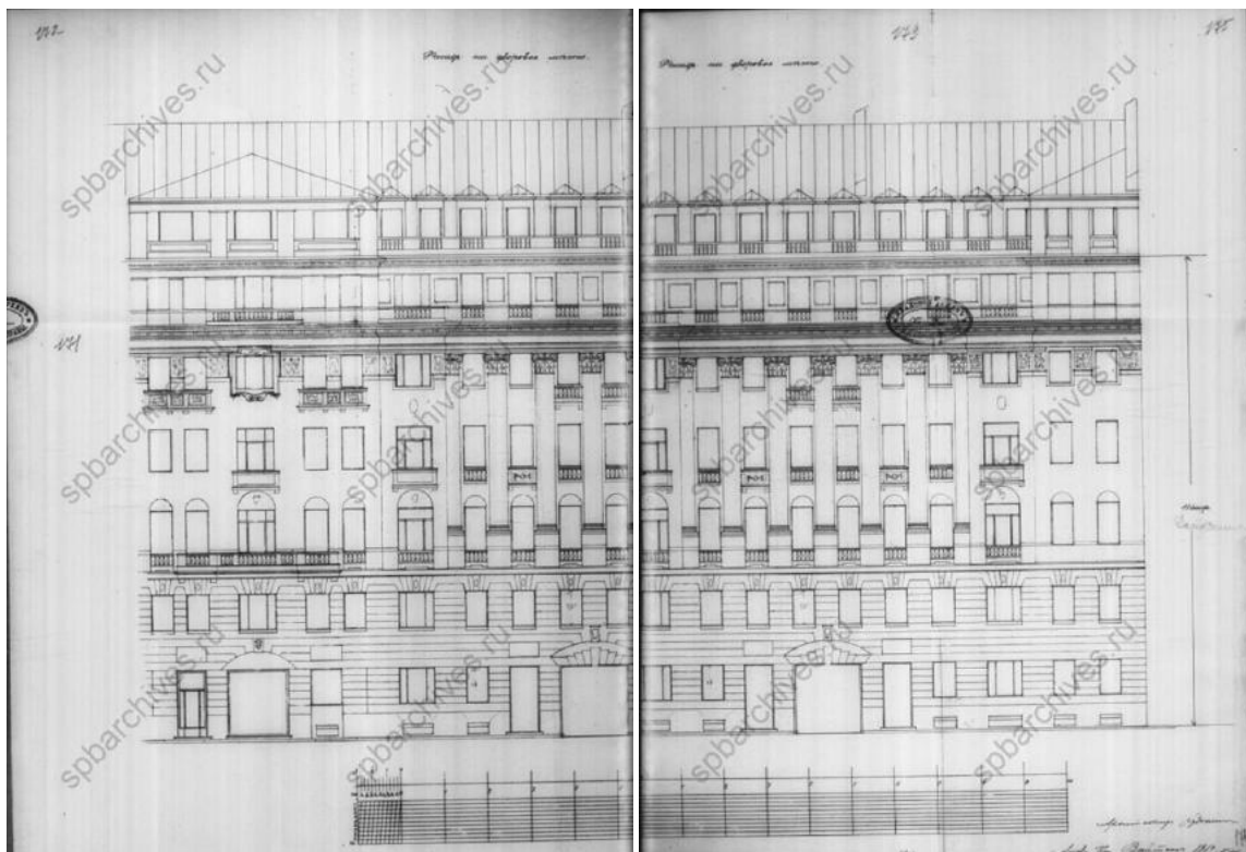
14. Проект постройки 6-этажного дома. Торцевой фасад. Арх. А.П. Вайтенс. 1914 год. // ЦГИА СПб. Ф.513. Оп. 102. Д. 7783. ЛЛ. 172-176.
