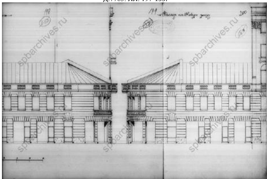
17. Проект постройки 2-этажного корпуса по Каменноостровскому проспекту. (изменение проекта 1914 года). Арх. А.П. Вайтенс. План. Северный фасад. 1916 год. // ЦГИА СПб. Ф. 513. Оп. 102. Д.7783. ЛЛ. 198-200.
