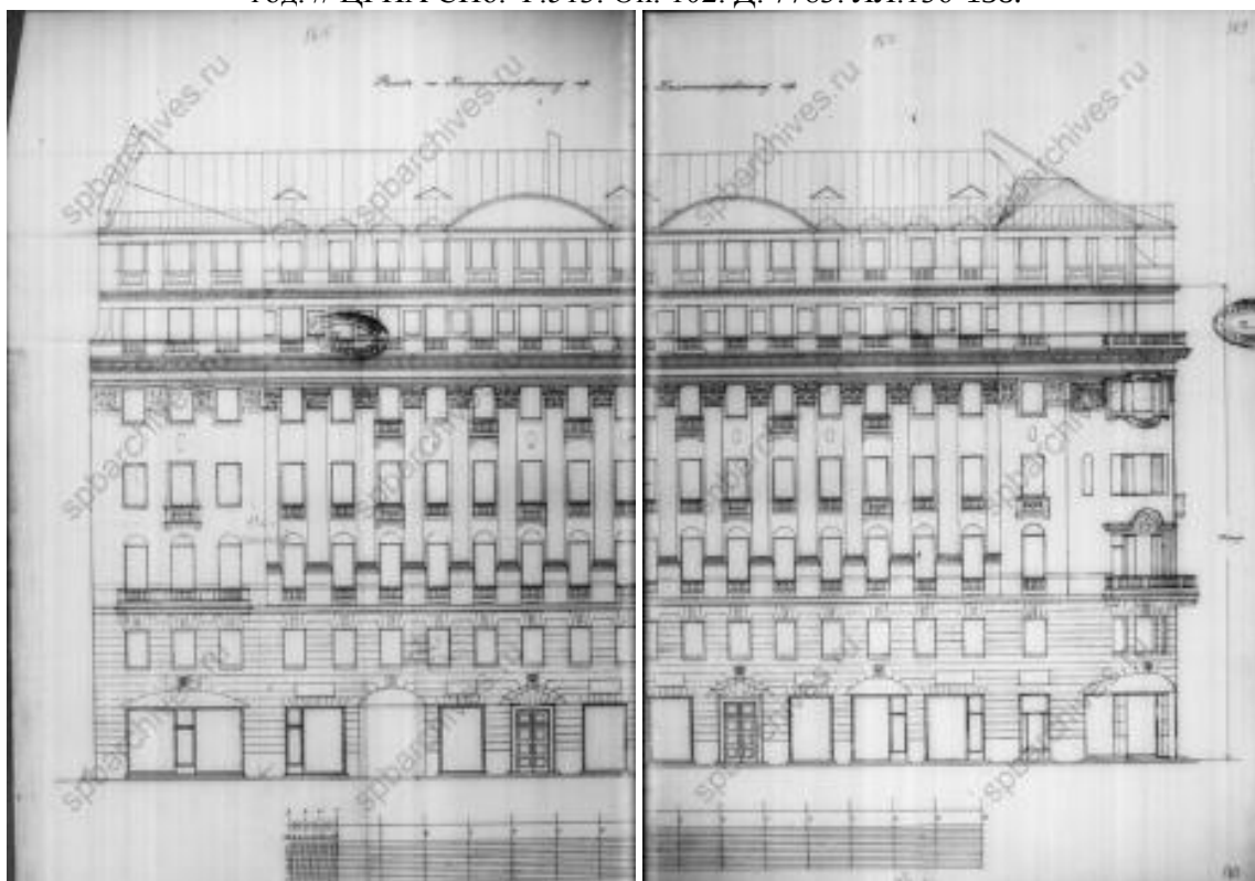
13. Проект постройки 6-этажного дома. Фасад по Каменноостровскому проспекту. Арх. А.П. Вайтенс. 1914 год. // ЦГИА СПб. Ф.513. Оп. 102. Д. 7783. ЛЛ. 165-170.
