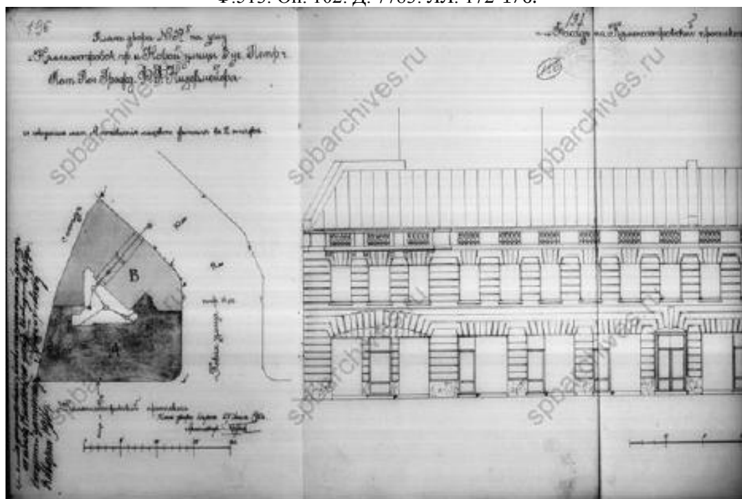
15. Проект постройки 2-этажного корпуса по Каменноостровскому проспекту. (изменение проекта 1914 года). Арх. А.П. Вайтенс. План. Северный фасад. 1916 год. // ЦГИА СПб. Ф. 513. Оп. 102. Д.7783. ЛЛ. 196-198.
