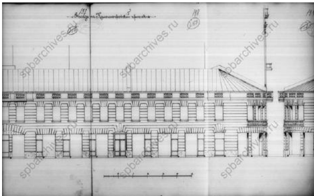
16. Проект постройки 2-этажного корпуса по Каменноостровскому проспекту. (изменение проекта 1914 года). Арх. А.П. Вайтенс. План. Северный фасад. 1916 год. // ЦГИА СПб. Ф. 513. Оп. 102. Д.7783. ЛЛ. 197-199.
