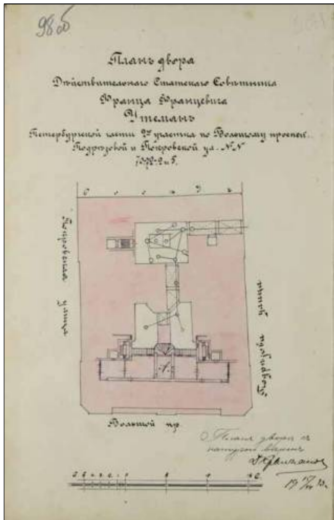
32. Утверждение проекта. План двора. Ф.Ф. Утемана. 1914 г. ЦГИА СПб. Фонд 513. Опись 102. Дело 7345. ЛЛ. 98-981 об.
