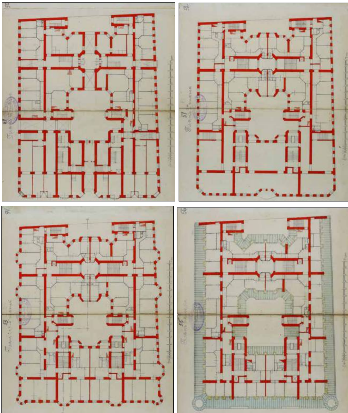
25. Поэтажные планы. 1911 г. ЦГИА СПб. Ф. 513. Оп. 102. Д. 7345. ЛЛ. 49-56.
