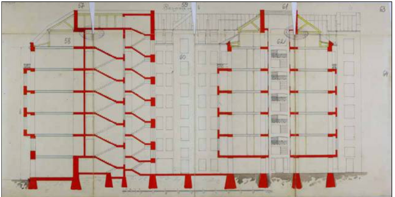
24. Разрез по ав. 1911 г. ЦГИА СПб. Ф. 513. Оп. 102. Д. 7345. ЛЛ. 57-64.
