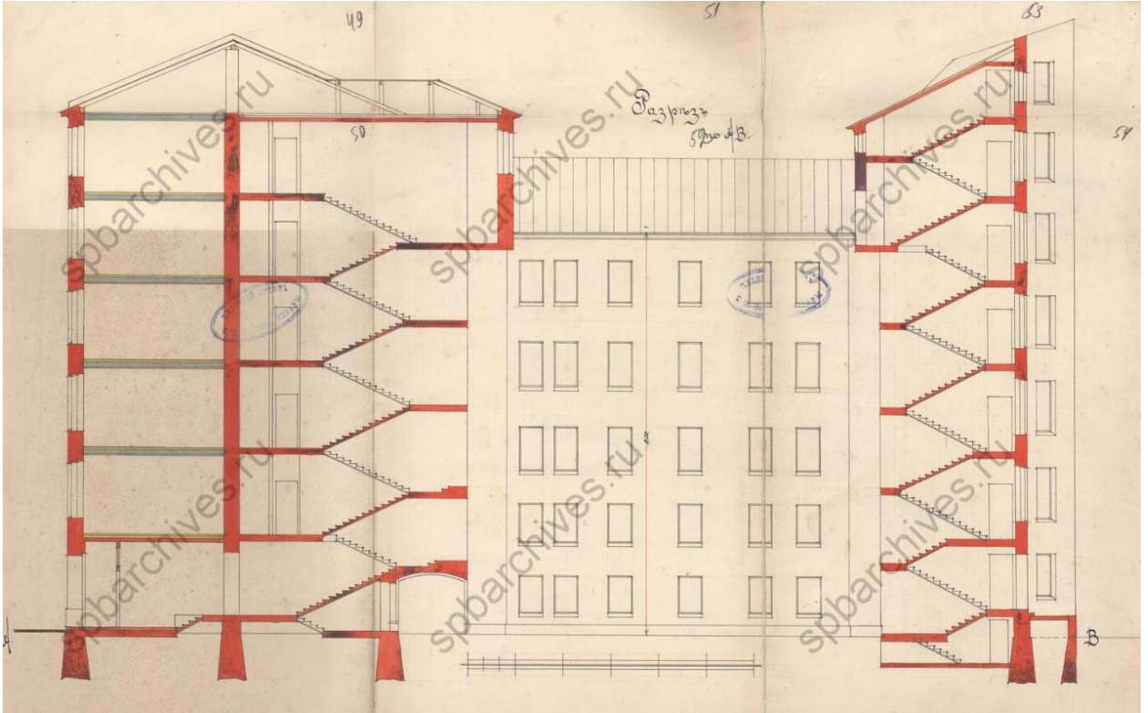
Илл. 12. Проектный разрез. 1908 г. (источник: ЦГИА СПб. Ф. 513. Оп. 102. Д. 9137).
