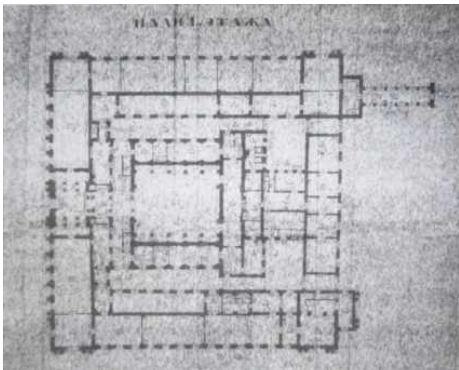
51. Корпус Бенуа. Инвентаризационный план 1 этажа. Фотокопия. 1974 г. Сектор хранения документированной информации (архив) КГИОП (П-166-6. № 187 п).
