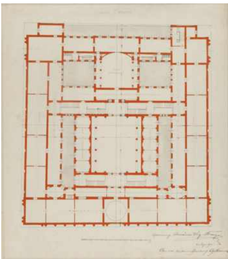
32. Проект выставочного корпуса Императорской Академии художеств. План 2 этажа. Архитектор Л. Бенуа. 1914 г. Государственной Русский музей (инв. № Аф ВХ 477).
