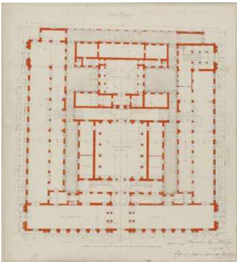
31. Проект выставочного корпуса Императорской Академии художеств. План 1 этажа. Архитектор Л. Бенуа. 1914 г. Государственной Русский музей (инв. № Аф ВХ 476).
