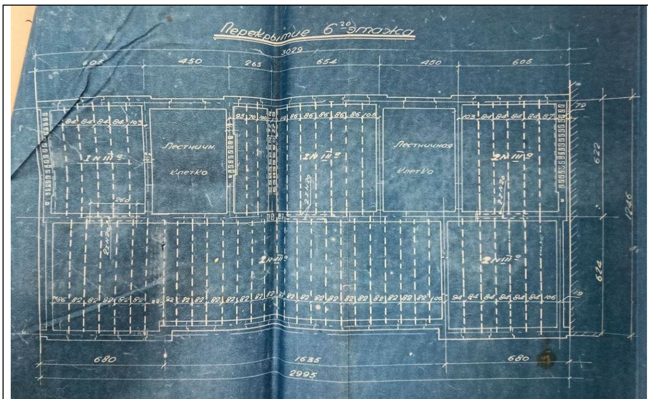
1934 г. Первоначальный проект. План перекрытия 6-го этажа. Архитектор И.С.Шапиро. ЦГАЛИ. Ф. Р-257. Оп.11. Д. 87.Л.34.
