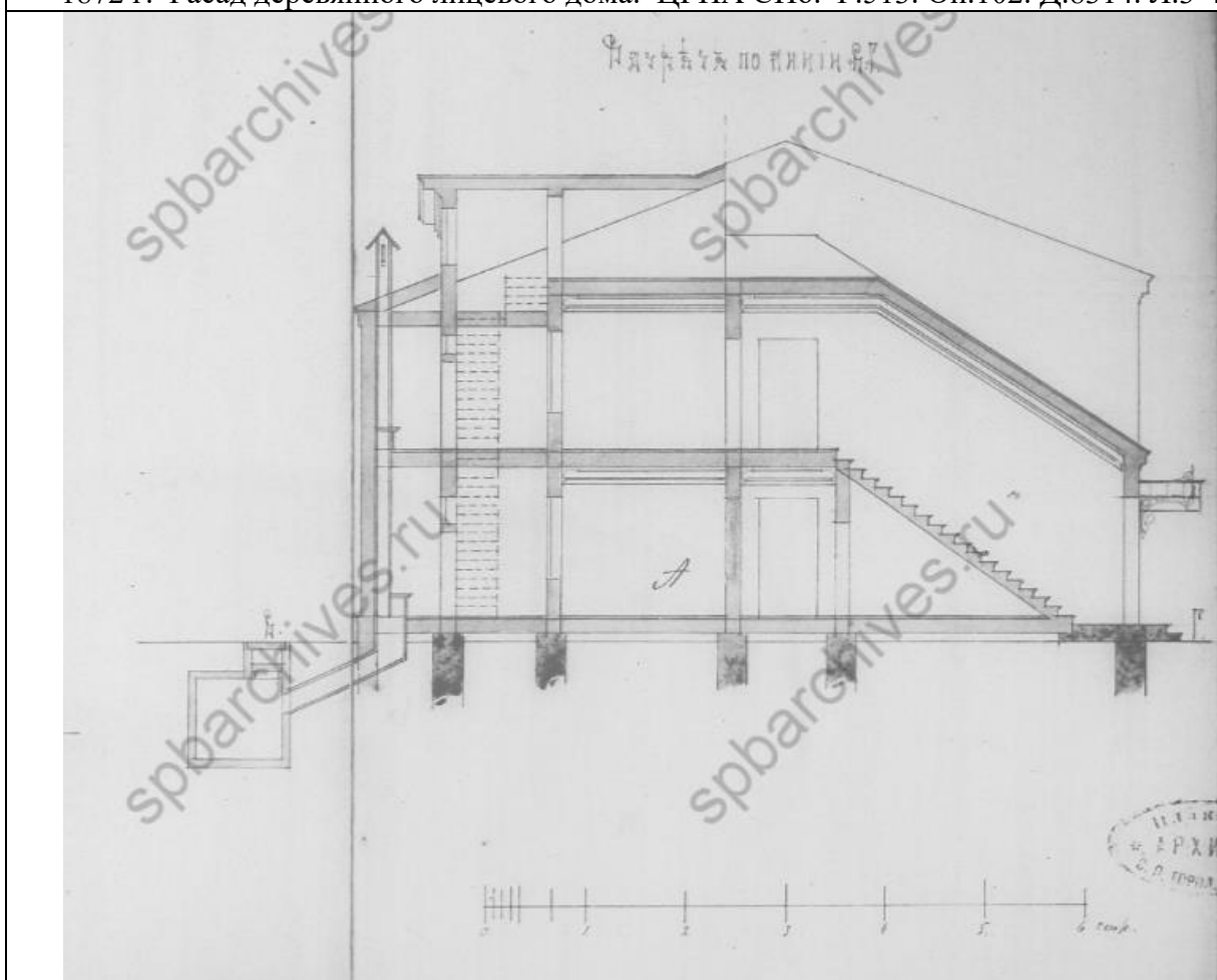
1872 г. Разрез деревянного лицевого дома. ЦГИА СПб. Ф.513. Оп.102. Д.8314. Л.5.
