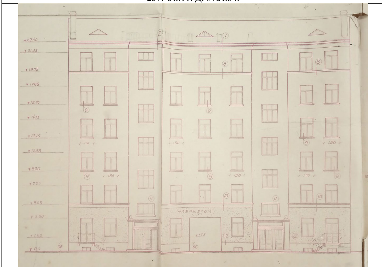
1934 г. Первоначальный проект. Дворовый фасад. Архитектор И.С.Шапиро. ЦГАЛИ. Ф. Р-257. Оп.11. Д. 87.Л.34.
