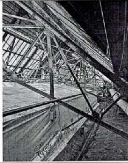
Фото 13. Фрагмент конструкций светового фонаря
