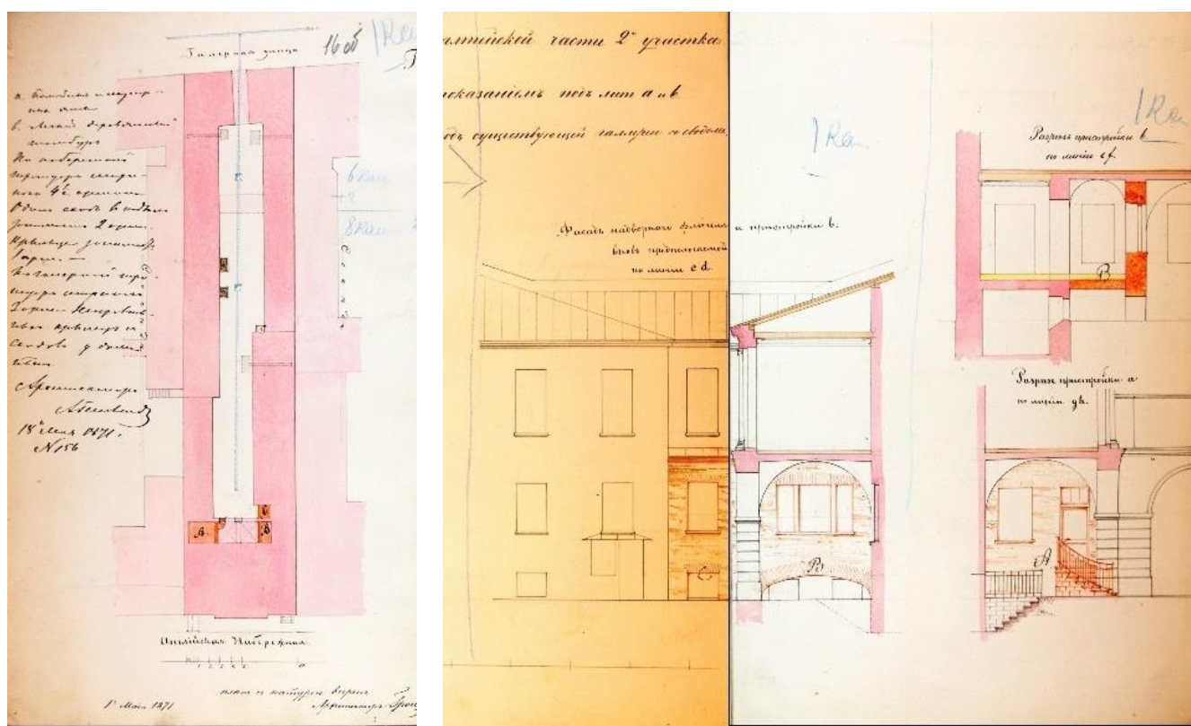
Илл.14-1. План двора и надворный фасад «набережного Дома» с показанием предполагаемых перестроек (галерея корпуса по Английской набережной). 1871 г. ЦГИА СПб. Ф. 513. Оп. 102. Д. 75. Лл. 16 об-19. Фрагменты.
