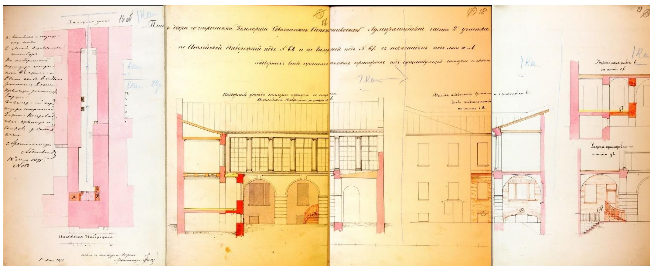
Илл.14. План двора и надворный фасад «набережного Дома» с показанием предполагаемых перестроек (галерея корпуса по Английской набережной). 1871 г. ЦГИА СПб. Ф. 513. Оп. 102. Д. 75. Лл. 16 об-19.
