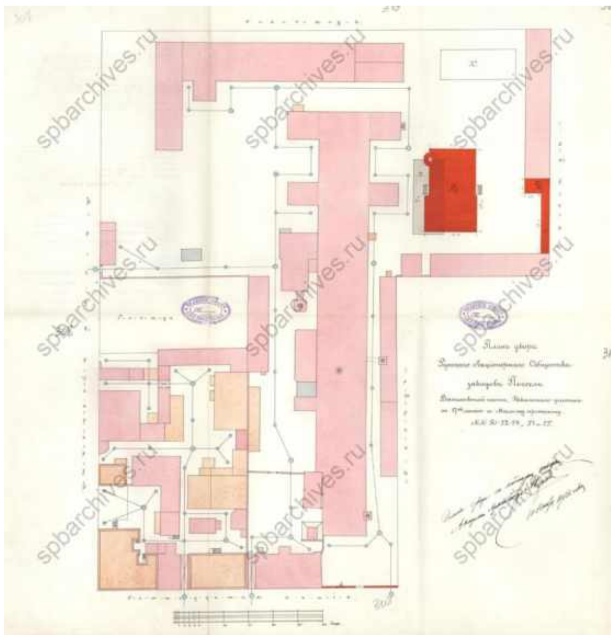
Илл. 42. План двора Русского акционерного общества заводов Посель. 1912 г. (источник: ЦГИА СПб. Ф. 513. Оп. 102. Д. 2003).
