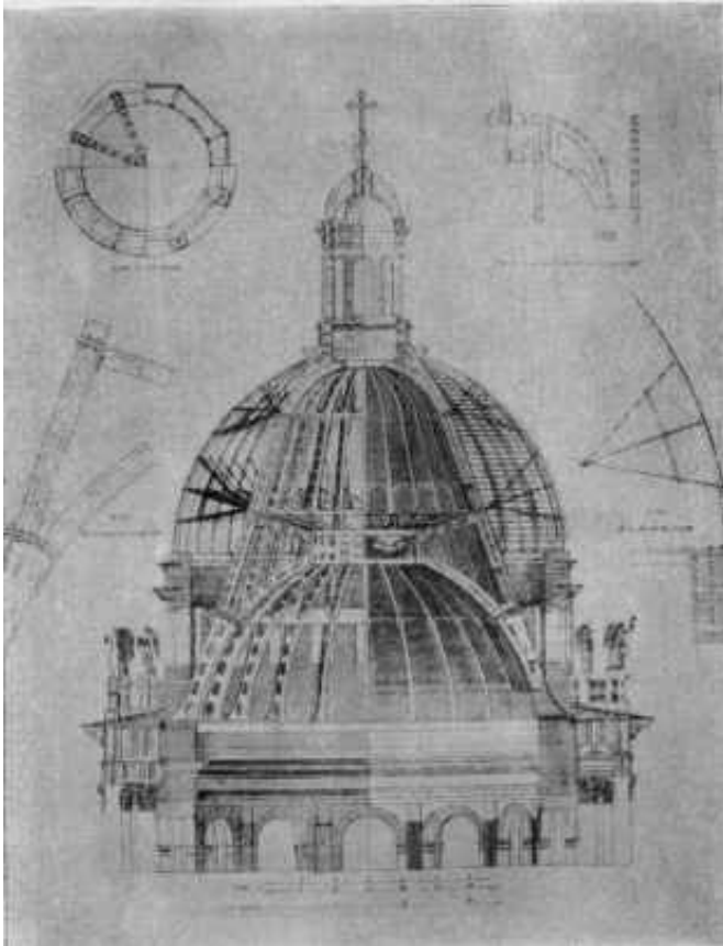
13. Разрез конструкции купола Исаакиевского собора. Гравюра Нормана старшего по рисунку О. Монферрана, 1845 г. Источник - https://online-karta.ru/schemes/shema-isaakievskogo-sobora?utm_medium=organic&utm_source=yasmartcamera
