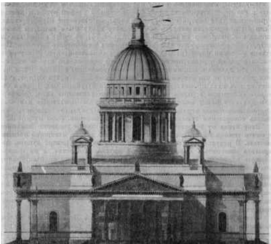
11. Продольный фасад Исаакиевского собора, окончательно утвержденный 14 февраля 1835 г. Источник - https://online-karta.ru/schemes/shema-isaakievskogo-sobora?utm_medium=organic&utm_source=yasmartcamera
