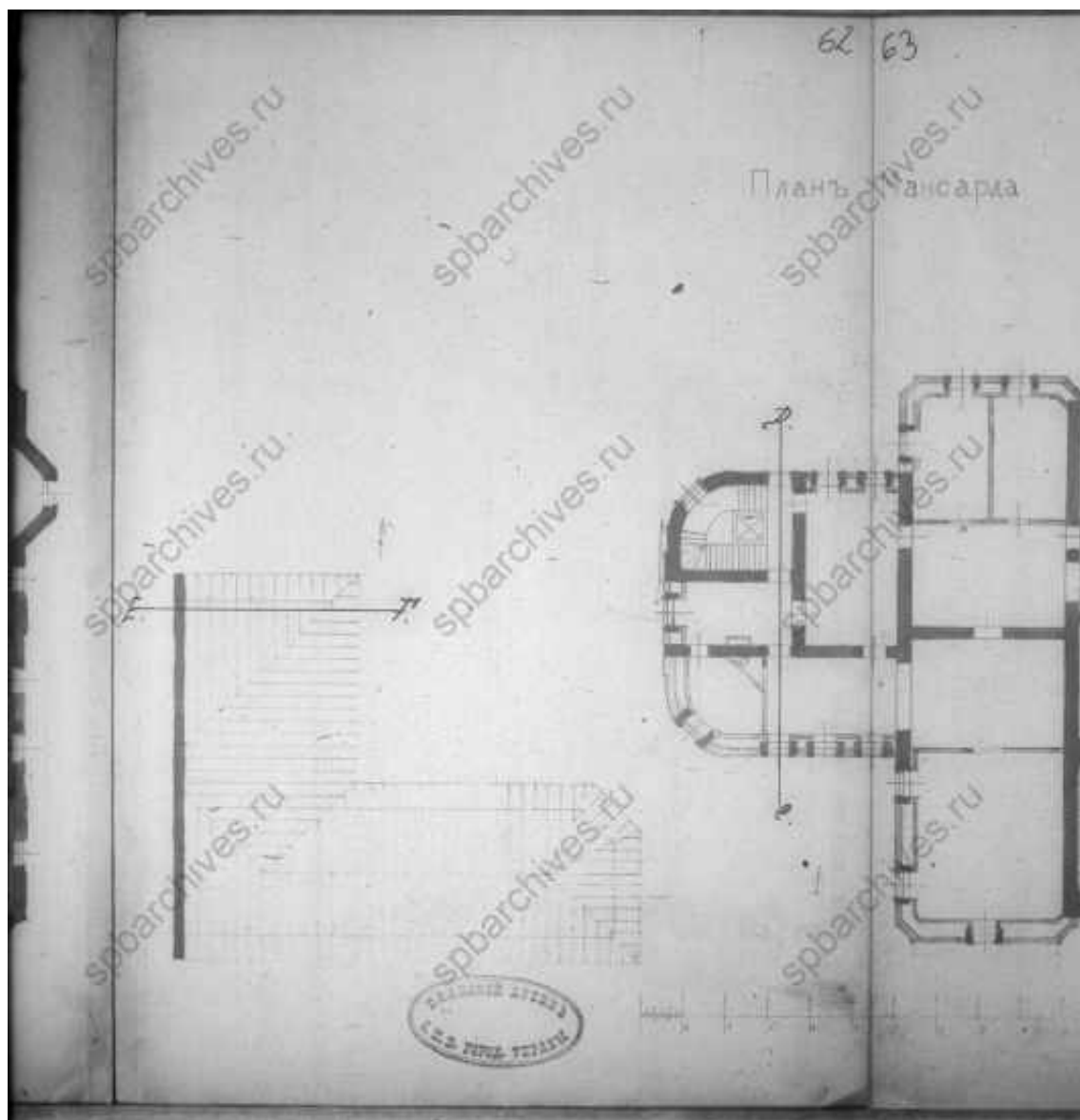
8. Чертежи дома на участке, принадлежавшем Шорохову, А.Н.Колупаевой, Клементьевой, Ф.Ф.Отто, А.К.Отто, В.А.Слепцову, А.С.Слепцовой, кн. К.А.Горчакову по Малой Монетной ул., 10, 12, 14 и Большой Монетной ул., 11. 1832–1908 гг. ЦГИА СПб ф.513 оп.102 д.8141. Л. 62
