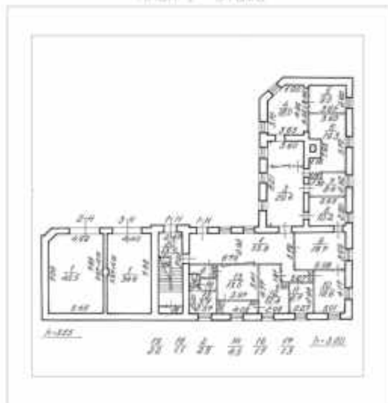
План 1 этажа
