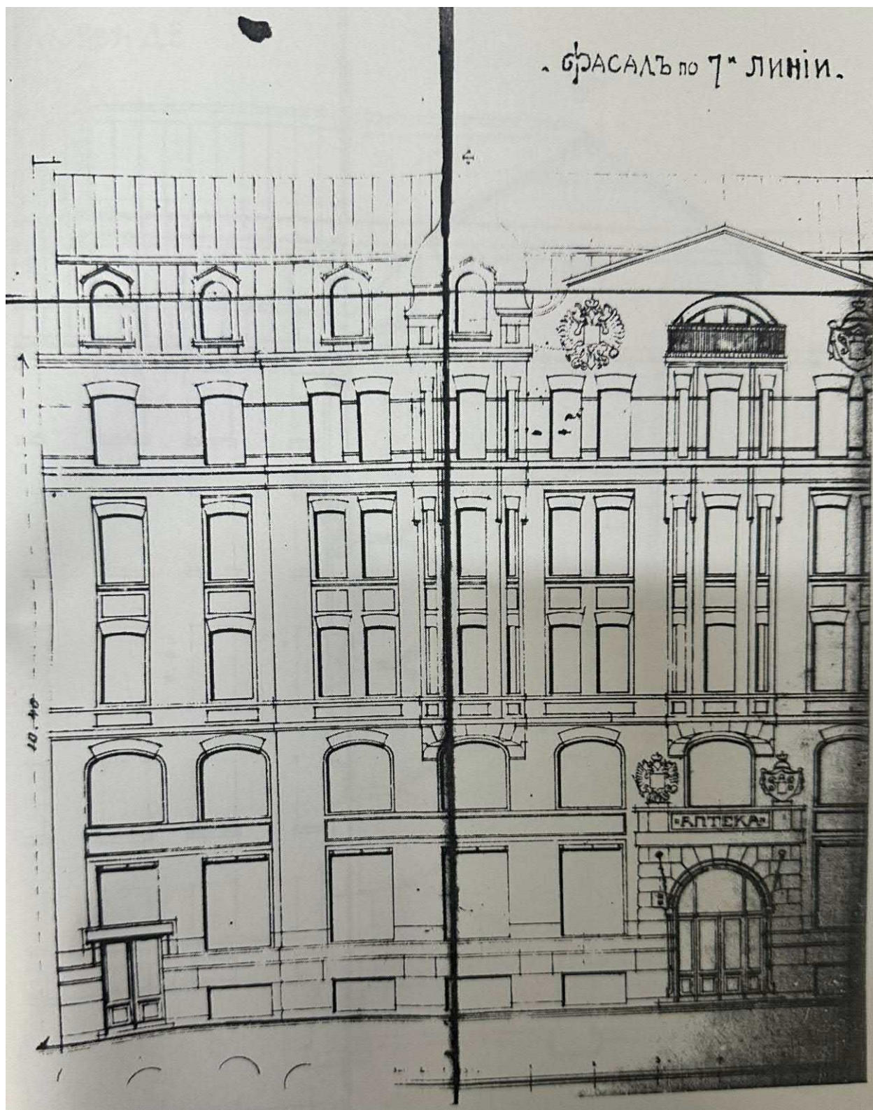
Илл. 7. Дом А.В.Пеля. Фасад здания. Архитектор З.Я.Леви, 1908г. ЦГИА СПб. Ф.513, оп.102, д..1630, л.155-156
