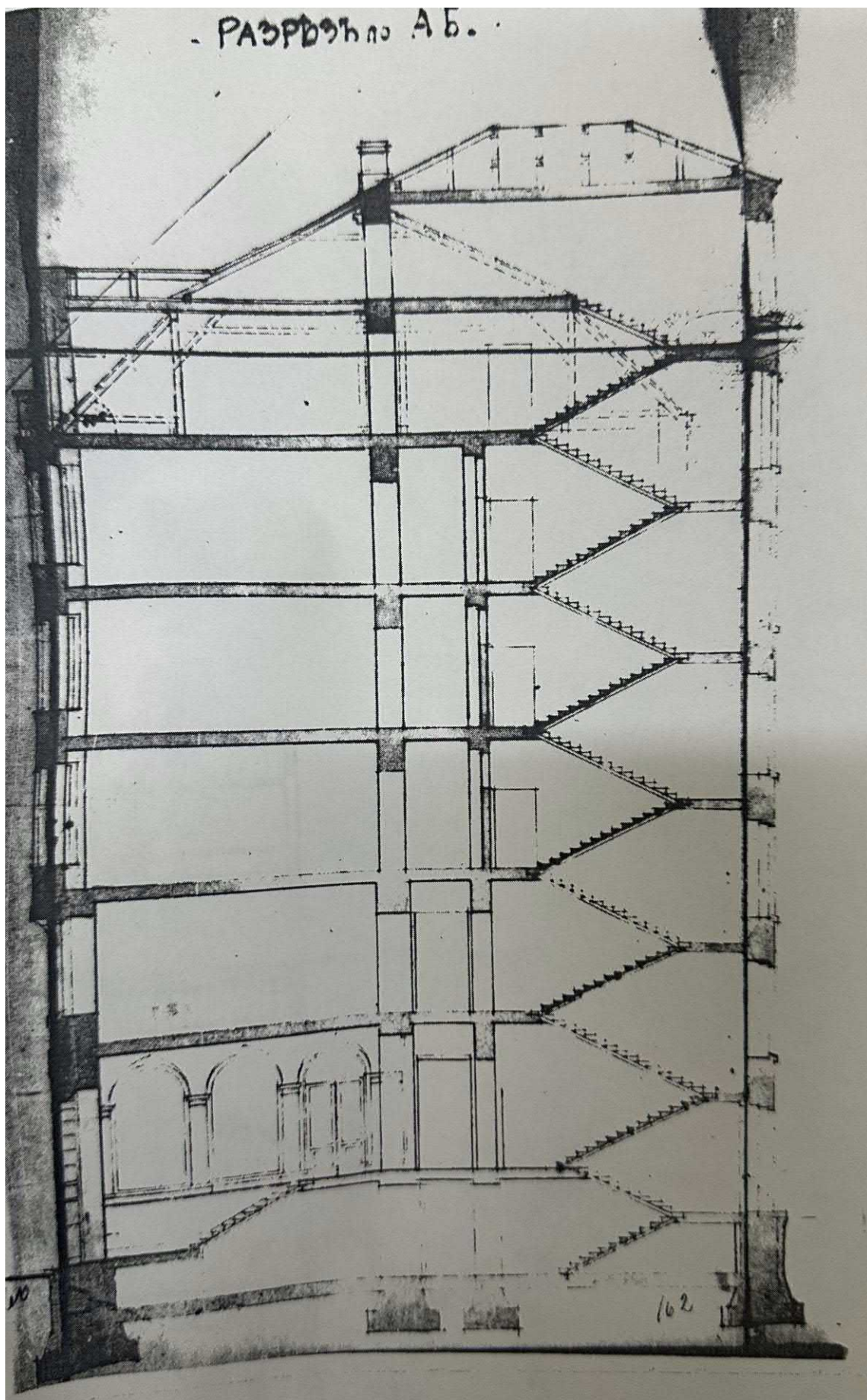
Илл. 9. Дом А.В.Пеля. Разрез здания. Архитектор З.Я.Леви, 1908г. ЦГИА СПб. Ф.513, оп.102, д.1630, л.163
