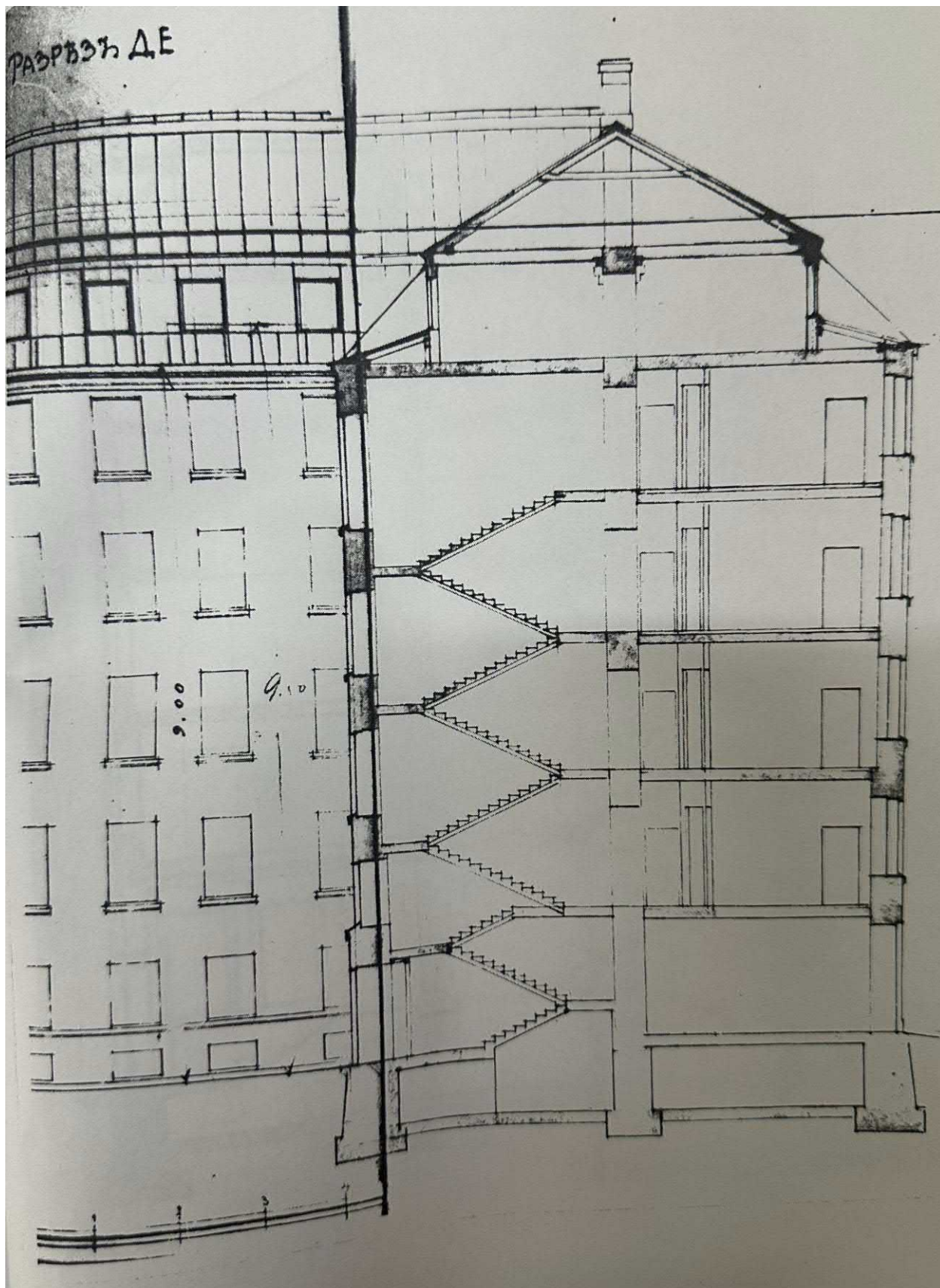
Илл. 8. Дом А.В.Пеля. Разрез здания. Архитектор З.Я.Леви, 1908г. ЦГИА СПб. Ф.513, оп.102, д.1630, л.161
