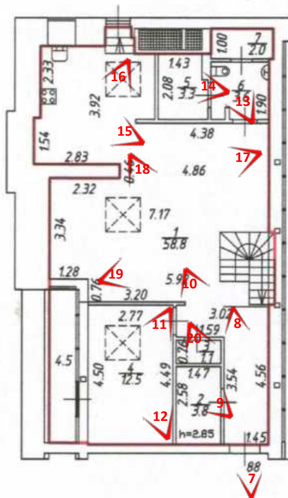
Рисунок 2. Схема фотофиксации на фрагменте плана 4 этажа
