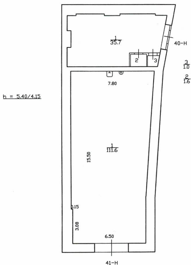
План 1 этажа
