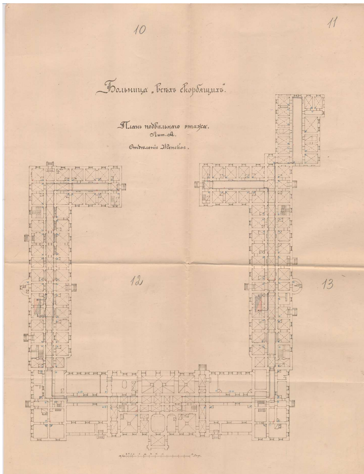
9. Больница всех скорбящих. План подвального этажа. Женское отделение. После 1887. ЦГИА СПб. Фонд 1357. Опись 10. Дело 173. Листы 10-13.
