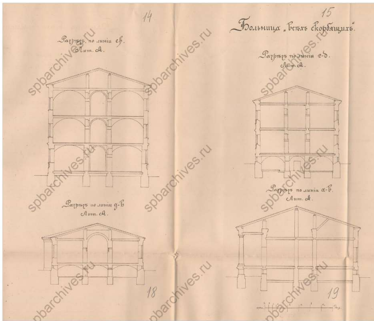
13. Больница всех скорбящих. Разрезы. После 1887. ЦГИА СПб. Фонд 1357. Опись 10. Дело 173. Листы 14-19.
