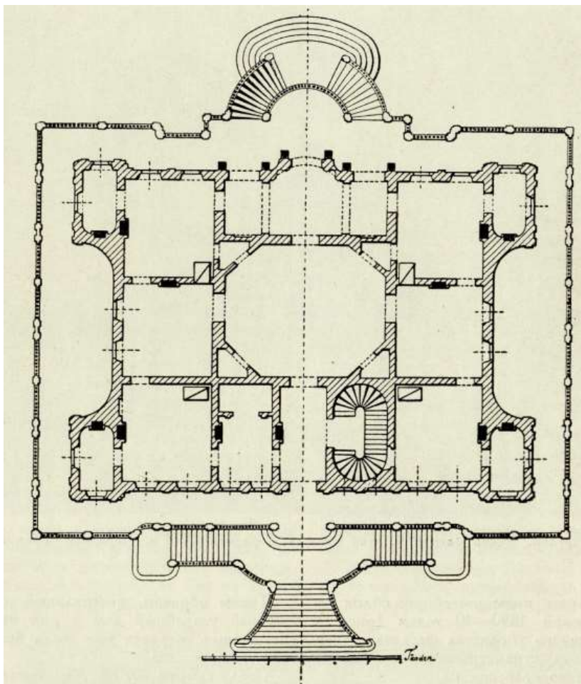
2. В. В. Растрелли. Первый вариант плана дачи Сиверса. Середина XVIII в. Народная библиотека в Варшаве. Приводится по: Денисов Ю. Усадьба XVIII века на Петергофской дороге// Архитектурное наследство. 1953. №4. С. 150.
