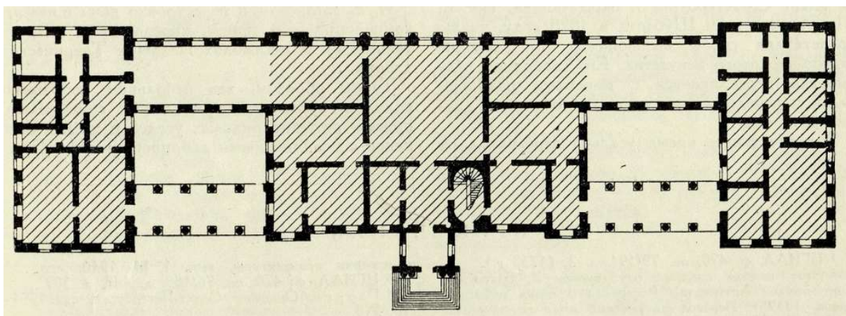
3. План первого этажа после перестройки в 1780-х гг. Реконструкция. Денисов Ю. Усадьба XVIII века на Петергофской дороге// Архитектурное наследство. 1953. №4. С. 154.
