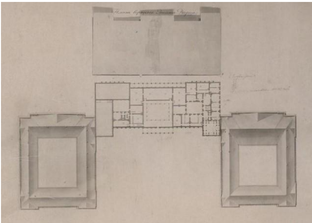
12. К. Росси. Михайловский дворец. План верхнего этажа. 1820-е гг. Фотокопия с чертежа. НИМ РАХ (инв. № Ф-4037)
