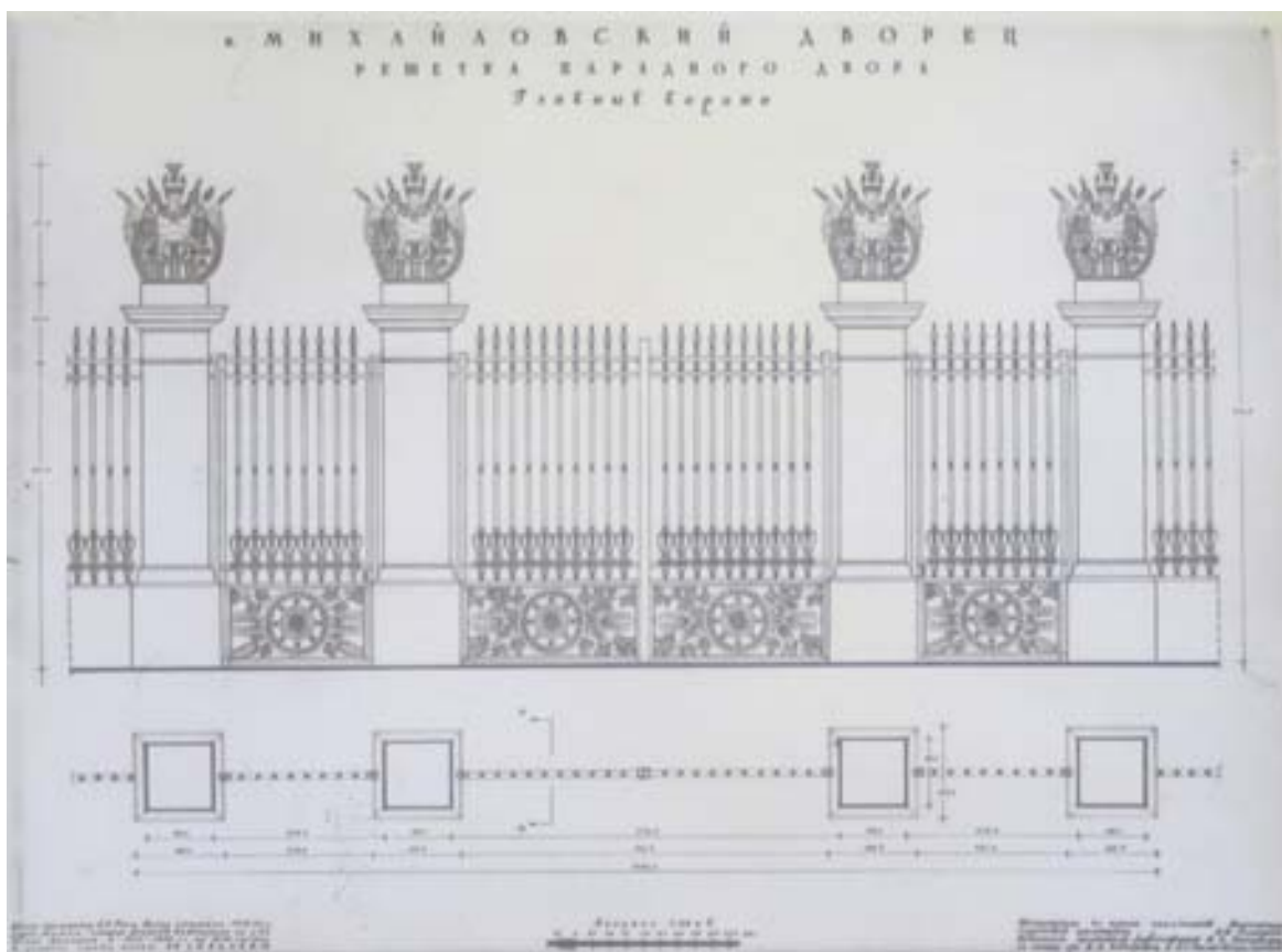
51. Государственный Русский музей. Михайловский дворец. Ворота ограды парадного двора. Обмерный чертеж. Фотокопия. 1956 г. Сектор хранения документированной информации (архив) КГИОП (П-166-1. № 183 п)
