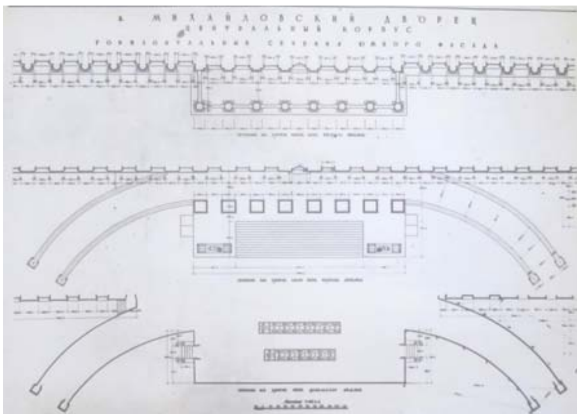
47. Государственный Русский музей. Михайловский дворец. Центральный портик с пандусом. План. Обмерный чертеж. Фотокопия. 1956 г. Сектор хранения документированной информации (архив) КГИОП (П-166-1. № 183 п)
