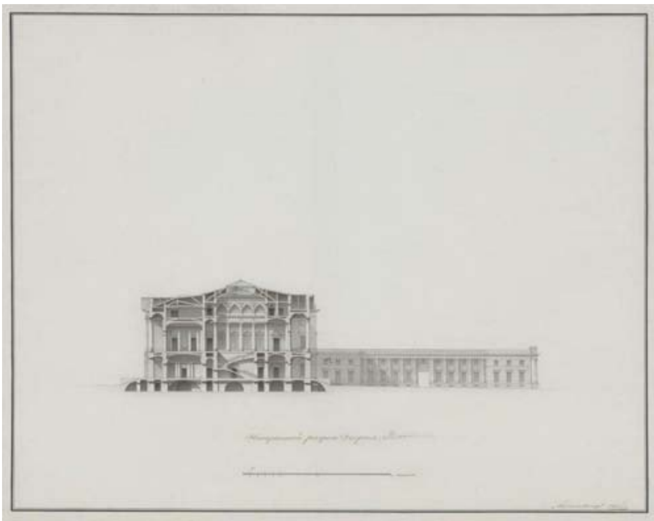
8. К. Росси. Михайловский дворец. Поперечный разрез по главному корпусу и фасада восточного флигеля. Бумага, тушь, отмывка. 1819 г. НИМ РАХ (инв. № А-261)
