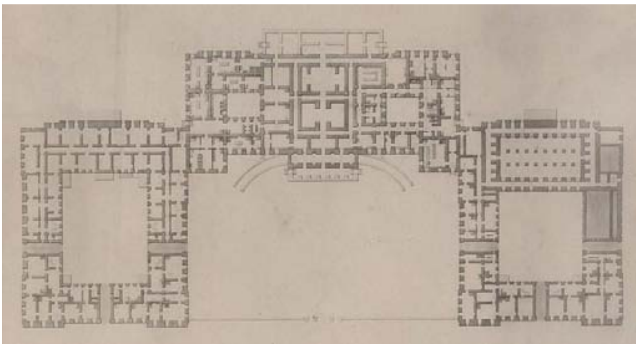
9. К. Росси. Михайловский дворец. План подвального этажа. 1820-е гг. Фотокопия с чертежа. НИМ РАХ (инв. № Ф-4034)
