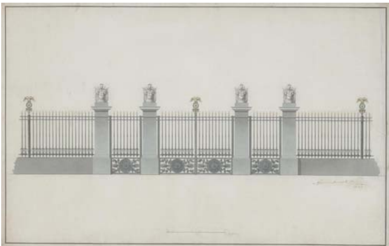
13. К. Росси. Проект ограды с воротами. Вариант с арматурой. Акварель. 1823 г. НИМ РАХ (инв. № А-274)
