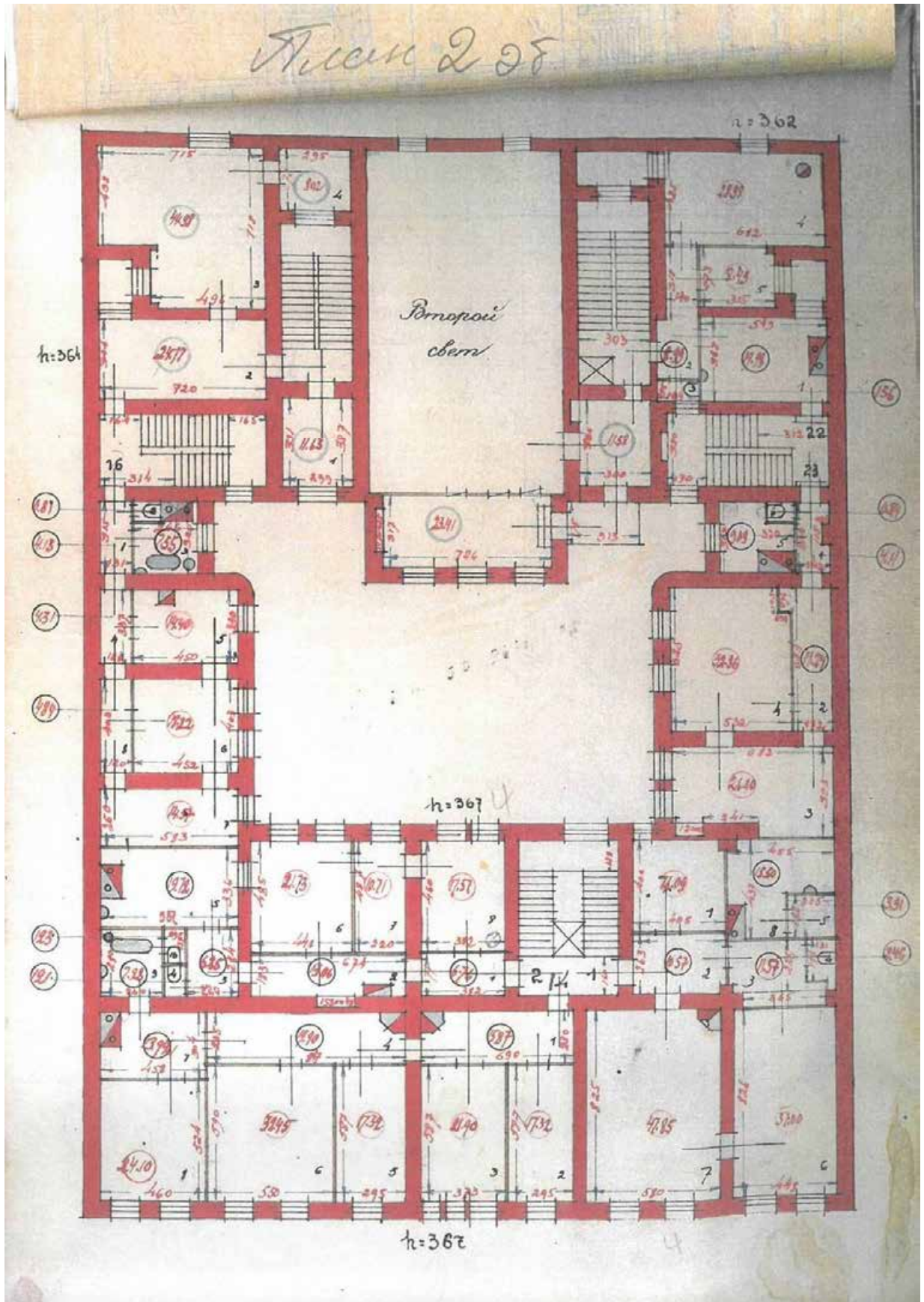
Илл.35. План 2-го этажа. 1931 г. ГУП ГУИОН ПИБ Центрального района.
