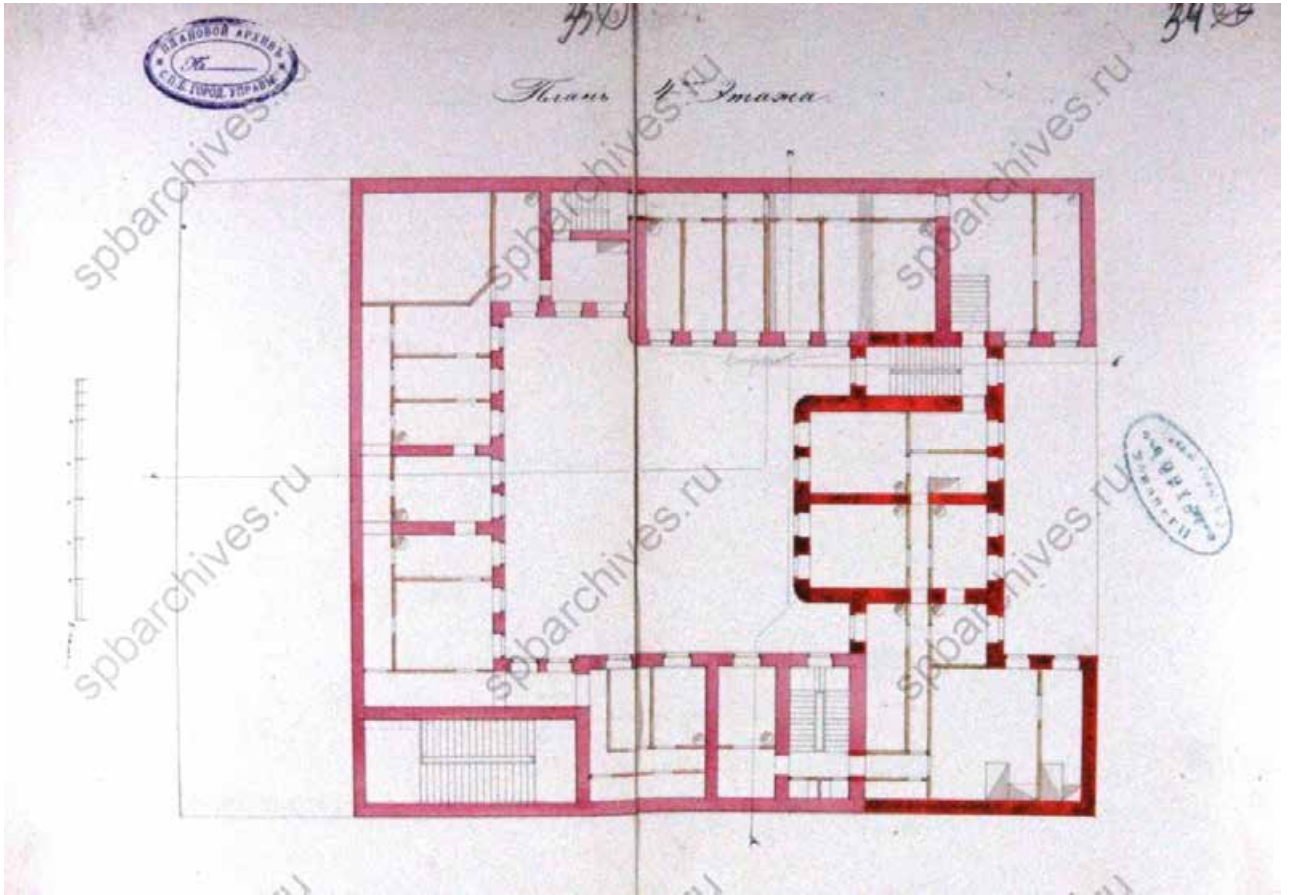
Илл.14. План 4-го этажа. 1880 г. ЦГИА СПб. Фонд 513. Описание 102. Дело 4318. Л. 33-34.
