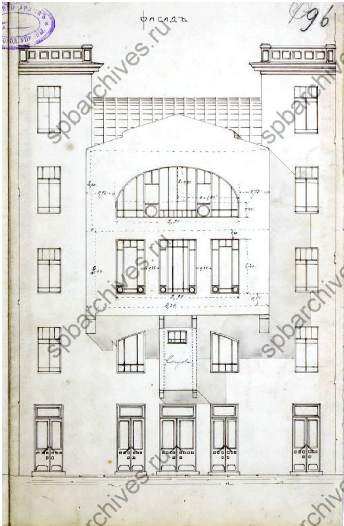
Илл.30. Фасад. 1911 г. ЦГИА СПб. Фонд 513. Описание 102. Дело 4318. Л. 96.
