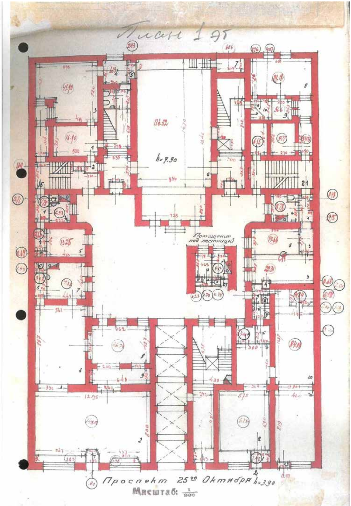
Илл.34. План 1-го этажа. 1931 г. ГУП ГУИОН ПИБ Центрального района.
