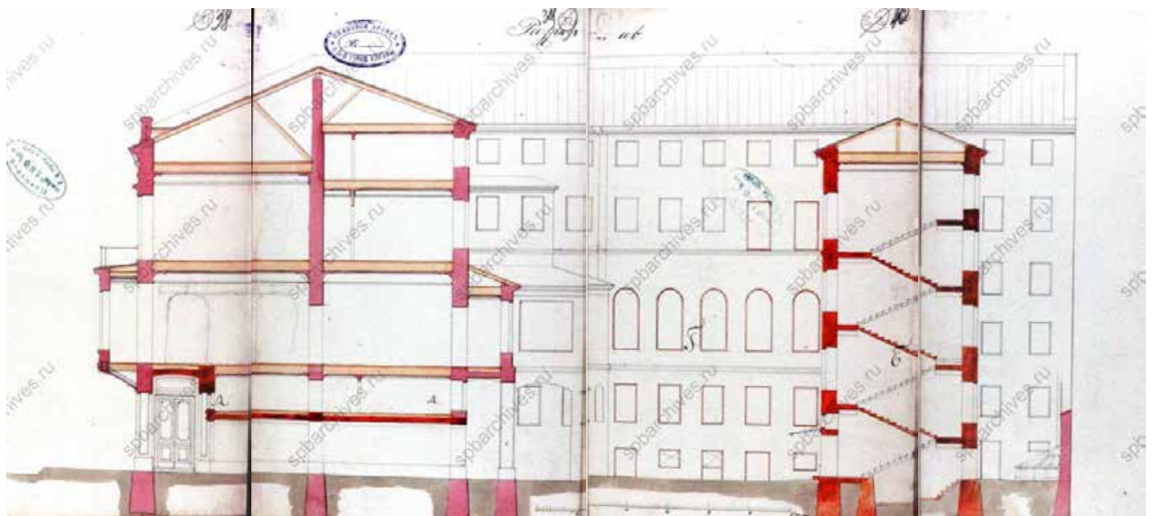
Илл.15. Разрез а-в. 1880 г. ЦГИА СПб. Фонд 513. Описание 102. Дело 4318. Л. 38-41.
