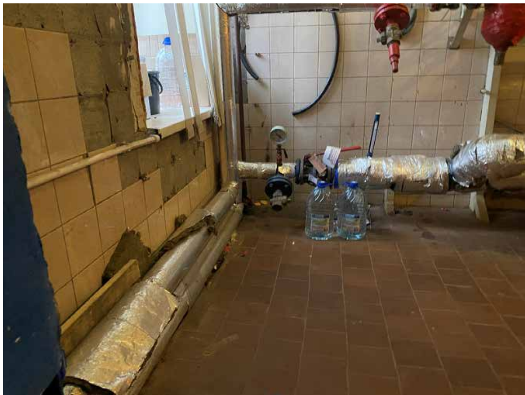
Фото 13, 1 этаж. Общий вид ИТП узла холодного водоснабжения
